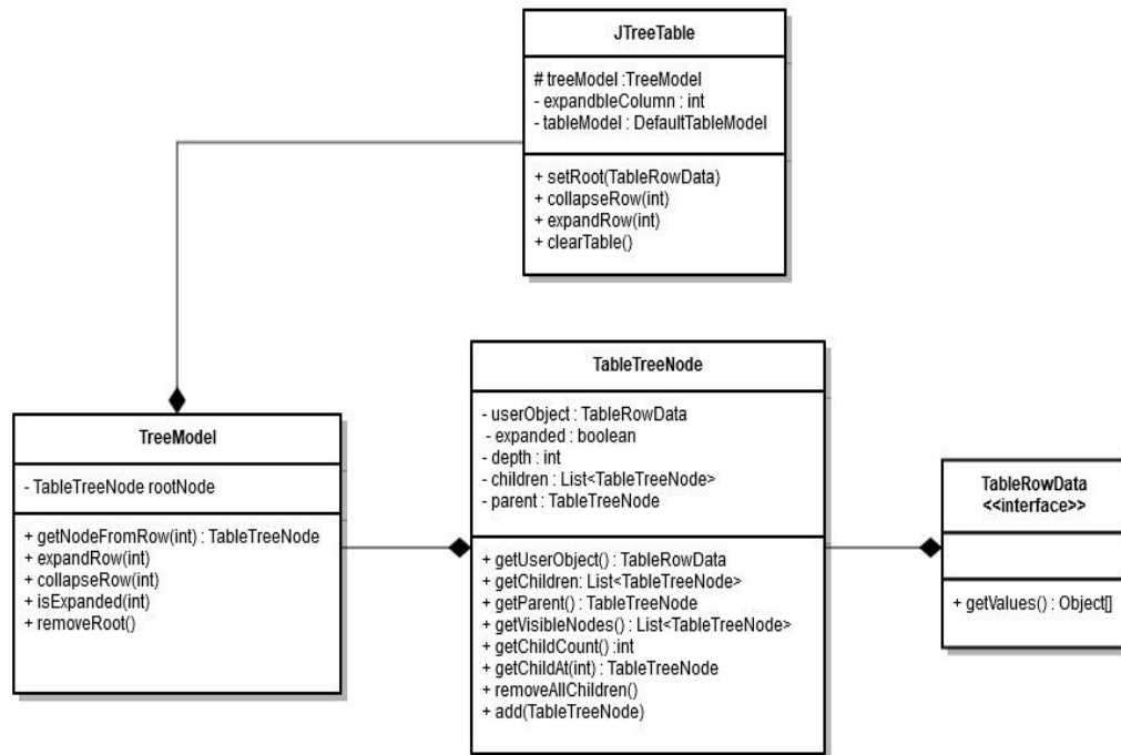
Figura 2.5: Diagrama UML del paquete com.general.view.jtreetable
