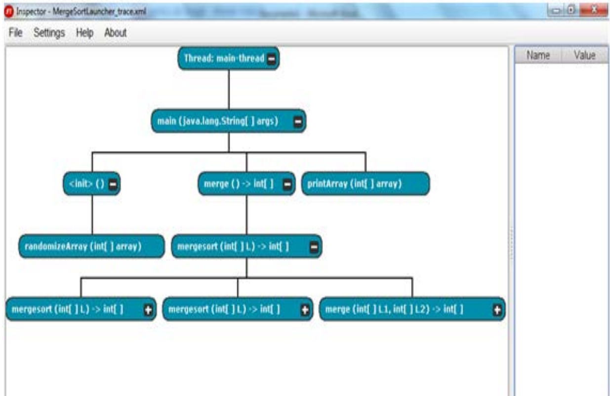
Figura 3.7: Pantalla Inspector I
