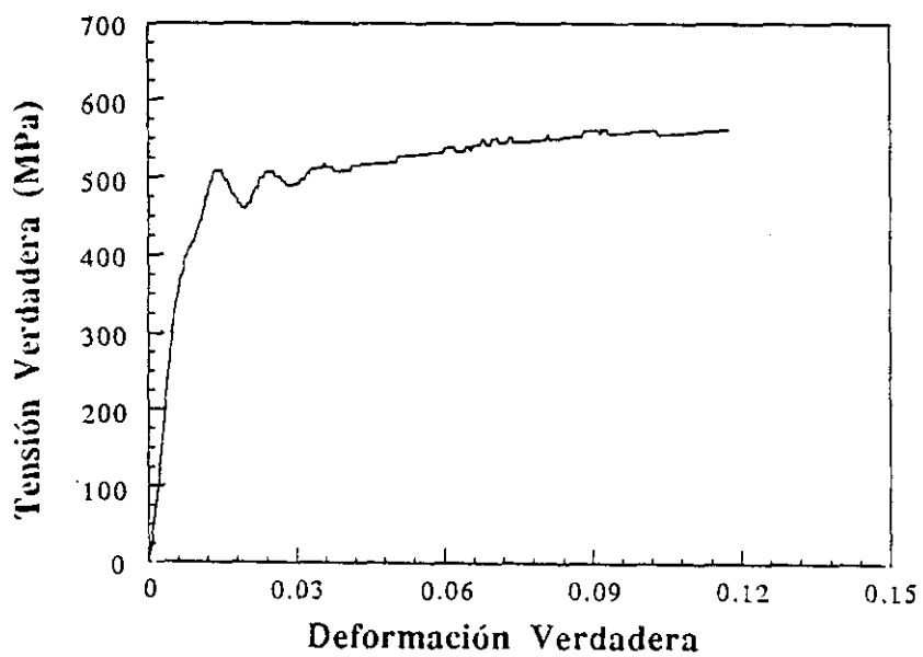
Figura 3.19 Curva Tensión verdadera-Deformación verdadera ( 1000\text{ s}^{-1} ).
