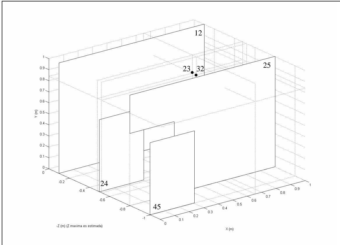
Figura 7-2-9: SECCIÓN DE ÍNDICES correspondiente al modelo tridimensional realista. Junto a cada reflector se muestra el índice asociado.
