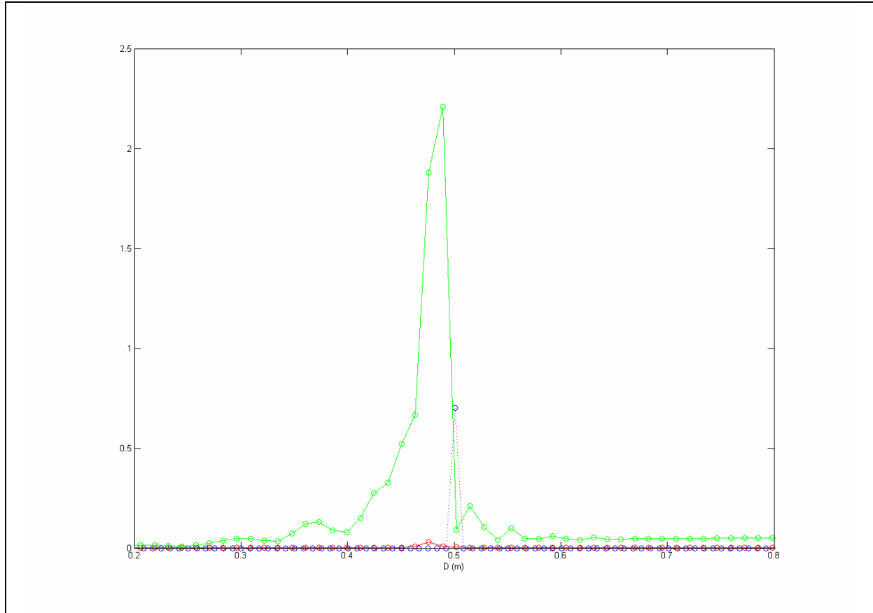
Figura 7-4-2: Trazas representativas de la DISTRIBUCIÓN MEDIDA, DISTRIBUCIÓN ESPERADA y DISTRIBUCIÓN DE REFLECTIVIDAD correspondientes al modelo tridimensional constituido por un único difractor puntual.
