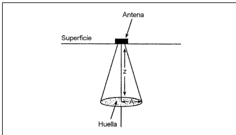
Figura 2-3-8: Cono de radiación de un geo-radar (Conyers y Goodman, 1997), donde A representa el semieje mayor de la huella elíptica y z , la profundidad desde la superficie.
