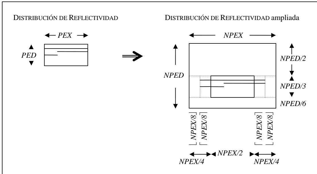
Figura 6-1-1: Ampliación de la DISTRIBUCIÓN DE REFLECTIVIDAD.
