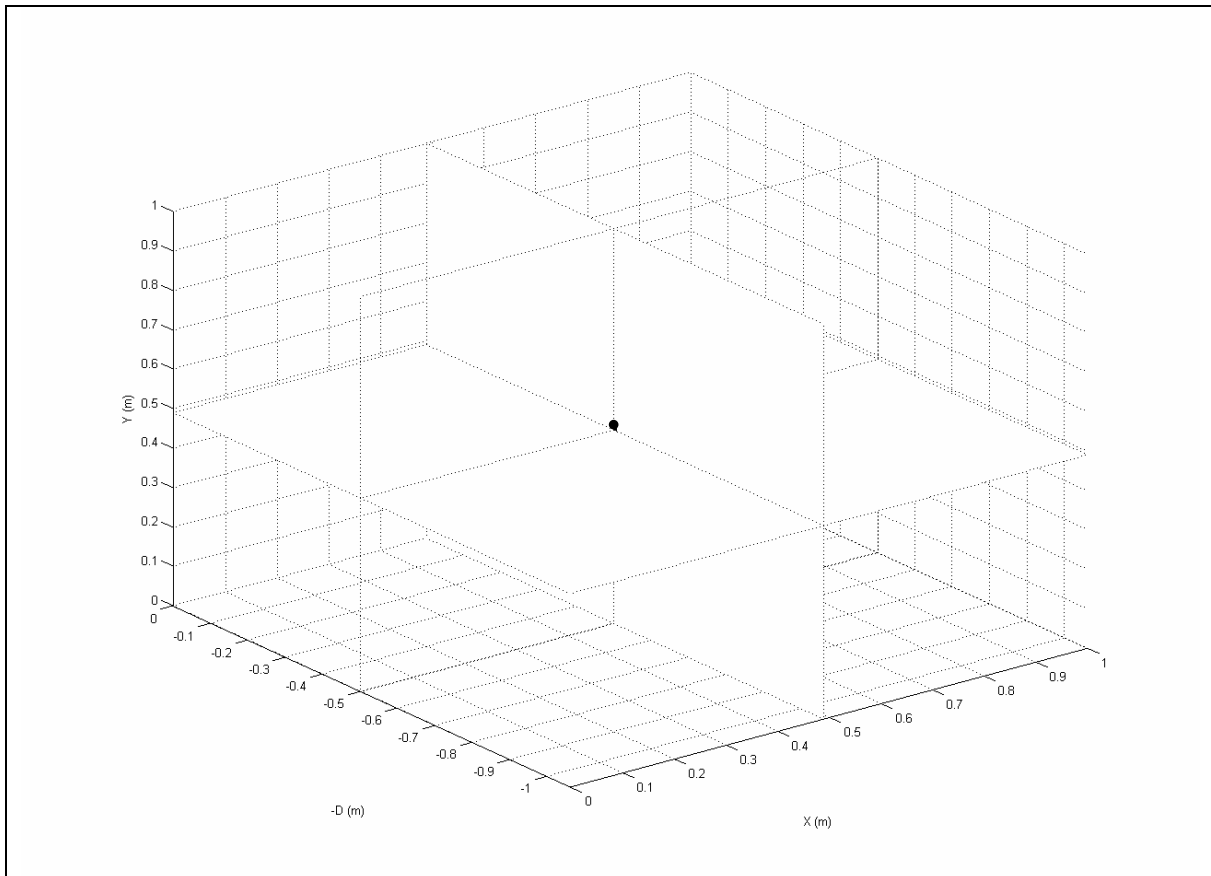
Figura 7-2-2: DISTRIBUCIÓN DE REFLECTIVIDAD correspondiente al modelo tridimensional constituido por un único difractor puntual. La reflectividad aparente del punto es r = -0,0196 + 0,6905i .
