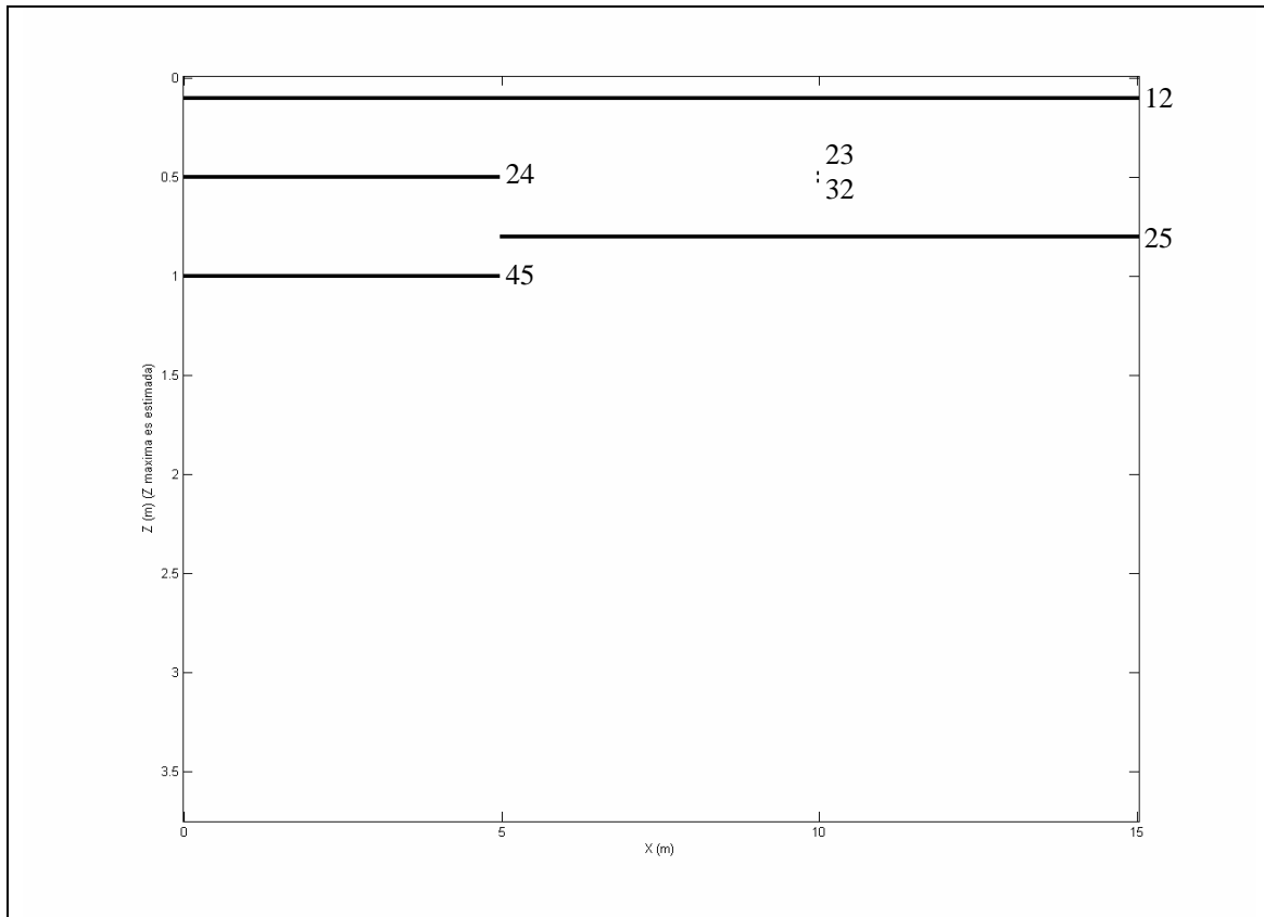
Figura 7-1-9: SECCIÓN DE ÍNDICES correspondiente al modelo bidimensional realista. Junto a cada reflector se muestra el índice asociado.
