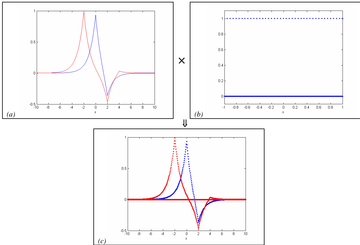
Figura 4-2-1: Muestreo de funciones, Ejemplo I:
