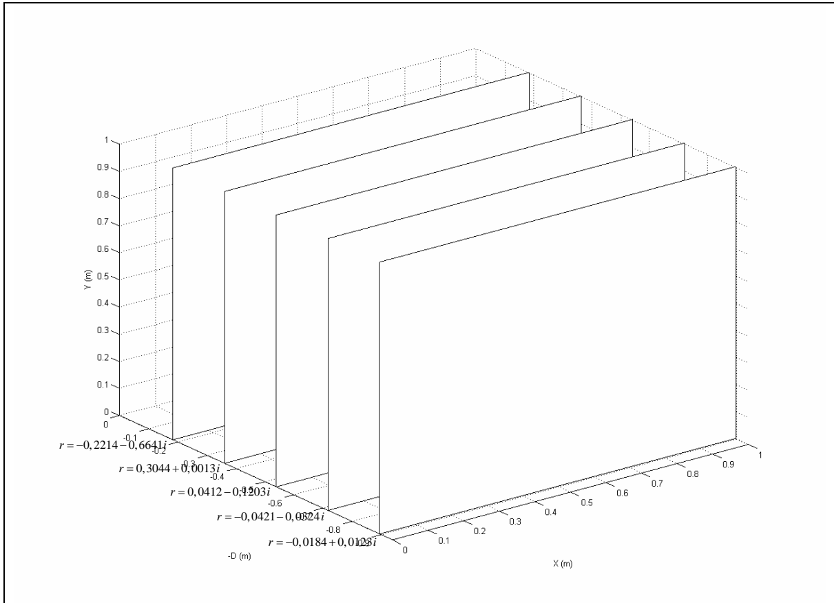
Figura 7-2-6: DISTRIBUCIÓN DE REFLECTIVIDAD correspondiente al modelo tridimensional constituido por dos capas plano-paralelas sobre un semiespacio infinito. Junto a cada reflector se muestra la reflectividad aparente.
