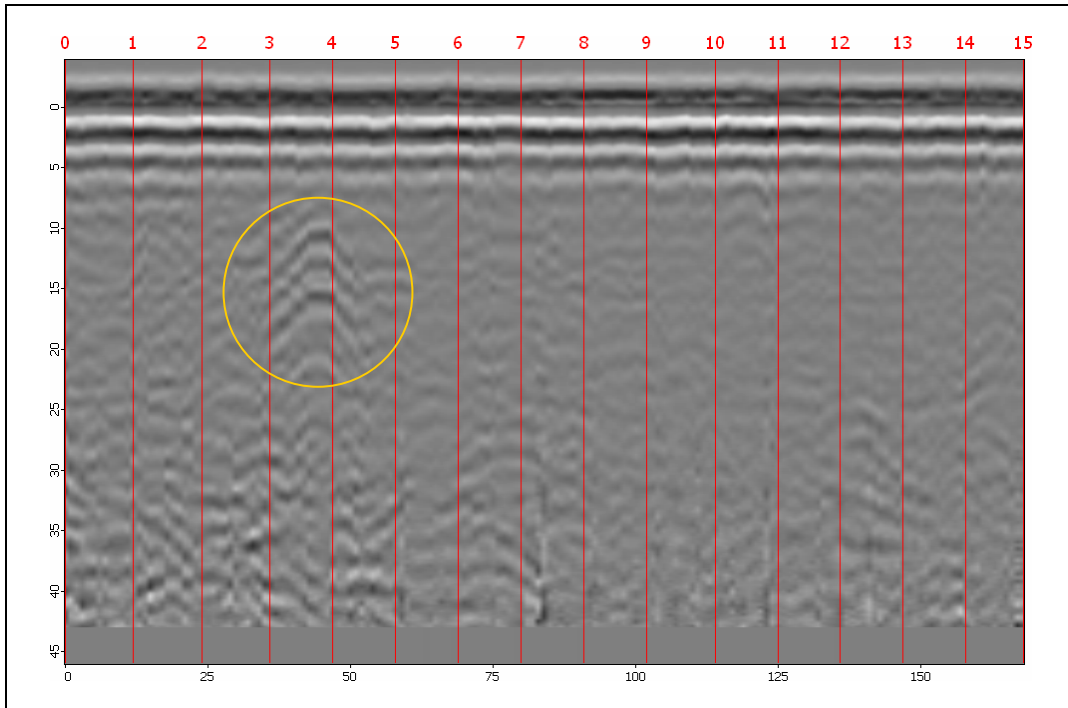
Figura 8-3-4: Mapa de color en tonos de gris del registro correspondiente a la huerta del Monasterio de El Paular tras la interpolación en el eje espacial (el blanco corresponde al valor mínimo, el negro al máximo). El eje de ordenadas expresa el tiempo doble de recorrido, en nanosegundos, y el eje de abscisas el número de traza. Las líneas verticales muestran la distancia desde el inicio del perfil, en metros. En amarillo se indica la señal a analizar.
