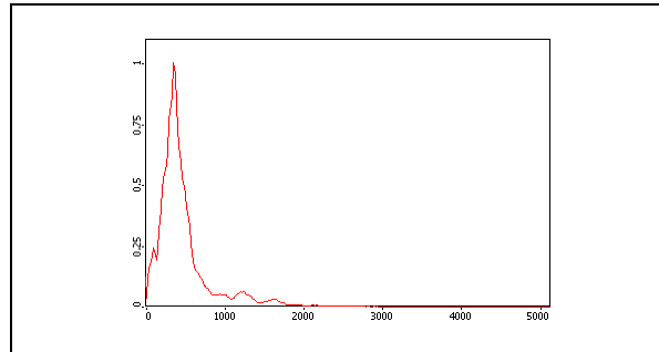
Figura 8–3-6: Espectro de potencia normalizado de la región del registro correspondiente a la huerta del Monasterio de El Paular que contiene la señal objeto de estudio, previo al filtrado temporal. El eje de abscisas expresa la frecuencia, en MHz.
