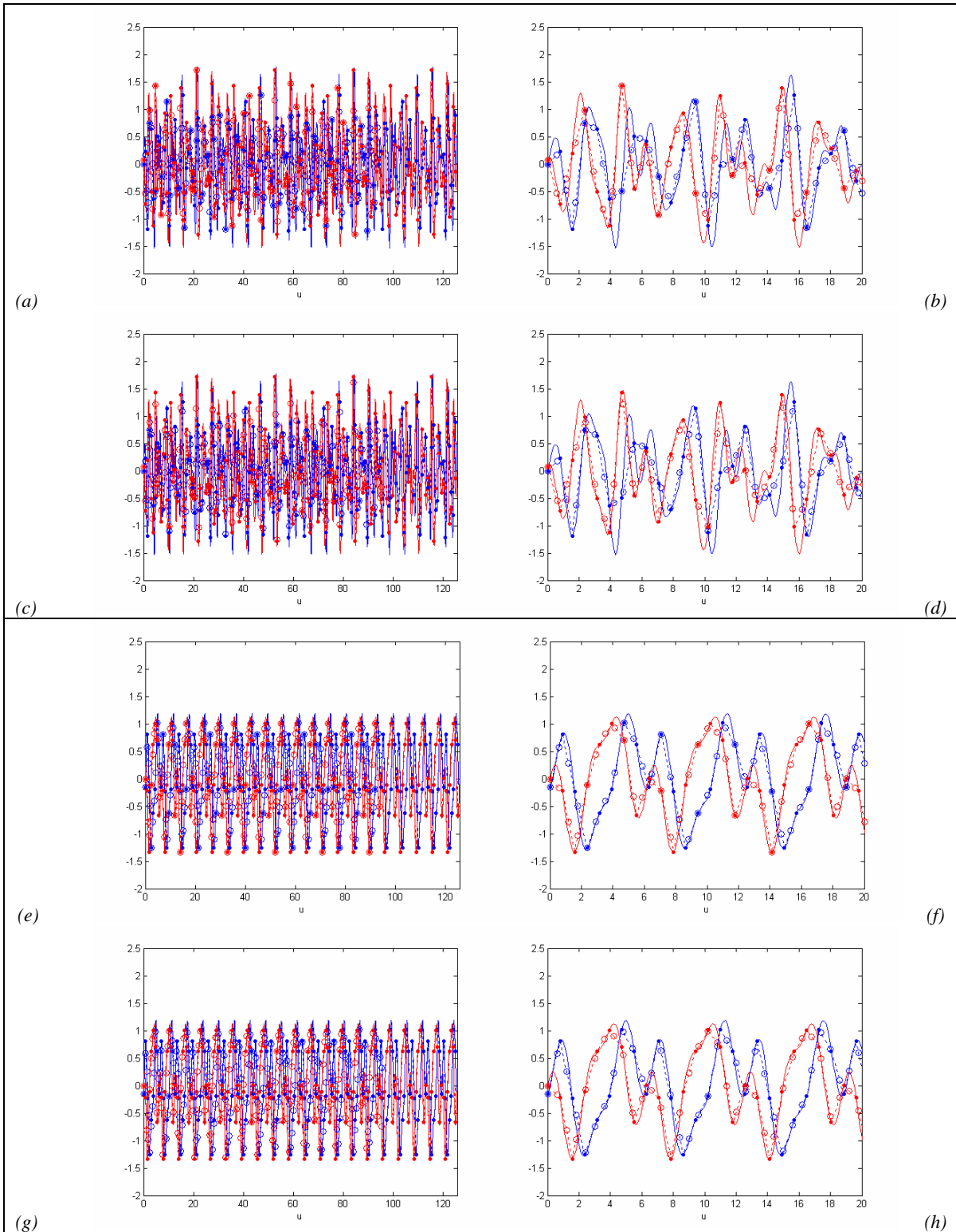
Figura 5-2-4: Interpolación en la transformada de Fourier directa mediante interpolación lineal, ejemplos II y III.
