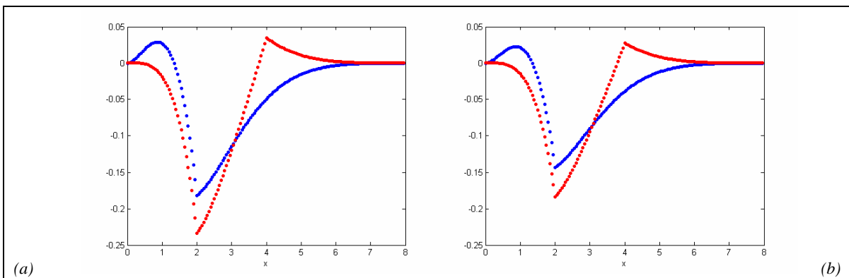
Figura 4-3-4: Transformada de Fourier inversa de funciones muestreadas con soporte acotado, Ejemplo I:
