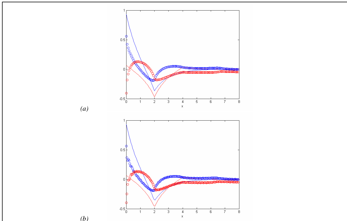
Figura 5-3-5: Relación entre la transformada inversa de la transformada directa interpolada mediante splines cúbicos y la función original, Ejemplo I.
