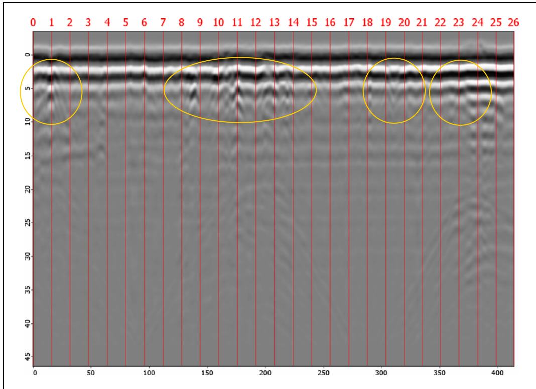
Figura 8-3-15: Mapa de color en tonos de gris del registro correspondiente al castro de El Ceremeño tras el filtrado espacial pasa baja (el blanco corresponde al valor mínimo, el negro al máximo). El eje de ordenadas expresa el tiempo doble de recorrido, en nanosegundos, y el eje de abscisas el número de traza. Las líneas verticales muestran la distancia desde el inicio del perfil, en metros. En amarillo se indican las señales a analizar.
