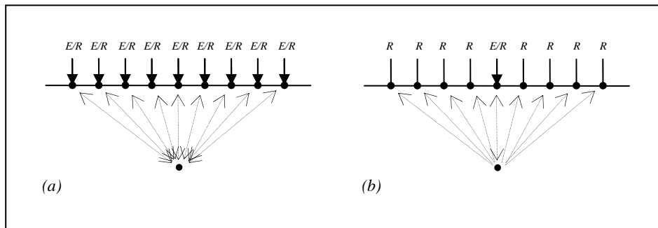
Figura 3–3-1: Representación de las situaciones a que hace referencia la §3.3.1.
