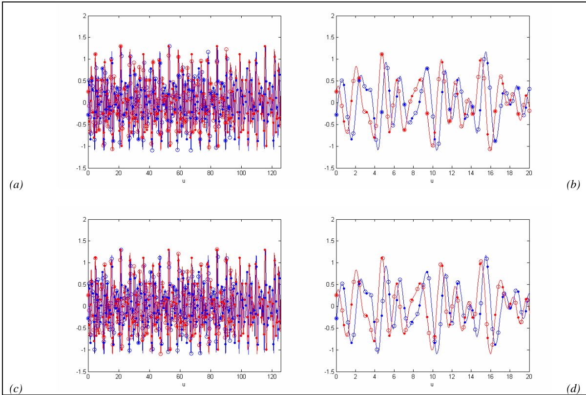
Figura 4–4-5: Interpolación en la transformada de Fourier directa mediante el Teorema del Muestreo generalizado (y II), Ejemplo II:
