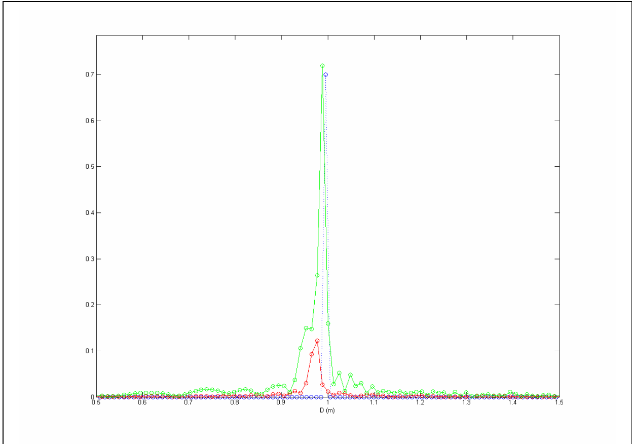
Figura 7-3-2: Trazas representativas de la DISTRIBUCIÓN MEDIDA, DISTRIBUCIÓN ESPERADA y DISTRIBUCIÓN DE REFLECTIVIDAD correspondientes al modelo bidimensional constituido por un único difractor puntual.
