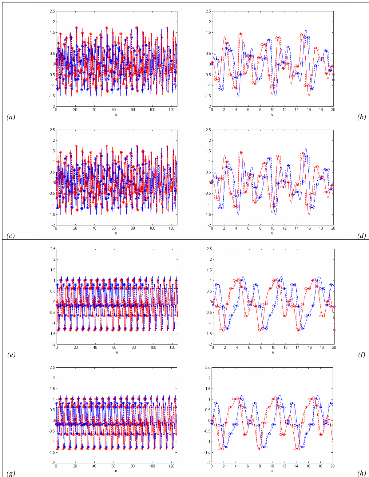
Figura 5-2-2: Interpolación en la transformada de Fourier directa mediante el método de vecinos más próximos, ejemplos II y III.
