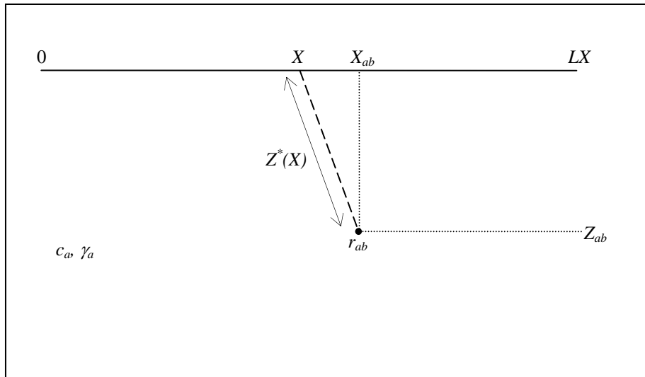
Figura 7–A-1: Planteamiento del Problema Directo para el modelo constituido por un difractor puntual.
