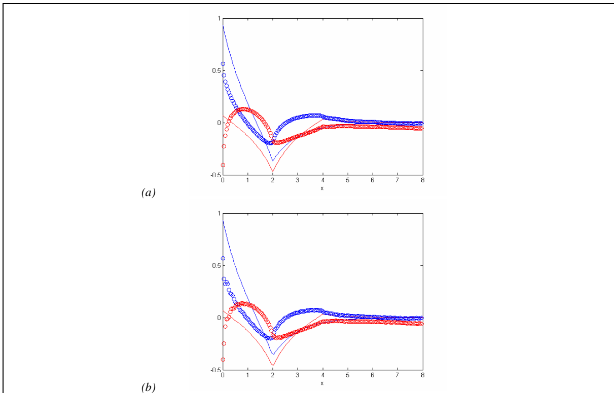
Figura 5–3-15: Relación entre la interpolación de la transformada inversa de la transformada directa interpolada por polinomios de Hermite cúbicos y la función original, Ejemplo I.
