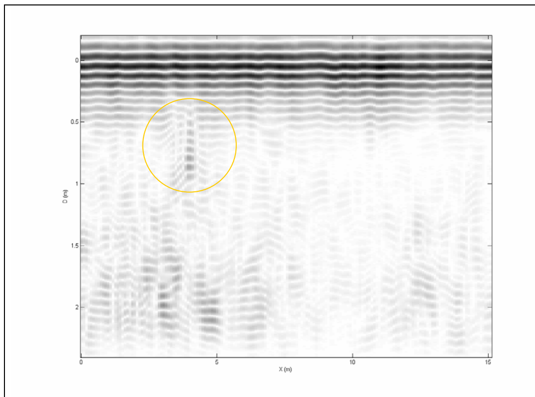
Figura 8-3-10: Mapa de color en tonos de gris de la DISTRIBUCIÓN MEDIDA correspondiente a la huerta del Monasterio de El Paular (el blanco corresponde al valor mínimo, el negro al máximo). El eje de ordenadas expresa la coordenada D y el eje de abscisas la distancia al origen, ambas en metros. En amarillo se indica la señal analizada.
