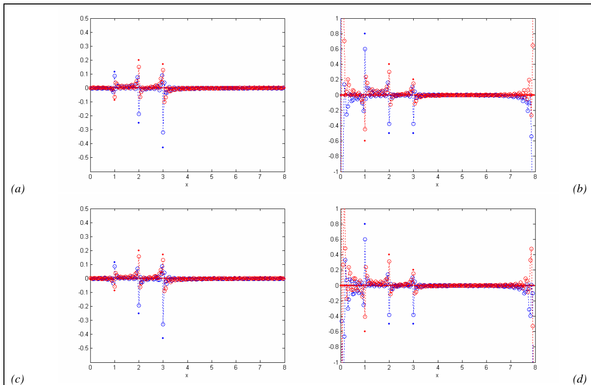
Figura 4-5-11: Relación entre la interpolación de la transformada inversa de la transformada directa interpolada mediante el Teorema del Muestreo generalizado y la función original (I), Ejemplo III:
