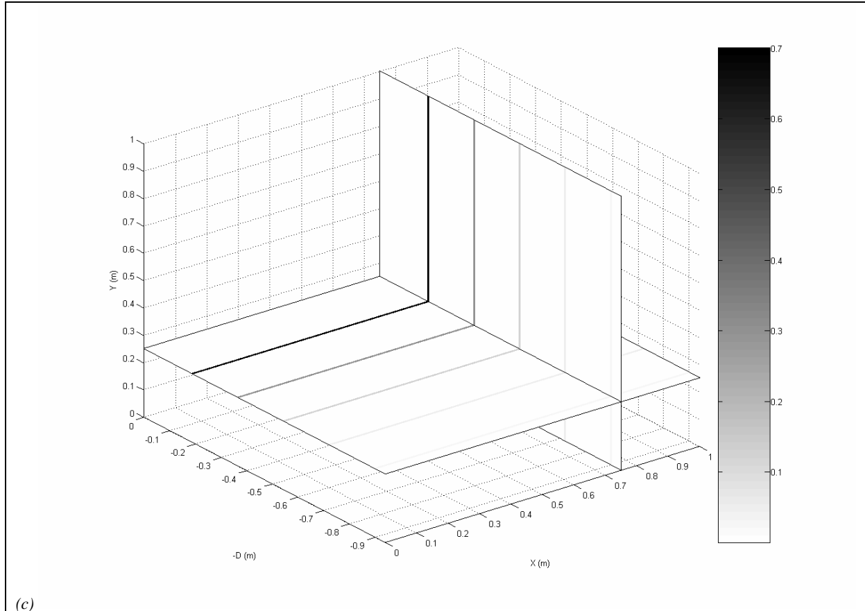
Figura 7-4-3: Comparación entre la DISTRIBUCIÓN MEDIDA y la DISTRIBUCIÓN ESPERADA con la DISTRIBUCIÓN DE REFLECTIVIDAD correspondientes al modelo tridimensional constituido por dos capas plano-paralelas sobre un semiespacio infinito.
