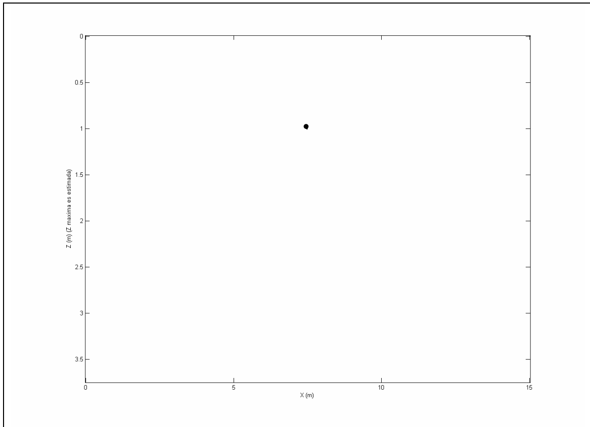
Figura 7-1-1: SECCIÓN DE ÍNDICES correspondiente al modelo bidimensional constituido por un único difractor puntual.
