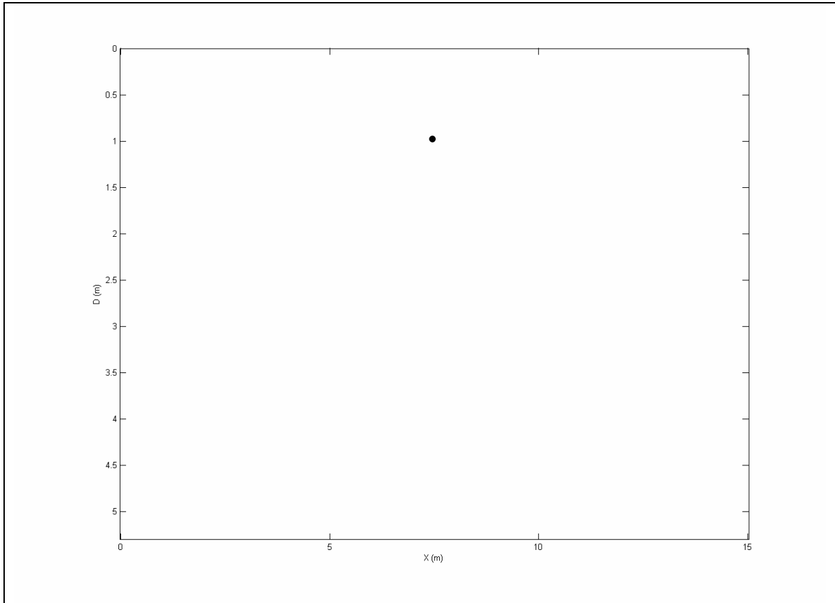
Figura 7-1-2: DISTRIBUCIÓN DE REFLECTIVIDAD correspondiente al modelo bidimensional constituido por un único difractor puntual. La reflectividad aparente del punto es r = 0,6805 + 0,0387i .
