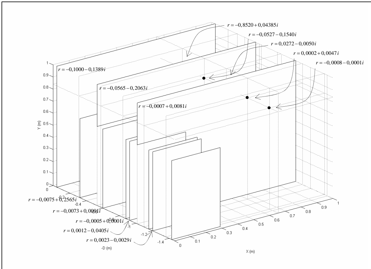
Figura 7-2-10: DISTRIBUCIÓN DE REFLECTIVIDAD correspondiente al modelo tridimensional realista. Junto a cada reflector se muestra la reflectividad aparente, en el caso en que las partes real o imaginaria sean apreciables.
