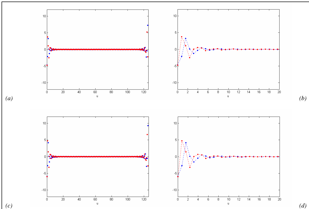
Figura 4–3-1: Transformada de Fourier directa de funciones muestreadas con soporte acotado, Ejemplo I:
