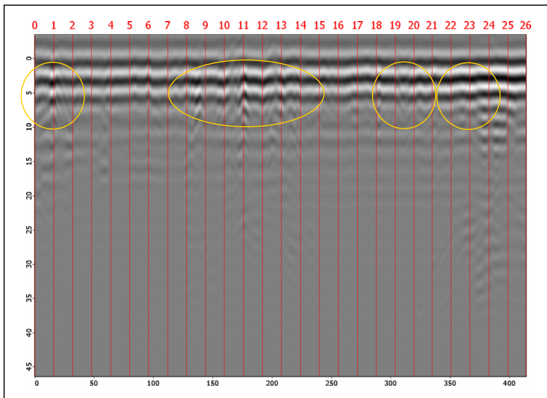
Figura 8-3-18: Mapa de color en tonos de gris del registro correspondiente al castro de El Ceremeño tras el filtrado temporal pasa banda (el blanco corresponde al valor mínimo, el negro al máximo). El eje de ordenadas expresa el tiempo doble de recorrido, en nanosegundos, y el eje de abscisas el número de traza. Las líneas verticales muestran la distancia desde el inicio del perfil, en metros. En amarillo se indican las señales a analizar.
