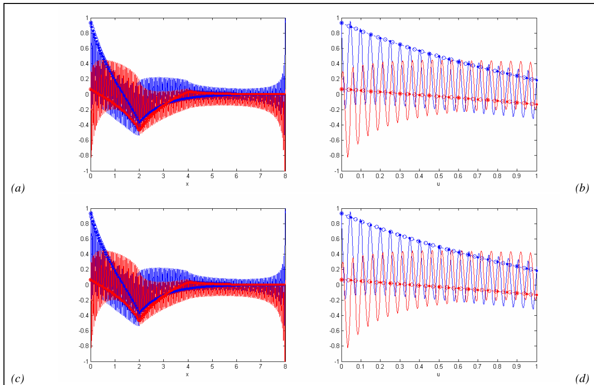
Figura 5–2-11: Interpolación en la transformada de Fourier inversa mediante interpolación lineal, Ejemplo I.
