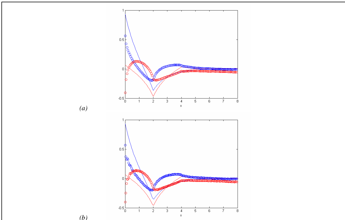
Figura 5–3-7: Relación entre la transformada inversa de la transformada directa interpolada por polinomios de Hermite cúbicos y la función original, Ejemplo I.
