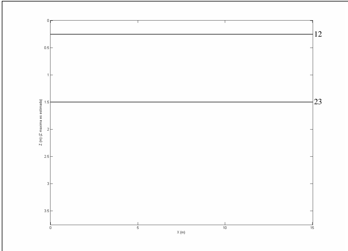
Figura 7-1-5: SECCIÓN DE ÍNDICES correspondiente al modelo bidimensional constituido por dos capas plano-paralelas sobre un semiespacio infinito. Junto a cada reflector se muestra el índice asociado.
