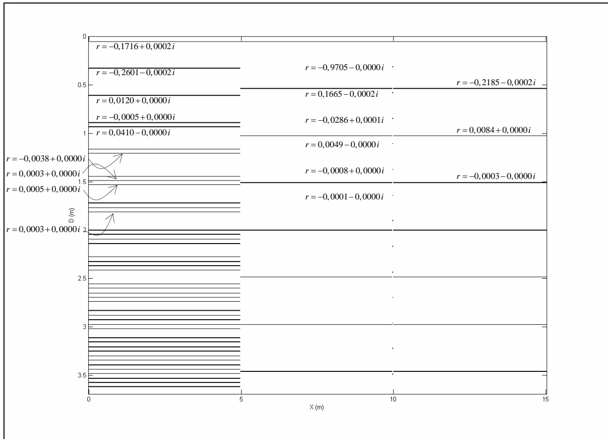
Figura 7-1-10: DISTRIBUCIÓN DE REFLECTIVIDAD correspondiente al modelo bidimensional realista. Junto a cada reflector se muestra la reflectividad aparente, en el caso en que las partes real o imaginaria sean apreciables.
