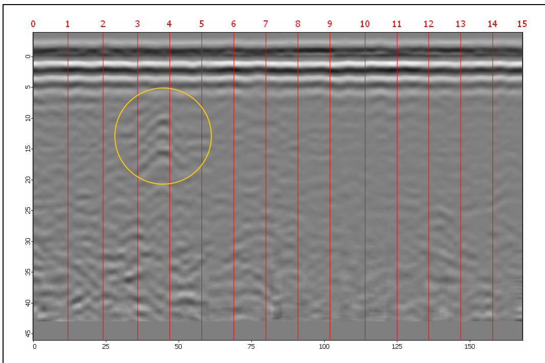
Figura 8-3-5: Mapa de color en tonos de gris del registro correspondiente a la huerta del Monasterio de El Paular tras el filtrado espacial pasa baja (el blanco corresponde al valor mínimo, el negro al máximo). El eje de ordenadas expresa el tiempo doble de recorrido, en nanosegundos, y el eje de abscisas el número de traza. Las líneas verticales muestran la distancia desde el inicio del perfil, en metros. En amarillo se indica la señal a analizar.
