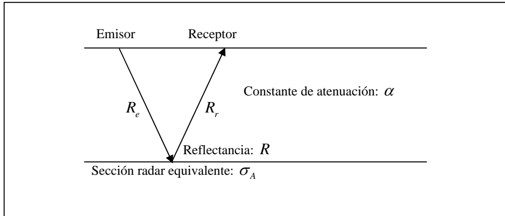
Figura 2-3-3: Diagrama para la determinación de la Ecuación del Radar.
