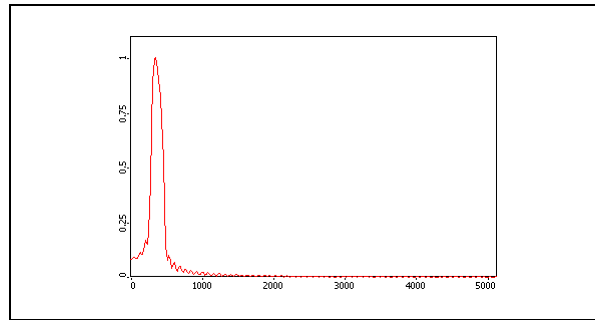
Figura 8-3-19: Espectro de potencia normalizado de la región del registro correspondiente al castro de El Ceremeño que contiene la señal objeto de estudio, tras el filtrado temporal. El eje de abscisas expresa la frecuencia, en MHz.
