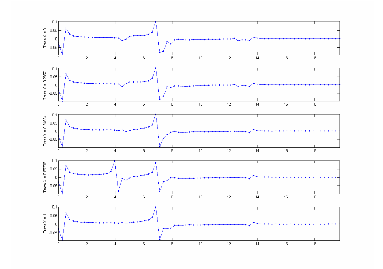
Figura 7-2-12: Trazas representativas de la SECCIÓN MEDIDA obtenida mediante la aplicación del algoritmo correspondiente al modelo tridimensional realista.
