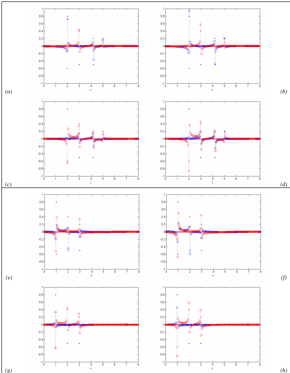
Figura 5-3-18: Relación entre la NUIFFT de la transformada directa interpolada y la función original, ejemplos II y III.
