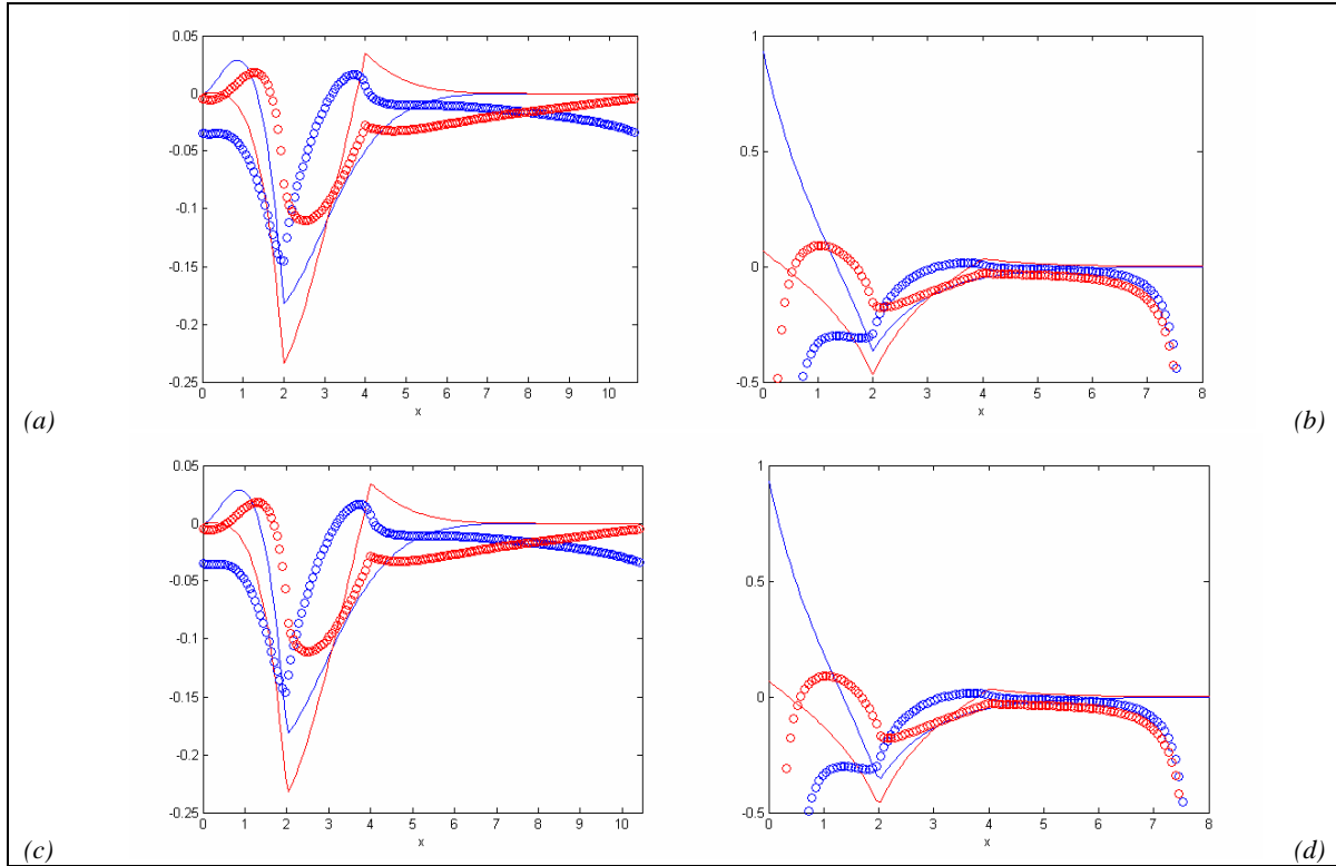
Figura 4-5-4: Relación entre la transformada inversa de la transformada directa interpolada mediante el Teorema del Muestreo generalizado y la función original (I), Ejemplo I:
