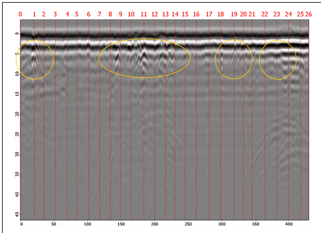
Figura 8–3-12: Mapa de color en tonos de gris del registro bruto correspondiente al castro de El Ceremeño (el blanco corresponde al valor mínimo, el negro al máximo). El eje de ordenadas expresa el tiempo doble de recorrido, en nanosegundos, y el eje de abscisas el número de traza. Las líneas verticales muestran la distancia desde el inicio del perfil, en metros. En amarillo se indican las señales a analizar.
