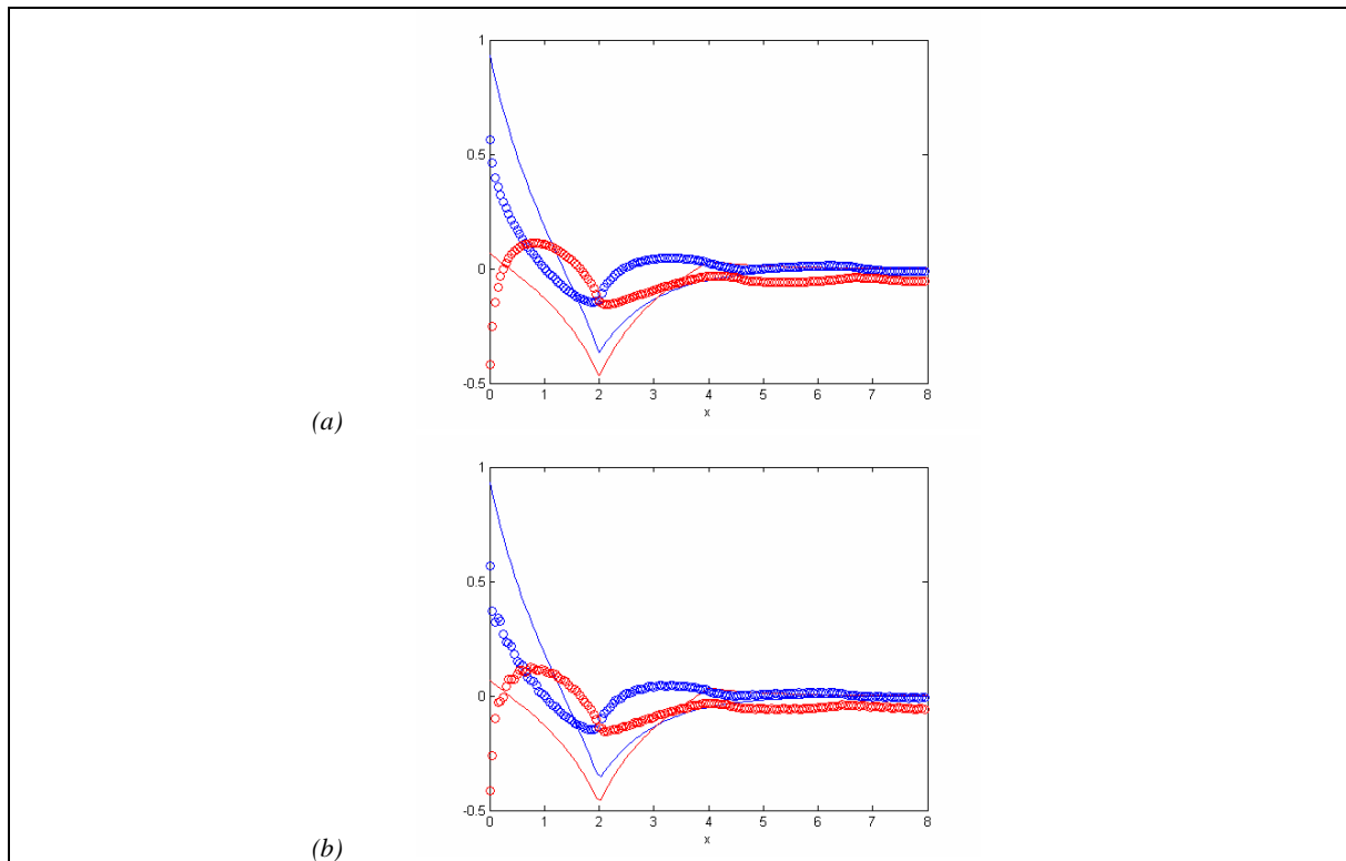
Figura 5–3-11: Relación entre la interpolación de la transformada inversa de la transformada directa interpolada mediante interpolación lineal y la función original, Ejemplo I.
