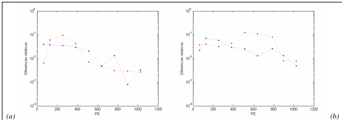
Figura 5-1-9: Residuos relativos correspondientes al modelo ajustado para el tiempo de cálculo óptimo vs. lf . Se muestran los resultados correspondientes a la evaluación directa (puntos) y el algoritmo de la convolución (asteriscos) para (a) la transformada directa y (b) la transformada inversa. Las líneas punteadas se incluyen para facilitar la observación de las tendencias.
