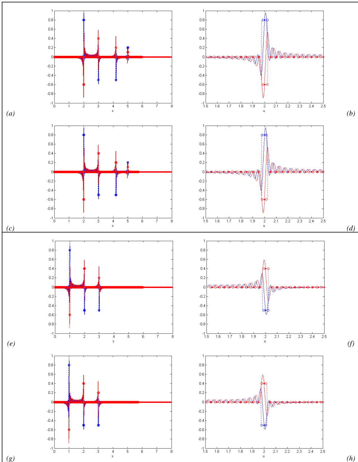
Figura 5–2-10: Interpolación en la transformada de Fourier inversa mediante el método de vecinos más próximos, ejemplos II y III.
