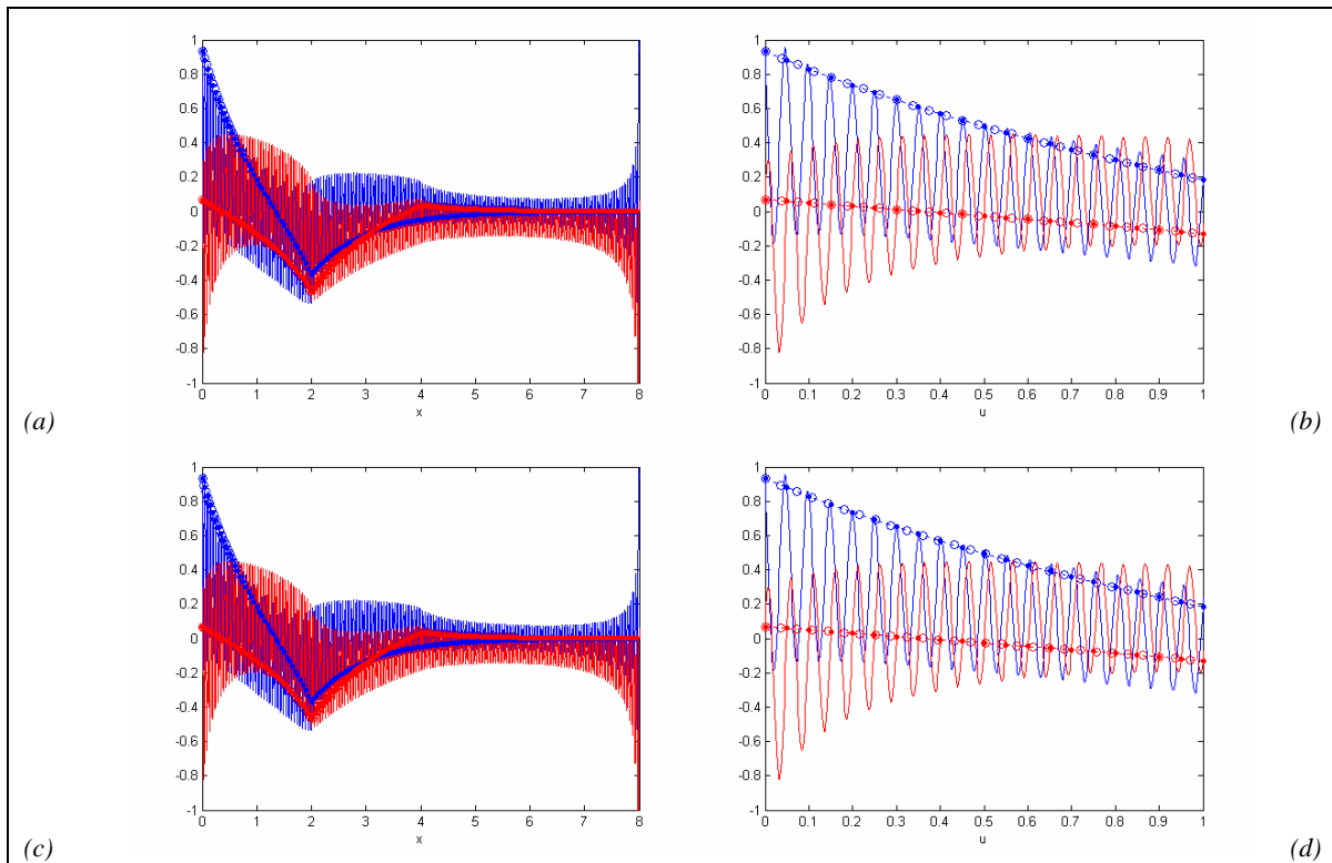
Figura 5–2-15: Interpolación en la transformada de Fourier inversa mediante interpolación por polinomios de Hermite cúbicos, Ejemplo I.
