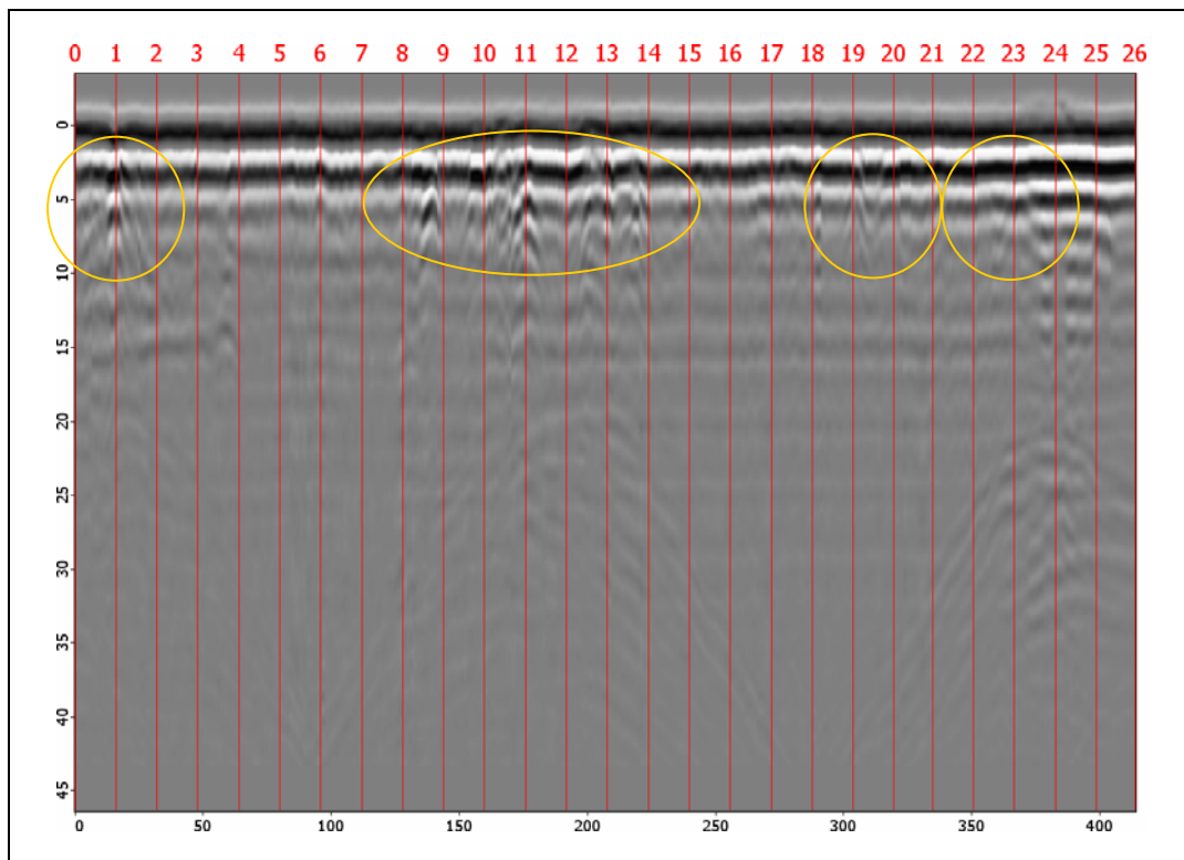
Figura 8-3-14: Mapa de color en tonos de gris del registro correspondiente al castro de El Ceremeño tras la interpolación en el eje espacial (el blanco corresponde al valor mínimo, el negro al máximo). El eje de ordenadas expresa el tiempo doble de recorrido, en nanosegundos, y el eje de abscisas el número de traza. Las líneas verticales muestran la distancia desde el inicio del perfil, en metros. En amarillo se indican las señales a analizar.
