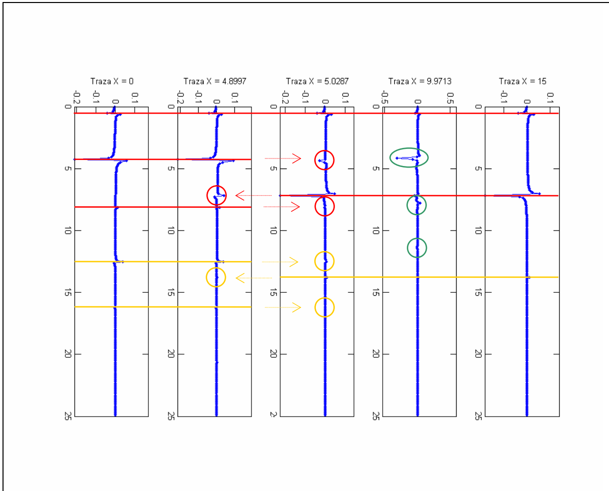
Figura 7-1-12: Trazas representativas de la SECCIÓN MEDIDA correspondiente al modelo bidimensional realista.
