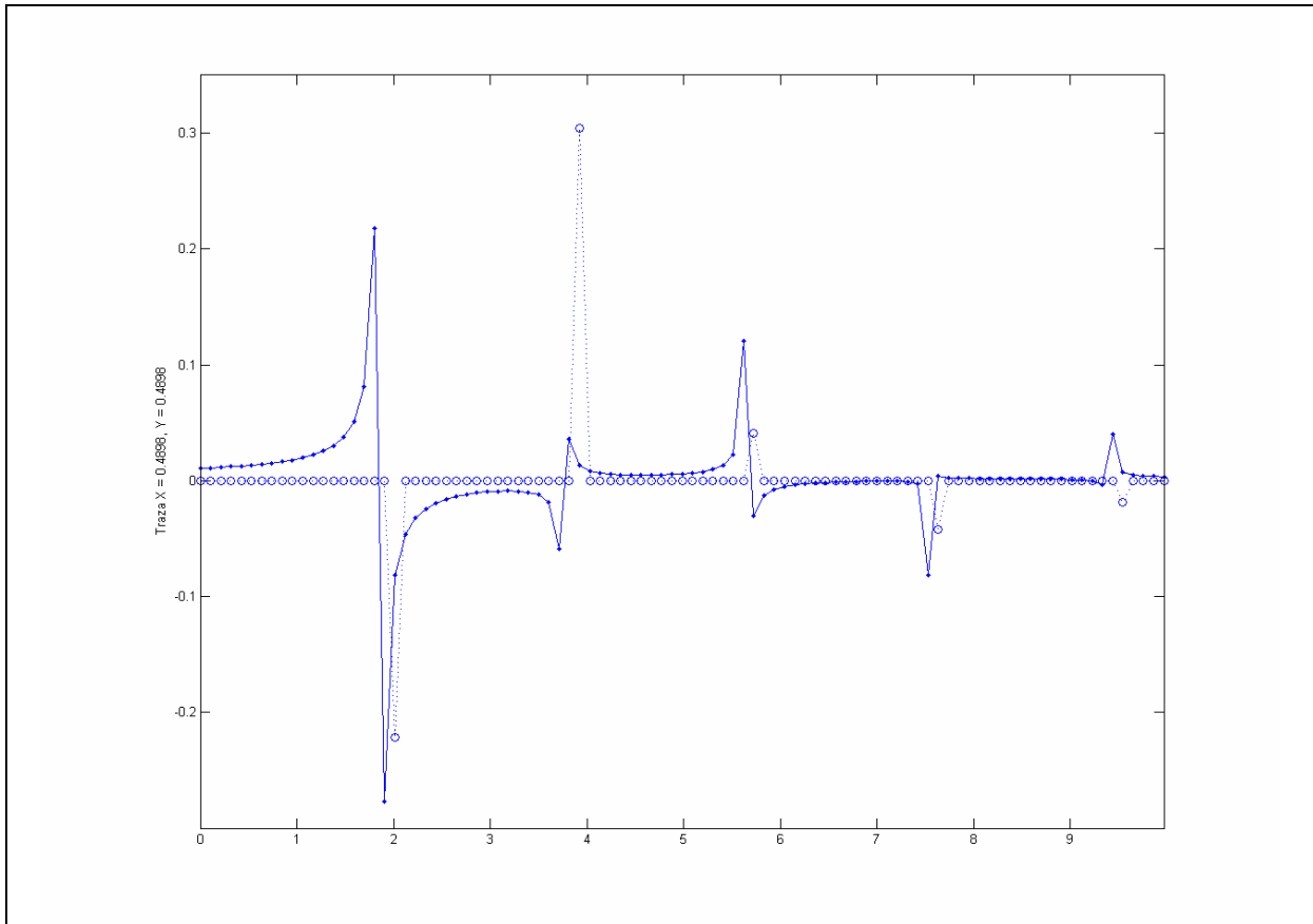
Figura 7-2-8: Trazas representativas de la SECCIÓN MEDIDA y la SECCIÓN ESPERADA correspondiente al modelo tridimensional constituido por dos capas plano-paralelas sobre un semiespacio infinito.
