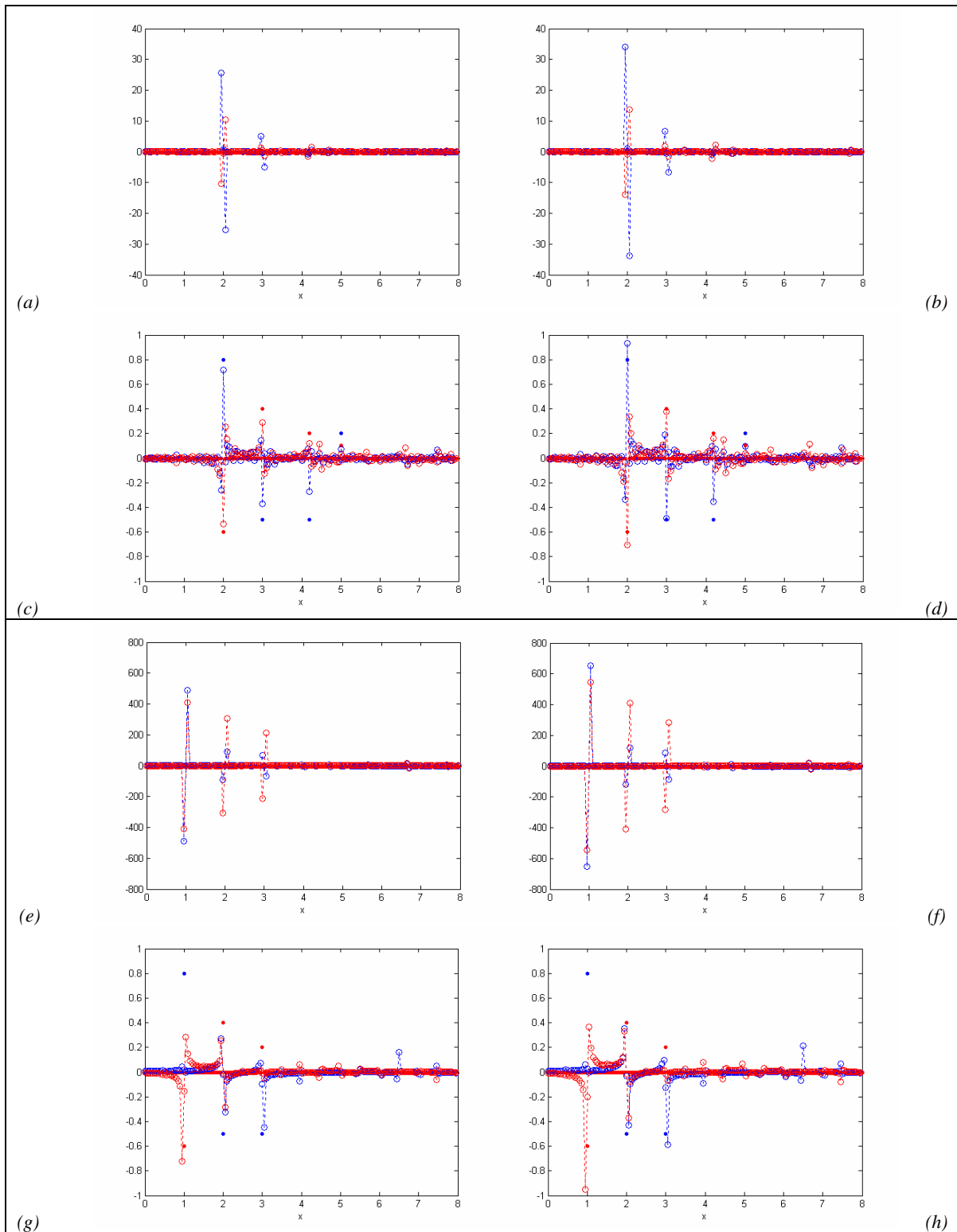
Figura 5-3-16: Relación entre la interpolación de la transformada inversa de la transformada directa interpolada por polinomios de Hermite cúbicos y la función original, ejemplos II y III.
