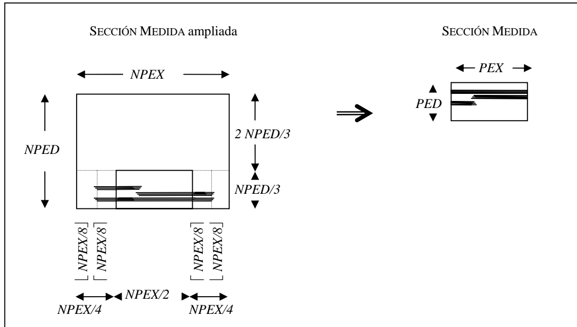
Figura 6-1-2: Reducción de la SECCIÓN MEDIDA.
