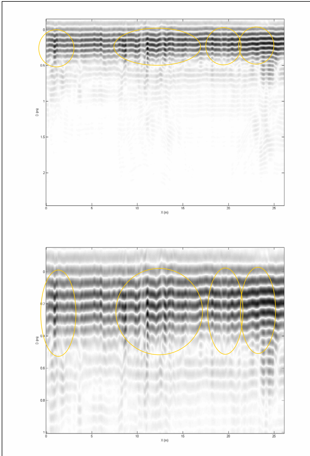
Figura 8-3-20: Mapa de color en tonos de gris de la DISTRIBUCIÓN MEDIDA correspondiente al castro de El Ceremeño (el blanco corresponde al valor mínimo, el negro al máximo) y detalle. El eje de ordenadas expresa la coordenada D y el eje de abscisas la distancia al origen, ambas en metros. En amarillo se indican las señales analizadas.
