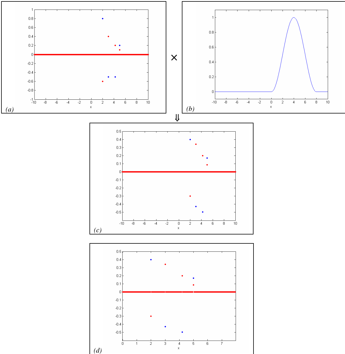
Figura 4–2-8: Funciones muestreadas con soporte acotado, Ejemplo II:
