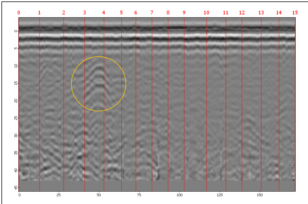
Figura 8-3-2: Mapa de color en tonos de gris del registro bruto correspondiente a la huerta del Monasterio de El Paular (el blanco corresponde al valor mínimo, el negro al máximo). El eje de ordenadas expresa el tiempo doble de recorrido, en nanosegundos, y el eje de abscisas el número de traza. Las líneas verticales muestran la distancia desde el inicio del perfil, en metros. En amarillo se indica la señal a analizar.
