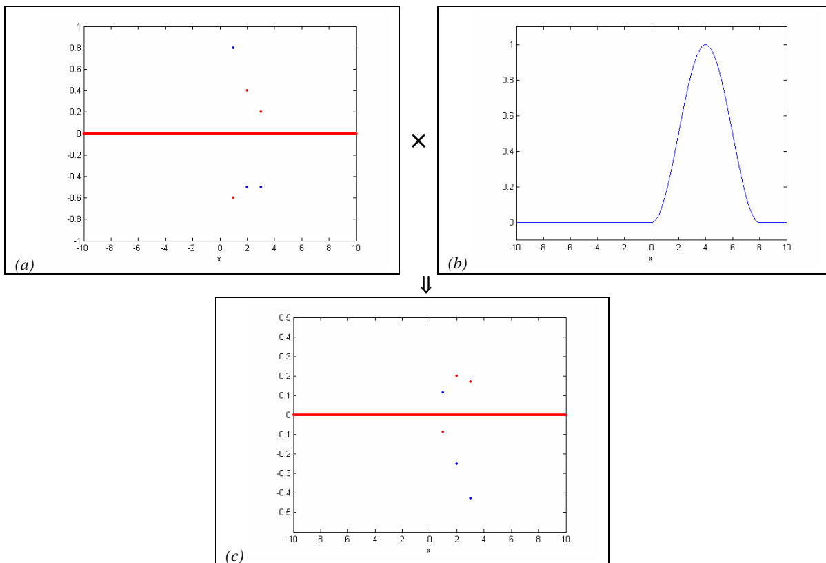
Figura 4–2-6: Acotación del soporte de funciones mediante la aplicación de ventanas, Ejemplo III:
