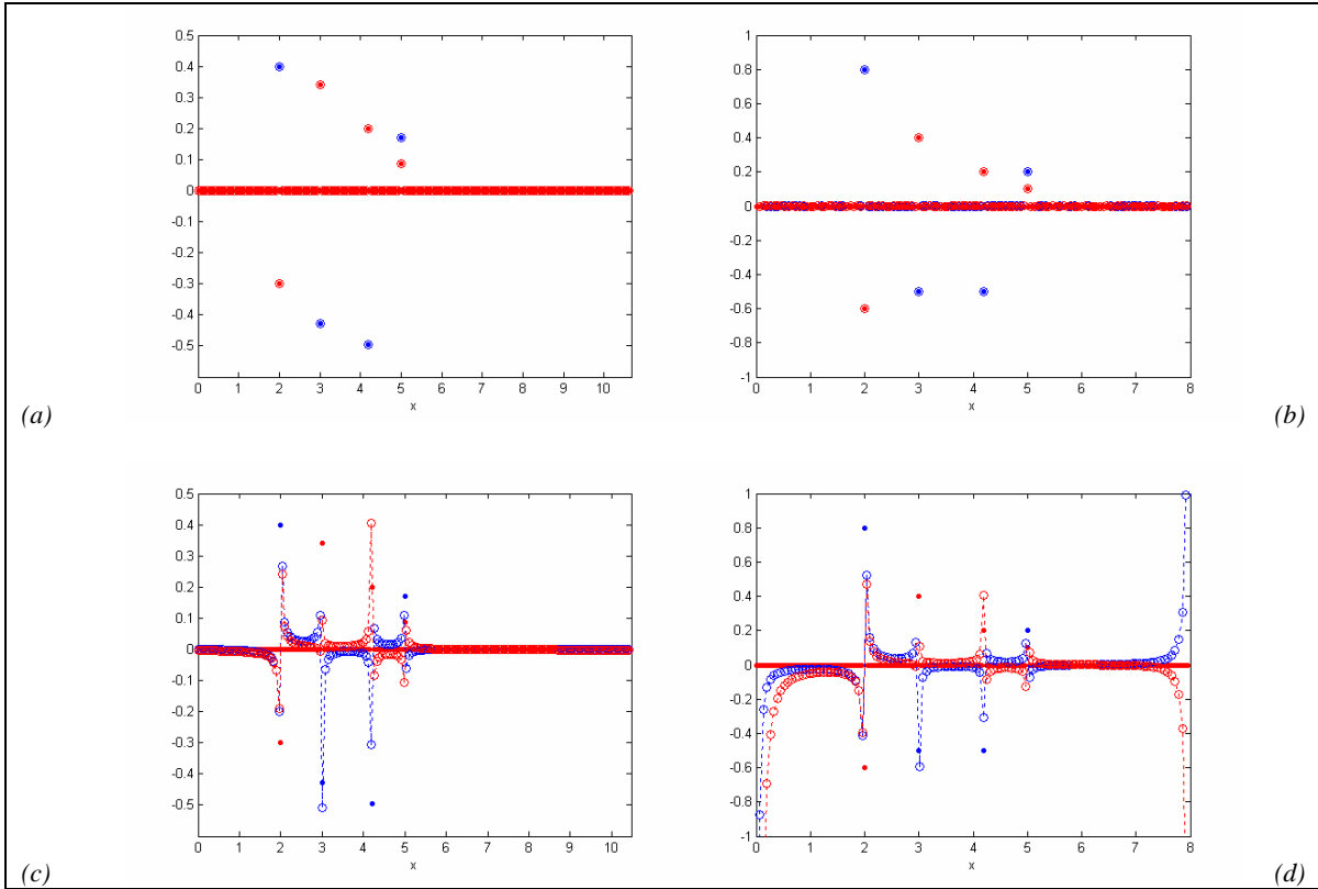
Figura 4-5-7: Relación entre la transformada inversa de la transformada directa interpolada mediante el Teorema del Muestreo generalizado y la función original (y II), Ejemplo II:
