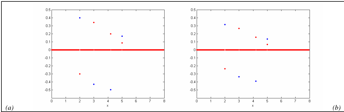
Figura 4-3-5: Transformada de Fourier inversa de funciones muestreadas con soporte acotado, Ejemplo II:
