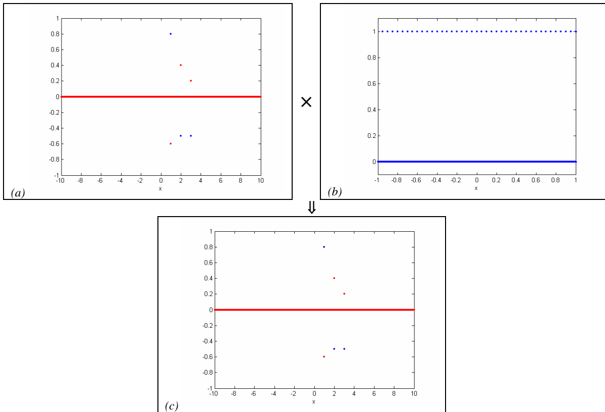
Figura 4-2-3: Muestreo de funciones, Ejemplo III:
