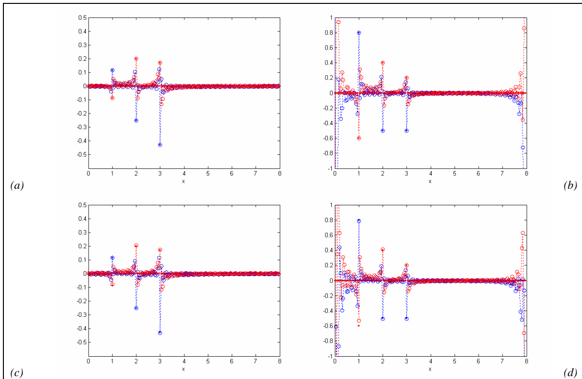
Figura 4-5-13: Relación entre la interpolación de la transformada inversa de la transformada directa interpolada mediante el Teorema del Muestreo generalizado y la función original (y II), Ejemplo III:
