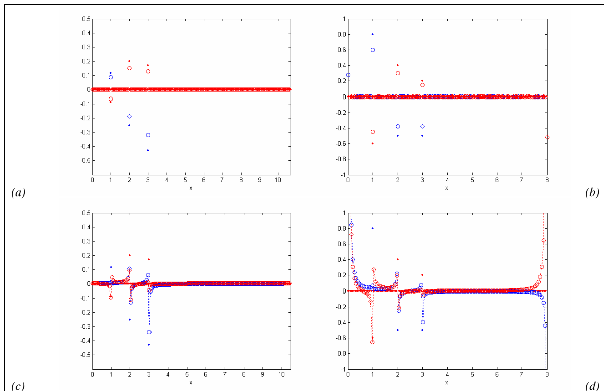
Figura 4–5-6: Relación entre la transformada inversa de la transformada directa interpolada mediante el Teorema del Muestreo generalizado y la función original (I), Ejemplo III:
