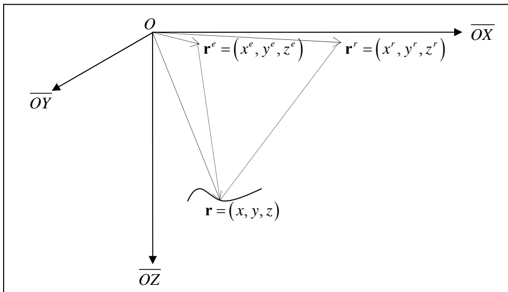
Figura 3-2-1: Sistema de coordenadas. Los vectores \mathbf{r}^e y \mathbf{r}^r denotan, respectivamente, la posición del emisor y el receptor; \mathbf{r} denota la posición de un punto genérico de la subsuperficie.
