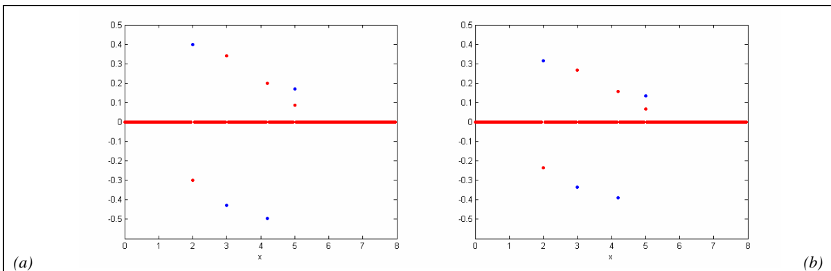
Figura 4-3-6: Transformada de Fourier inversa de funciones muestreadas con soporte acotado, Ejemplo III:
