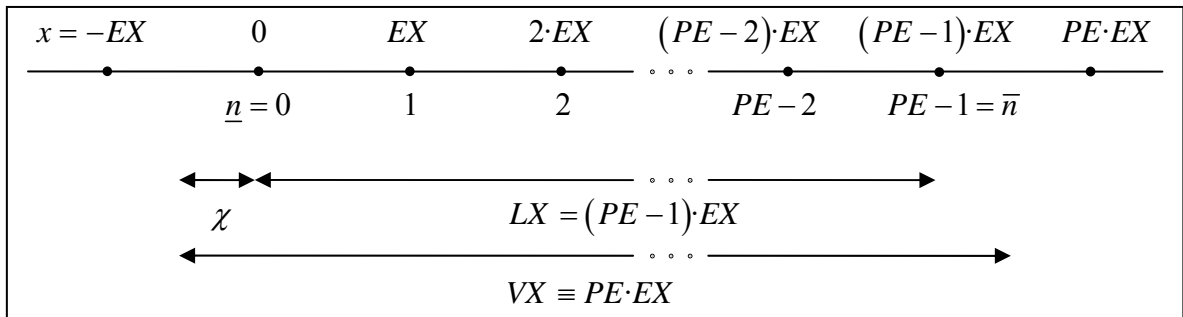
Figura 4-2-10: Elección de \chi y determinación de LX , VX y los índices n .
