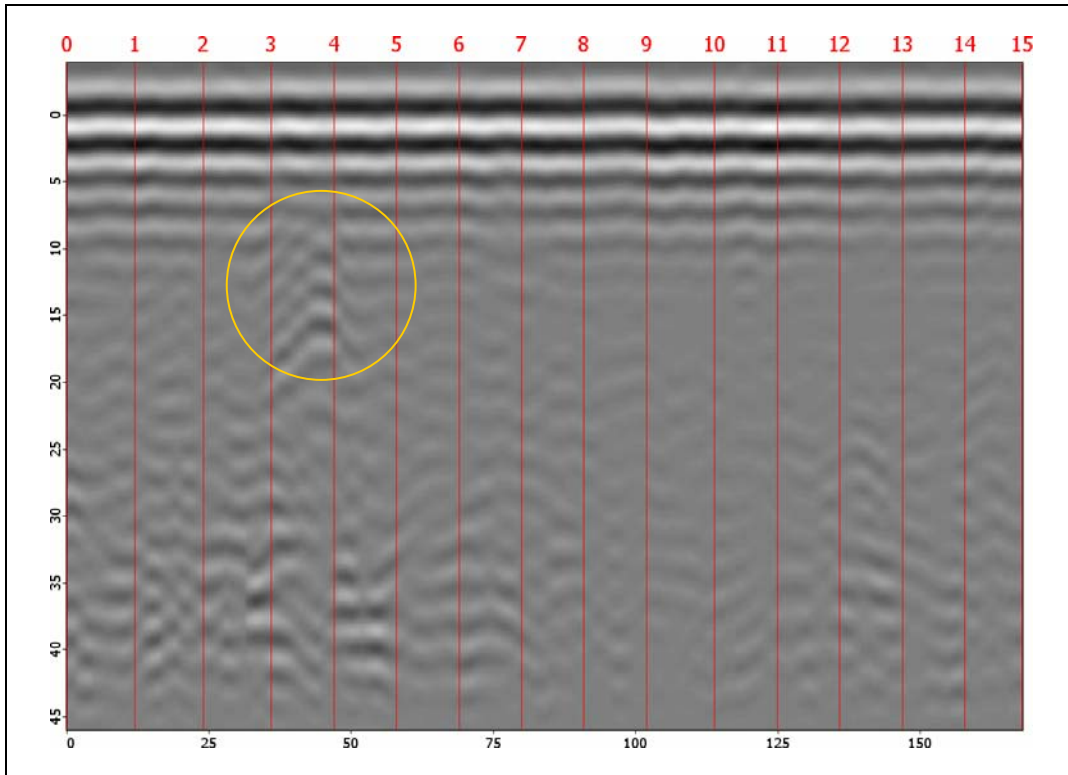
Figura 8-3-8: Mapa de color en tonos de gris del registro correspondiente a la huerta del Monasterio de El Paular tras el filtrado temporal pasa banda (el blanco corresponde al valor mínimo, el negro al máximo). El eje de ordenadas expresa el tiempo doble de recorrido, en nanosegundos, y el eje de abscisas el número de traza. Las líneas verticales muestran la distancia desde el inicio del perfil, en metros. En amarillo se indica la señal a analizar.
