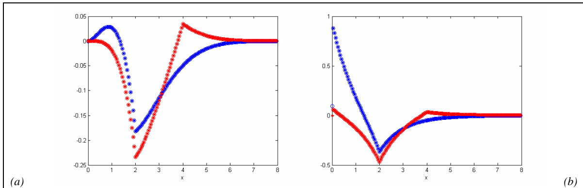
Figura 4-5-1: Relación entre la transformada inversa de la transformada directa y la función original, Ejemplo I:
