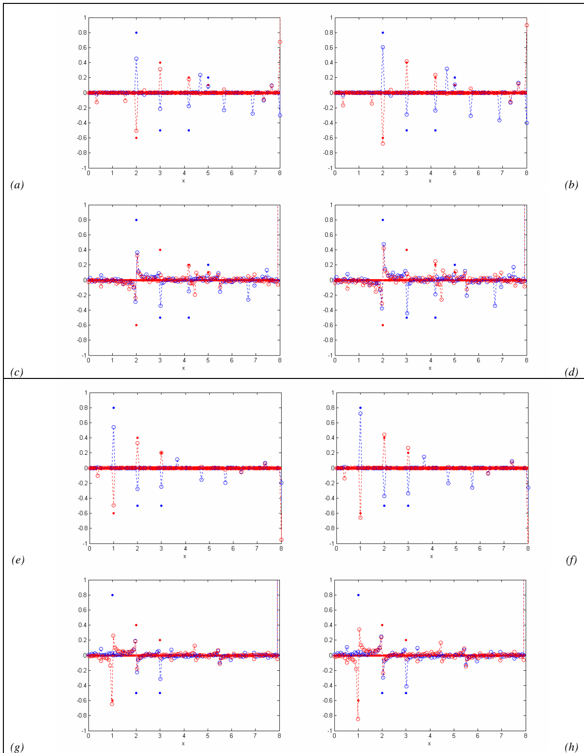
Figura 5-3-2: Relación entre la transformada inversa de la transformada directa interpolada mediante el método de vecinos más próximos y la función original, ejemplos II y III.
