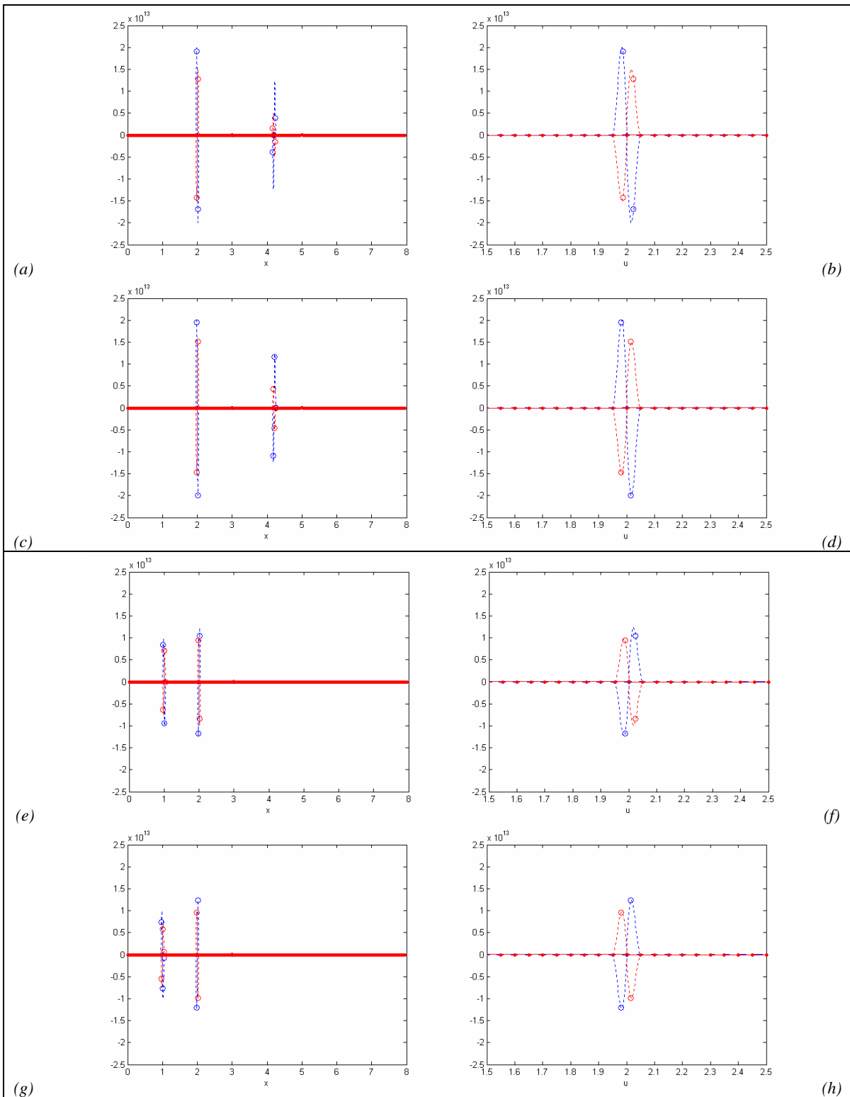
Figura 5-2-16: Interpolación en la transformada de Fourier inversa mediante interpolación por polinomios de Hermite cúbicos, ejemplos II y III.
