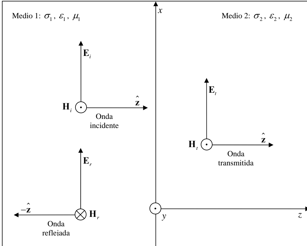
Figura 1-2-1: Ondas planas incidente (subíndice i ), reflejada (subíndice r ) y transmitida (subíndice t ) en la interfaz que separa los medios 1 y 2. El símbolo \odot (vs. \otimes ) representa un vector normal al plano de la hoja dirigido hacia el exterior (vs. interior).
