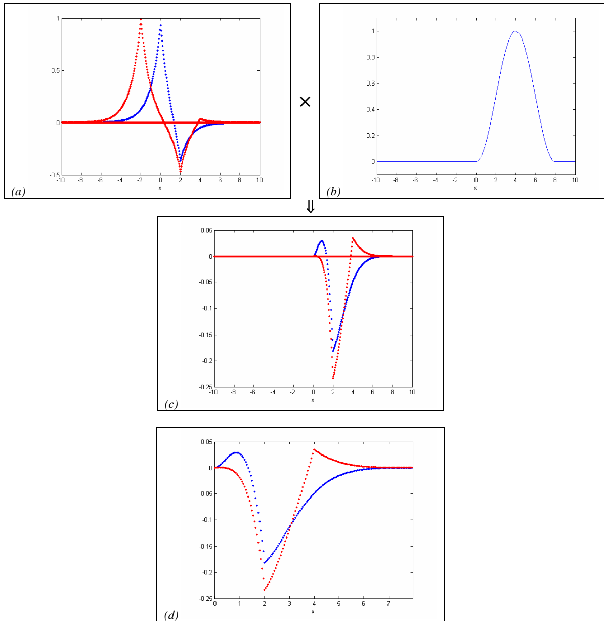
Figura 4–2-7: Funciones muestreadas con soporte acotado, Ejemplo I:
