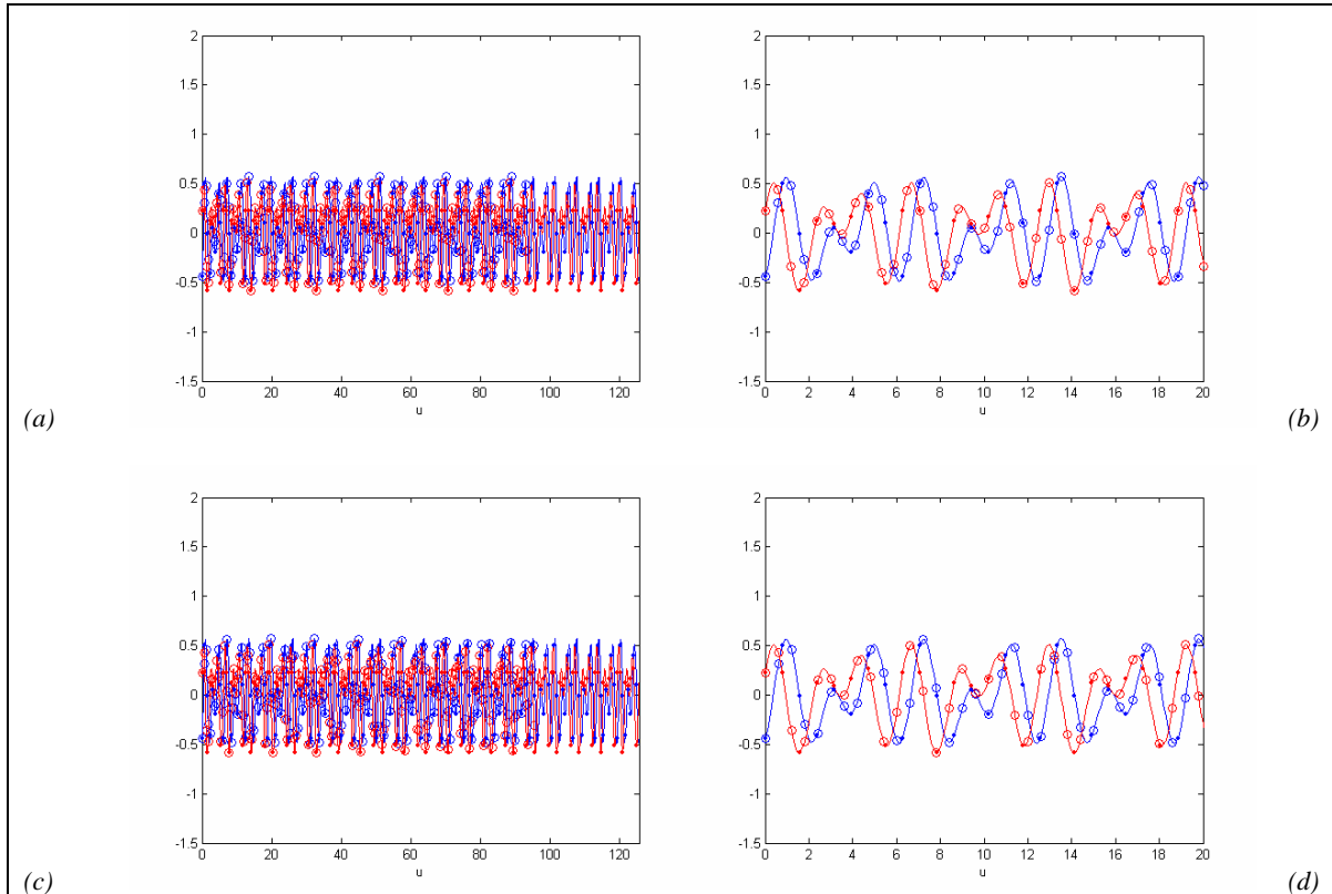
Figura 4–4-6: Interpolación en la transformada de Fourier directa mediante el Teorema del Muestreo generalizado (y II), Ejemplo III:
