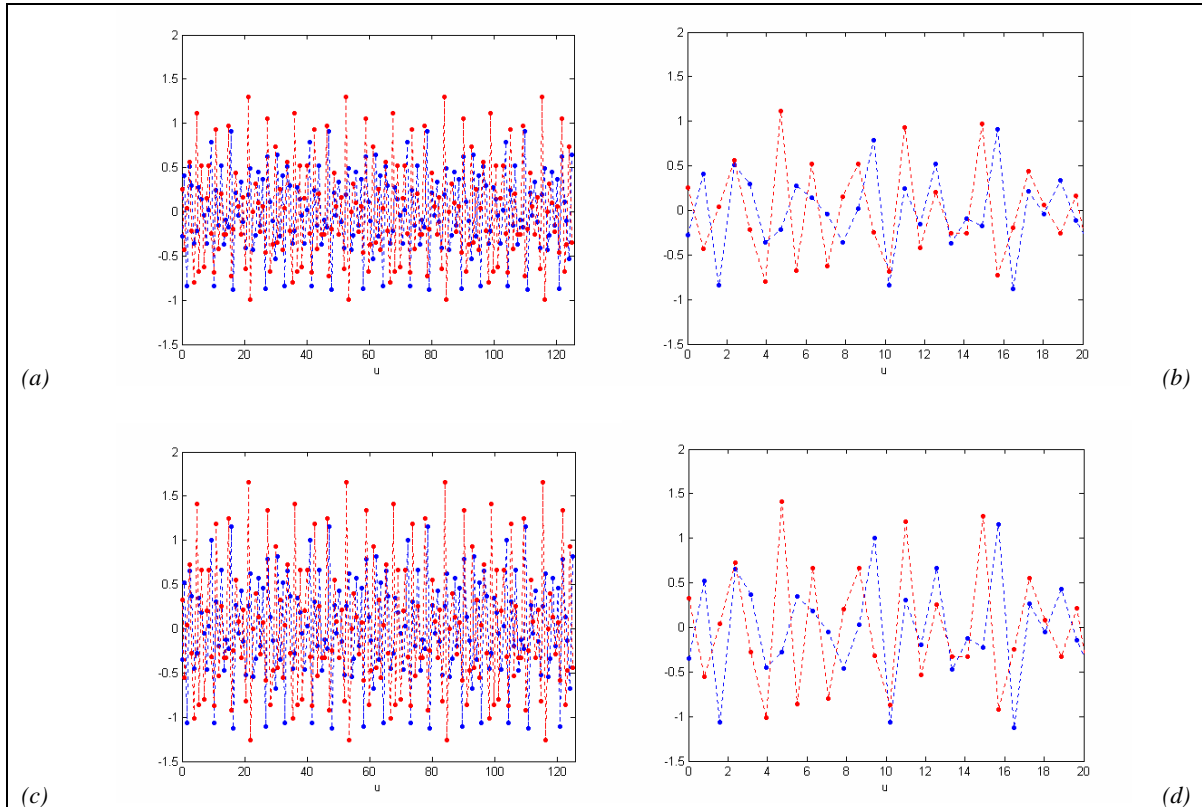
Figura 4–3-2: Transformada de Fourier directa de funciones muestreadas con soporte acotado, Ejemplo II:
