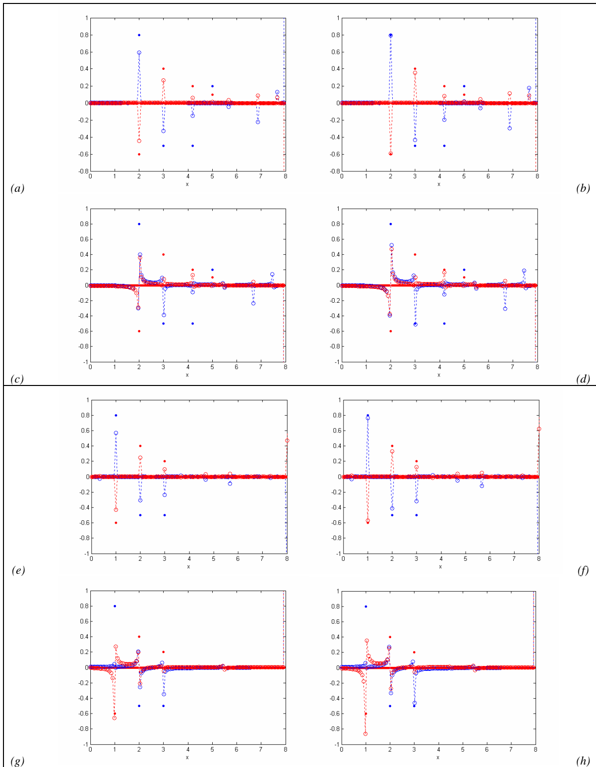
Figura 5-3-6: Relación entre la transformada inversa de la transformada directa interpolada mediante splines cúbicos y la función original, ejemplos II y III.
