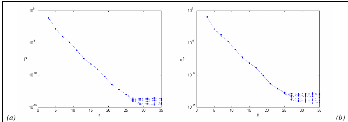
Figura 5-1-4: Variación del E_2 medio vs. lf . Los resultados para los valores de PE considerados se muestran para (a) la transformada directa y (b) la transformada inversa. Las líneas punteadas se incluyen para facilitar la observación de las tendencias.
