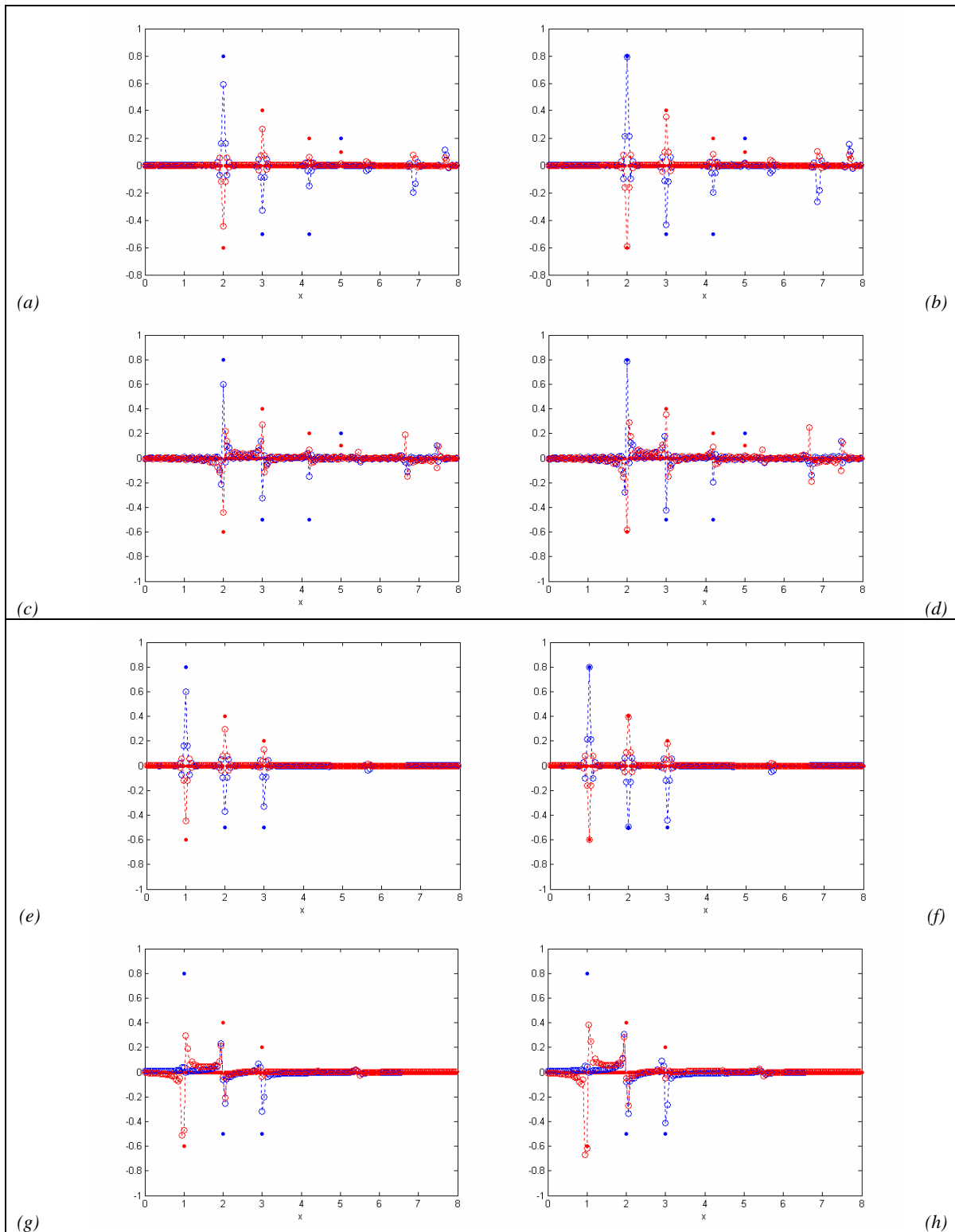
Figura 5-3-14: Relación entre la interpolación de la transformada inversa de la transformada directa interpolada mediante splines cúbicos y la función original, ejemplos II y III.
