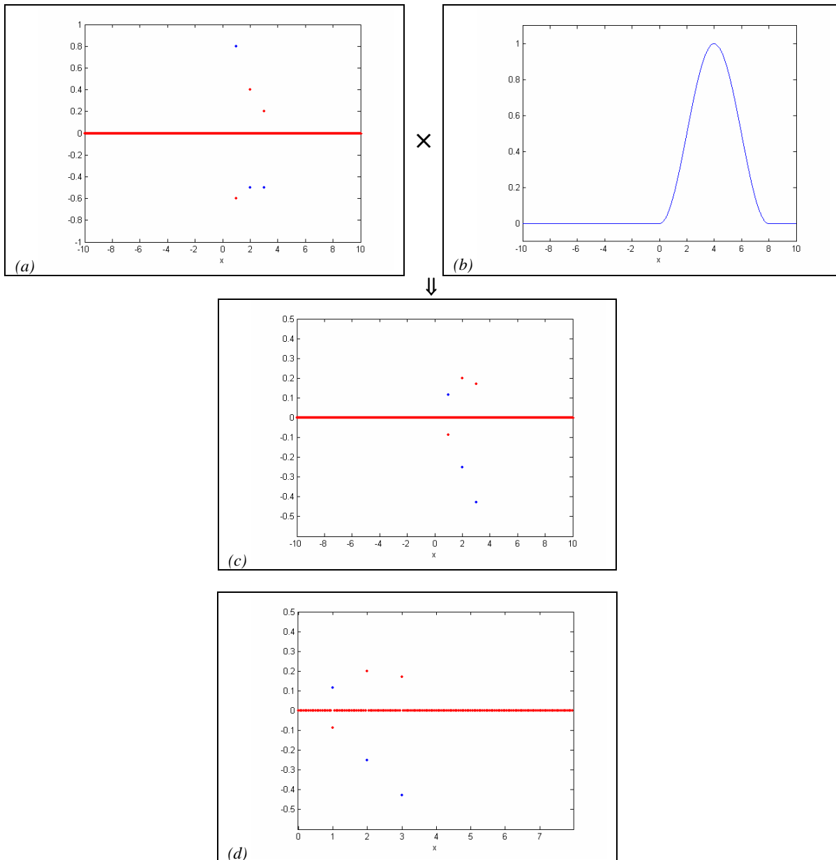
Figura 4–2-9: Funciones muestreadas con soporte acotado, Ejemplo III:
