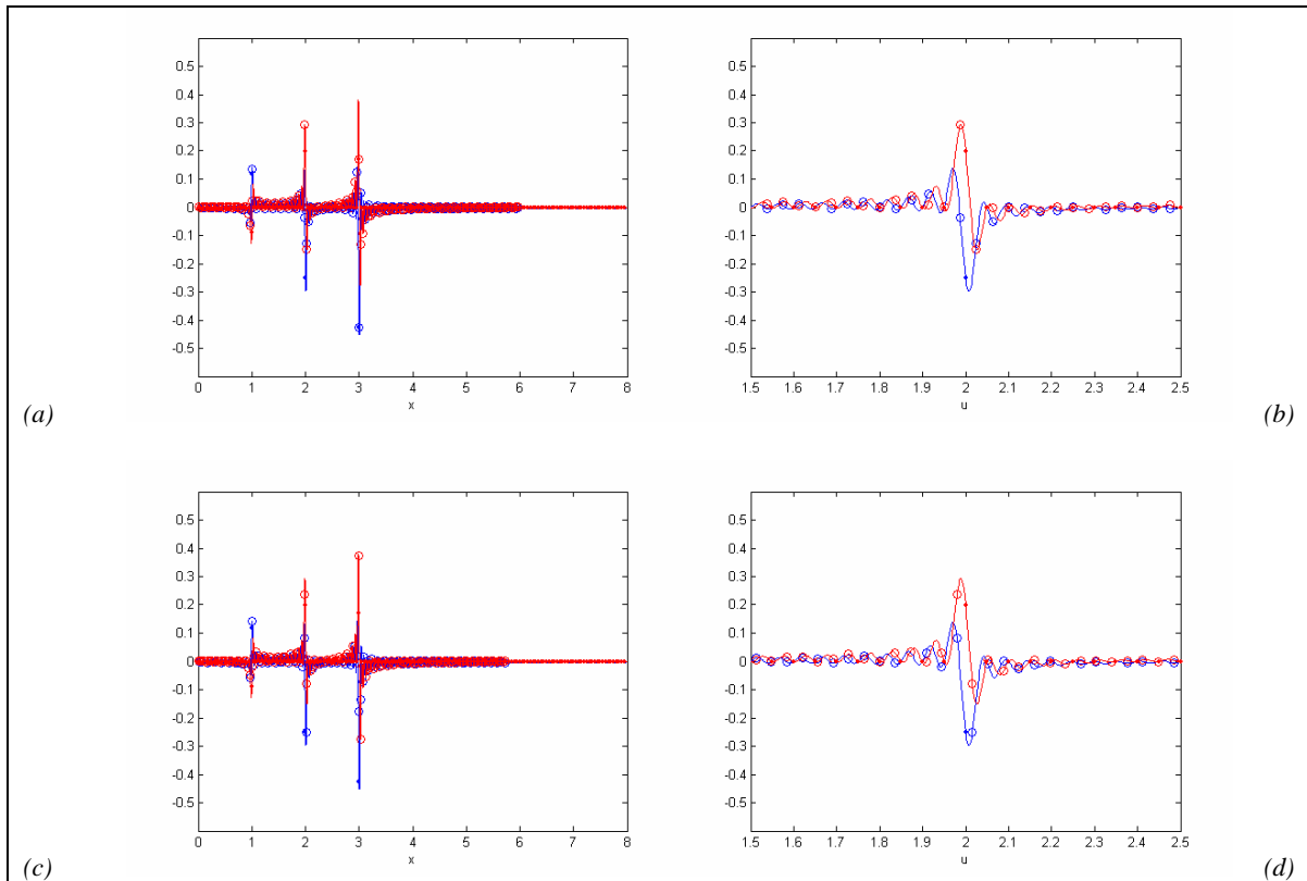
Figura 4-4-12: Interpolación en la transformada de Fourier inversa mediante el Teorema del Muestreo generalizado (y II), Ejemplo III:
