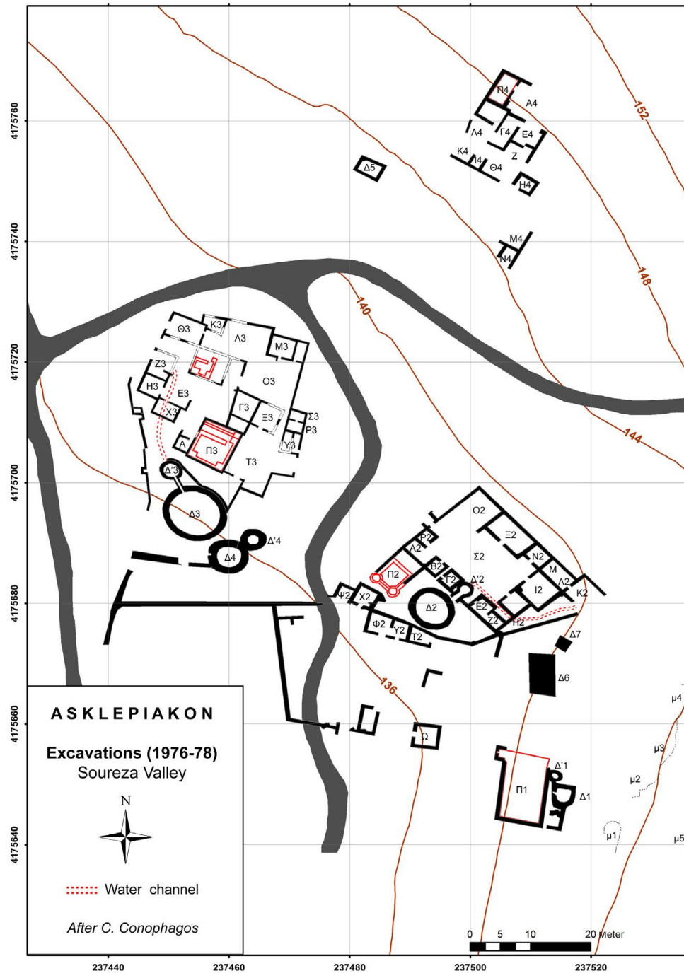
Fig. 7: Talleres del área conocida como “Asklepiakon”, Soureza (segunda mitad del s. IV a.C.)
