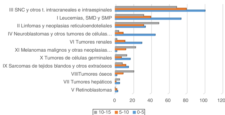
Figura 2 Categorías diagnósticas según grupos de edad. Años 1999 a 2016.
