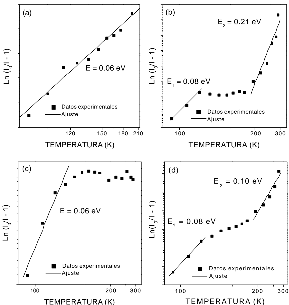
Figura 3.13 Evolución de la intensidad con la temperatura de las bandas de (a) 2.5–2.6 eV, (b) 2.32 eV, (c) 2.0 eV y (d) 1.67 eV en una muestra recristalizada en atmósfera de Ar. Se muestran los ajustes lineales utilizados para estimar la energía de activación.
