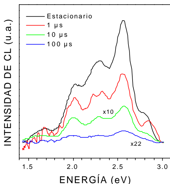
Figura 3.11. Espectros de CL de una muestra recristalizada en Ar tomados a 85 K con baja densidad de excitación en estado estacionario y diferentes tiempos de retardo.
