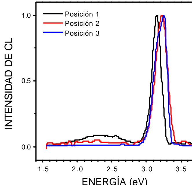
Figura 4.8. Espectros de CL normalizados a la unidad adquiridos a temperatura ambiente sobre las posiciones marcadas en la figura 4.7 (b).
