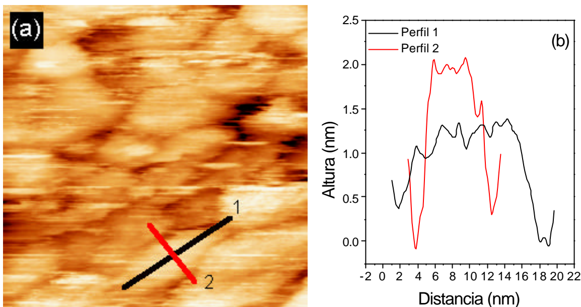
Figura 5.3. (a) Imagen de topografía en el STM adquirida con V_t = -1.8 \text{ V} e I_t = 0.2 \text{ nA} , el tamaño es de 55 \times 55 \text{ nm}^2 , (b) perfiles de altura realizados sobre la imagen anterior, la línea negra representa el perfil marcado con 1 y la roja el indicado con un 2.
