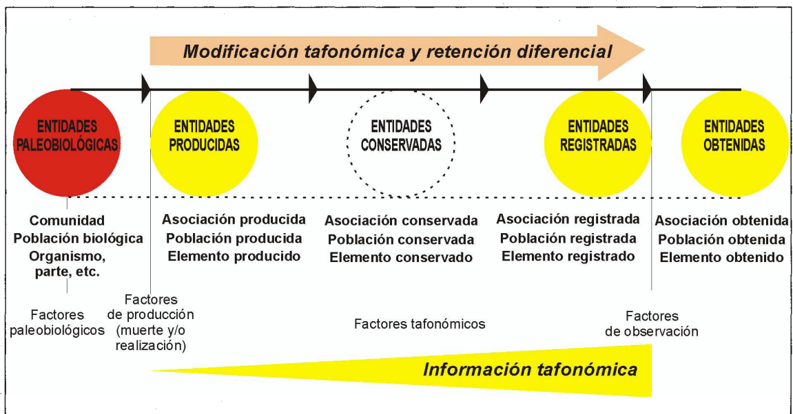
Fig. 2. Modelo de la fosilización entendida desde un planteamiento sistemista y evolucionista. La fosilización es un proceso no-paleobiológico, experimentado por entidades tafonómicas, que no implica pérdida o disminución de la información paleobiológica. Los factores tafonómicos no son necesariamente destructivos. La fosilización es un proceso capaz de incrementar la información tafonómica. Desde este punto de vista, el registro fósil está constituido por las entidades conservadas que han tenido mayor eficacia durante la alteración tafonómica, y que han sido producidas por entidades paleobiológicas o por otras entidades tafonómicas preexistentes (Fernández López, 2000).
