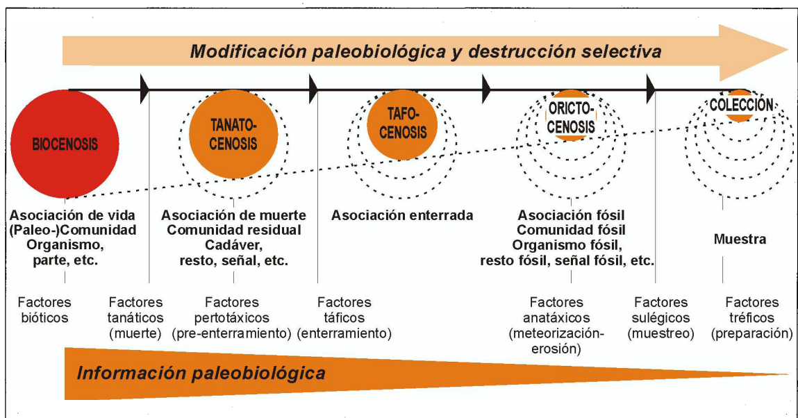
Fig. 1. Modelo de la fosilización entendido desde un planteamiento individualista o globalista y transformista. La fosilización es un proceso paleobiológico, experimentado por entidades biológicas del pasado, que implica pérdida o disminución de la información paleobiológica debido a los diferentes factores que han actuado como filtros sucesivos. Según esta concepción, el registro fósil está constituido por los vestigios más resistentes de las entidades paleobiológicas (Fernández López, 2000).
