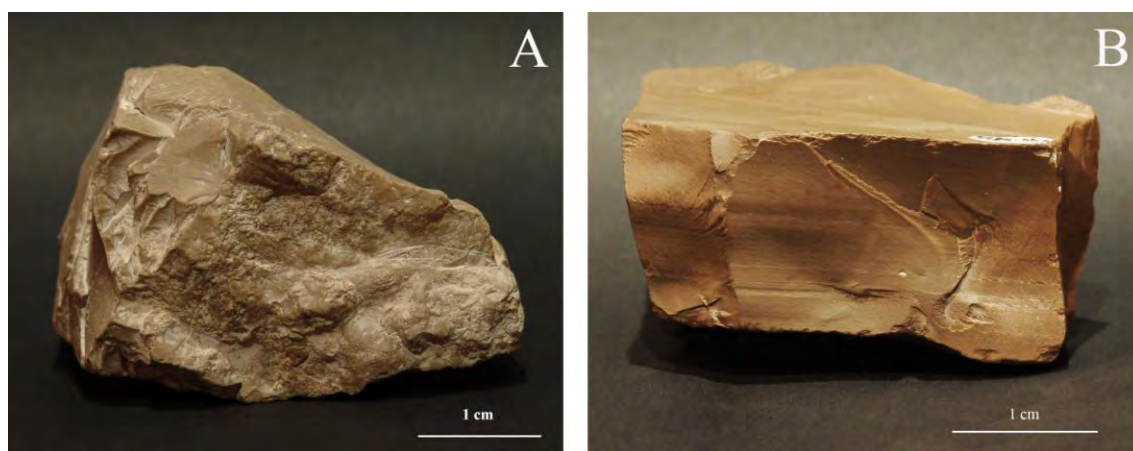
Figura 29. Caliza: A. Caliza. B. Caliza en la que se observa una ligera estratificación.
