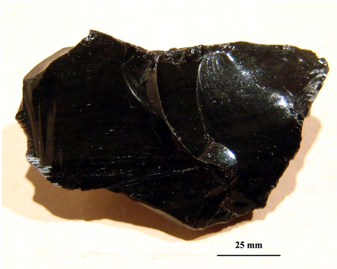
Figura 26. Obsidiana. Destaca la fracturación concéntrica.
