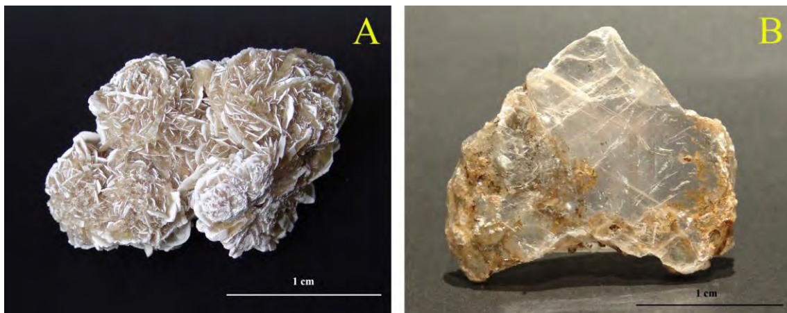
Figura 14. Yeso. A. Rosa del desierto. B. Cristal transparente de yeso variedad selenita.
