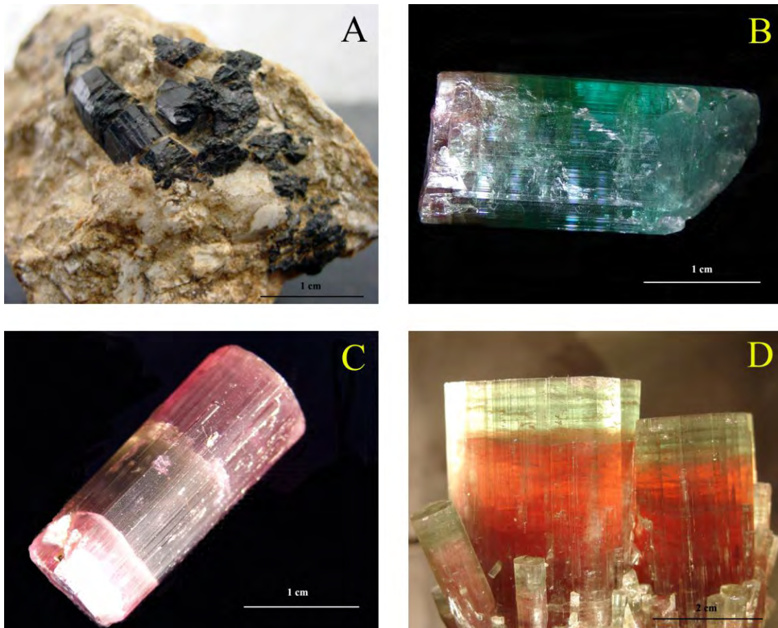
Figura 17. Variedades de turmalina: A. Chorlo. B. Verdelita. C. Rubelita. D. Turmalina zonada.
