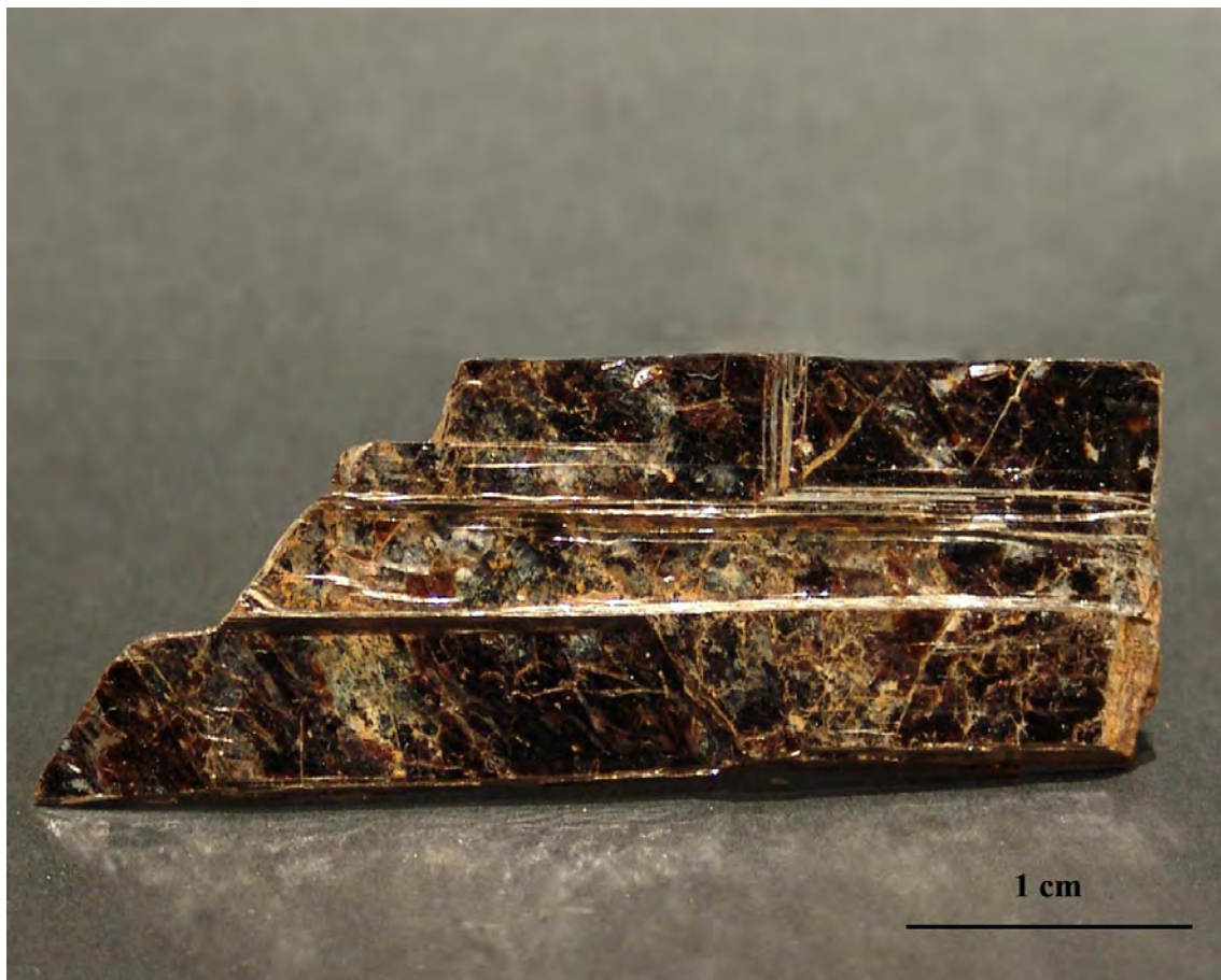
Figura 19. Agregado laminar de biotita.
