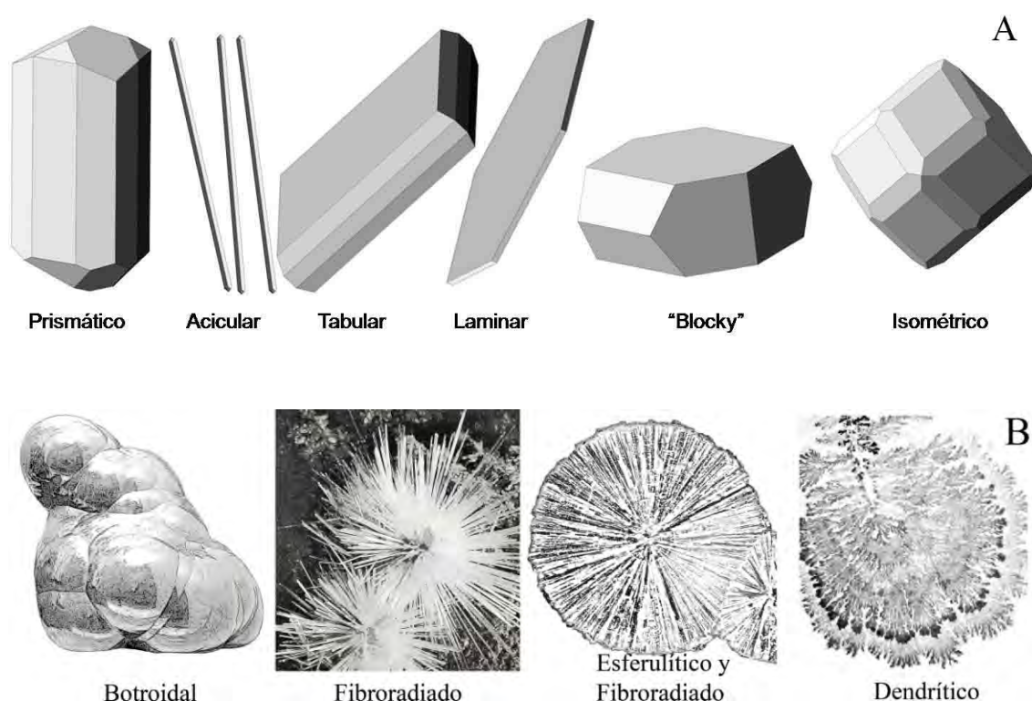
Figura 2. Hábitos cristalinos. A. Hábitos de monocristales. B. Hábitos de agregados cristalinos.
