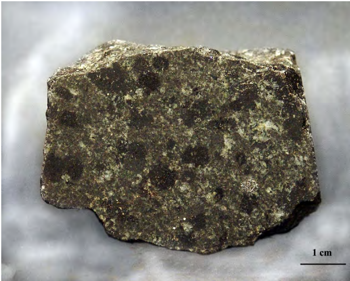
Figura 24. Basalto. Se observan cristales sobre una matriz vítrea.
