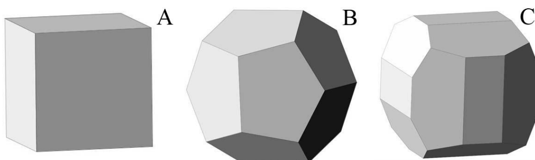
Figura 1. Algunas formas de la pirita. A. Cubo. B. Piritoedro. C. Combinación de cubo y piritoedro.
