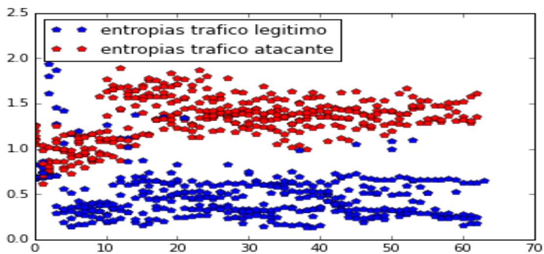
Figura 7.6: Entropías
