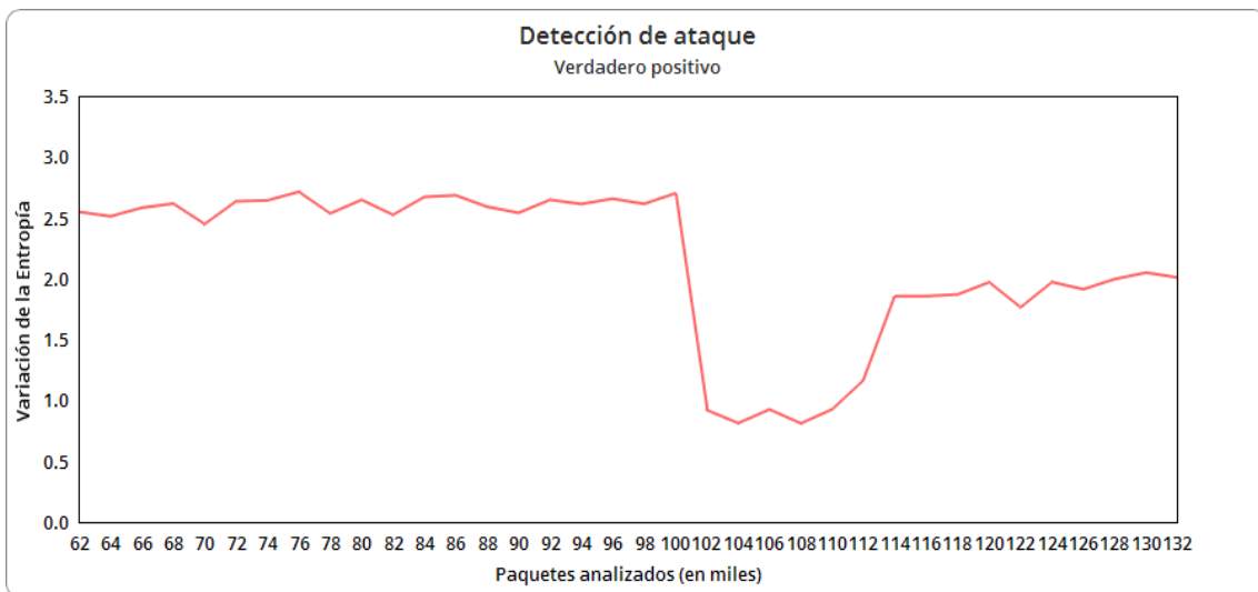
Figura 7.3: Ataque detectado
