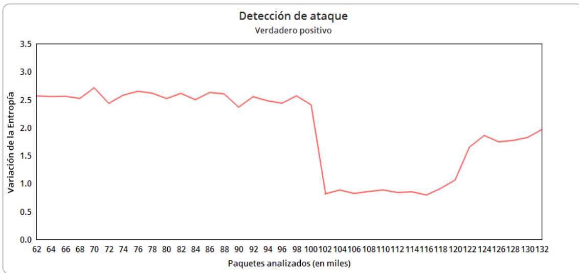
Figura 7.2: Ataque detectado
