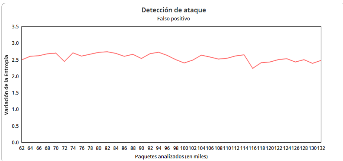
Figura 7.5: Falso positivo
