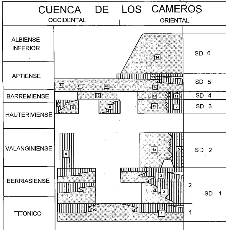
Figura 5.- a) Estratigrafía de la Cuenca de Los Cameros: Estratigrafía Secuencial del relleno de la cuenca. Secuencias Deposicionales (SD) y unidades estratigráficas: SD 1.1.- Alogrupo Tera (1). SD 1.2.- Alogrupo Oncala = Aloformación Huérteles (2) y Aloformación Valdeprados (3). SD 2.- Fms (4a) y Heterolítica inferior (5) del Gr Urbión; Fm Peñacoba (6). SD 3.- Fms (4b) y Cabretón (7) del Gr Urbión; Fm Galmayo (8); Fm (9); Fm Hortigüela (10). SD 4.- Fms (4c) y Heterolítica de transición (11) del Grupo Urbión; Fm Pantano (12). SD 5.- Fms (4d), Abejar (4e), (4f) y (4g) del Gr Urbión; Gr Enciso (13). SD 6.- Gr Oliván. Facies: siliciclásticas aluviales (punteado); carbonáticas lacustres (rayado vertical); mixtas (rayado vertical con punteado); carbonáticas con influencia marina (en blanco). La denominación de las unidades estratigráficas está basada en parte en: Tischer (1965, 1966), Platt (1989), Clemente y Alonso (1990), Salinas y Mas (1990), Gómez (1992) y Clemente et al. (1991). b) Estratigrafía de la Cuenca de Los Cameros: Sucesiones características en distintas zonas de la cuenca. Facies predominantes: 1.- areniscas, arenas y conglomerados; 2.- areniscas; 3.- lutitas y areniscas; 4.- Lutitas y areniscas con intercalaciones de calizas; 5.- Calizas, margas y arcillas lacustres (alguna incursión marina ocasional); 6.- calizas lacustres (alguna incursión marina ocasional); 7.- calizas lacustres y conglomerados aluviales; 8.- Jurásico marino (calizas y areniscas).
