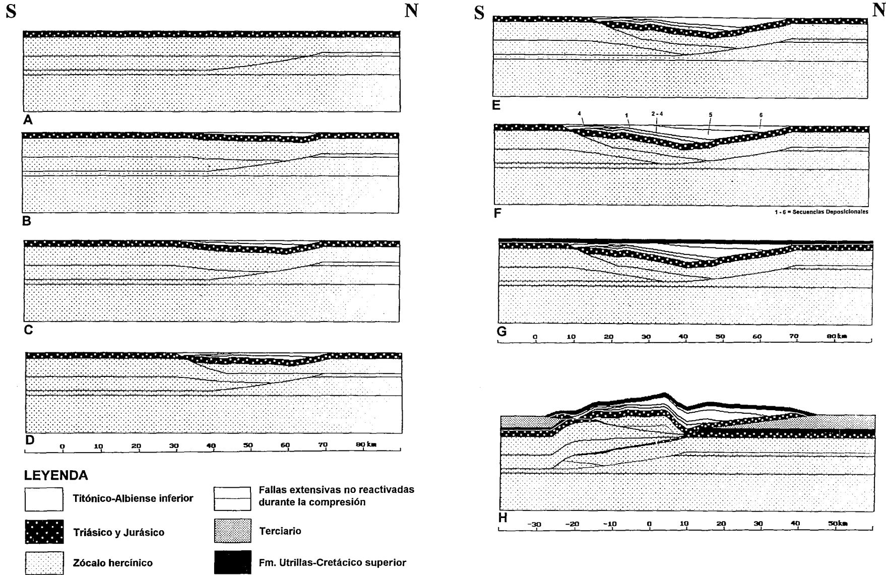
Figura 10.- Hipótesis propuesta sobre la evolución de la cuenca de Los Cameros. A: geometría de la falla extensiva previamente a la formación de la cuenca. B, C, D, E y F: diferentes estadios en que se produjo el depósito de las seis secuencias deposicionales durante el período Titónico-Albiense inferior. G: situación con posterioridad al depósito de la Fm Utrillas y el Cretácico superior. H: inversión terciaria.
