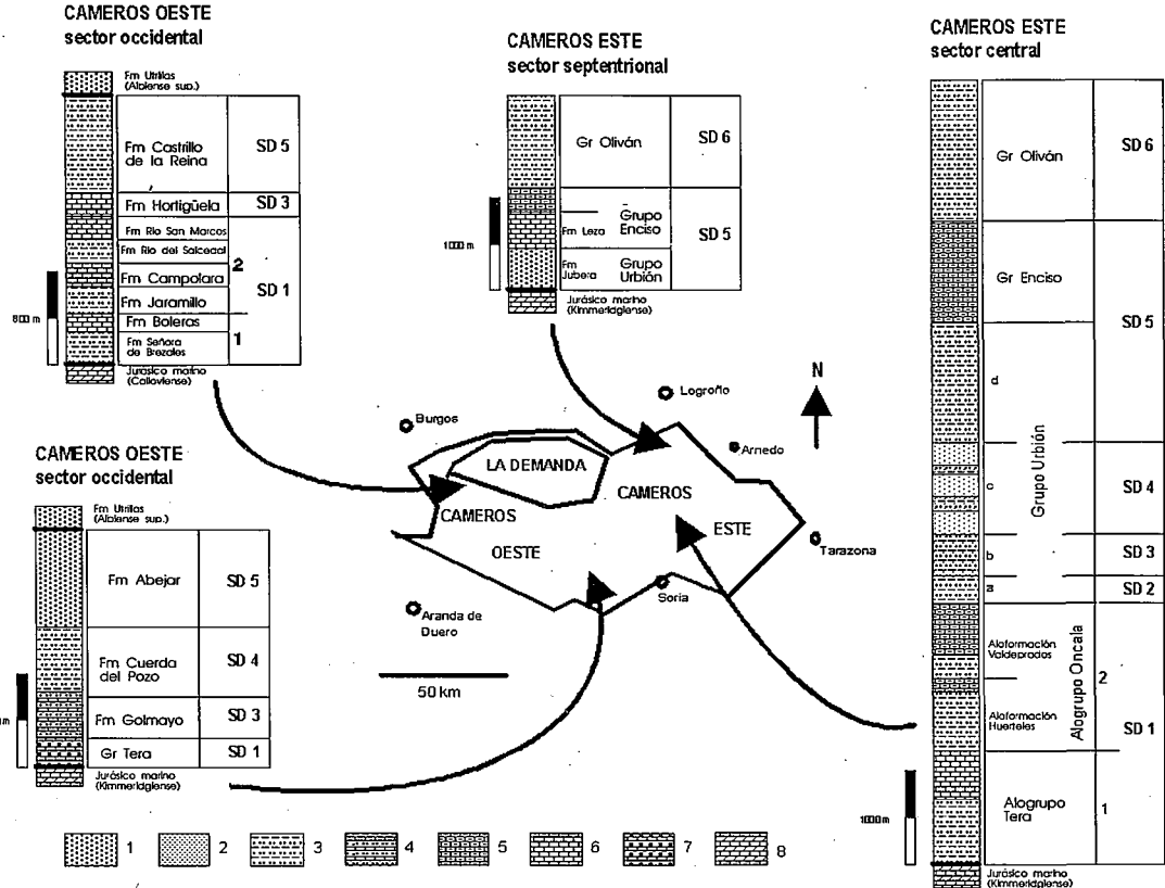
Figura 5.- a) Estratigrafía de la Cuenca de Los Cameros: Estratigrafía Secuencial del relleno de la cuenca. Secuencias Deposicionales (SD) y unidades estratigráficas: SD 1.1.- Alogrupo Tera (1). SD 1.2.- Alogrupo Oncala = Aloformación Huérteles (2) y Aloformación Valdeprados (3). SD 2.- Fms (4a) y Heterolítica inferior (5) del Gr Urbión; Fm Peñacoba (6). SD 3.- Fms (4b) y Cabretón (7) del Gr Urbión; Fm Galmayo (8); Fm (9); Fm Hortigüela (10). SD 4.- Fms (4c) y Heterolítica de transición (11) del Grupo Urbión; Fm Pantano (12). SD 5.- Fms (4d), Abejar (4e), (4f) y (4g) del Gr Urbión; Gr Enciso (13). SD 6.- Gr Oliván. Facies: siliciclásticas aluviales (punteado); carbonáticas lacustres (rayado vertical); mixtas (rayado vertical con punteado); carbonáticas con influencia marina (en blanco). La denominación de las unidades estratigráficas está basada en parte en: Tischer (1965, 1966), Platt (1989), Clemente y Alonso (1990), Salinas y Mas (1990), Gómez (1992) y Clemente et al. (1991). b) Estratigrafía de la Cuenca de Los Cameros: Sucesiones características en distintas zonas de la cuenca. Facies predominantes: 1.- areniscas, arenas y conglomerados; 2.- areniscas; 3.- lutitas y areniscas; 4.- Lutitas y areniscas con intercalaciones de calizas; 5.- Calizas, margas y arcillas lacustres (alguna incursión marina ocasional); 6.- calizas lacustres (alguna incursión marina ocasional); 7.- calizas lacustres y conglomerados aluviales; 8.- Jurásico marino (calizas y areniscas).
