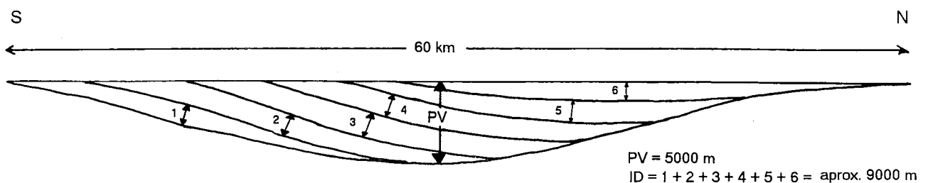
Figura 2.- Expresión simplificada del espesor de los depósitos que rellenan la cuenca. PV - potencia según un sondeo vertical hipotético; ID - incremento de depósito en el sentido del desplazamiento del depocentro.
