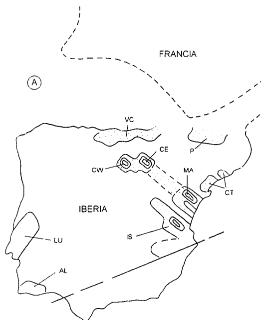
CUENCAS PRINCIPALES DEL RIFTING IBERICO
