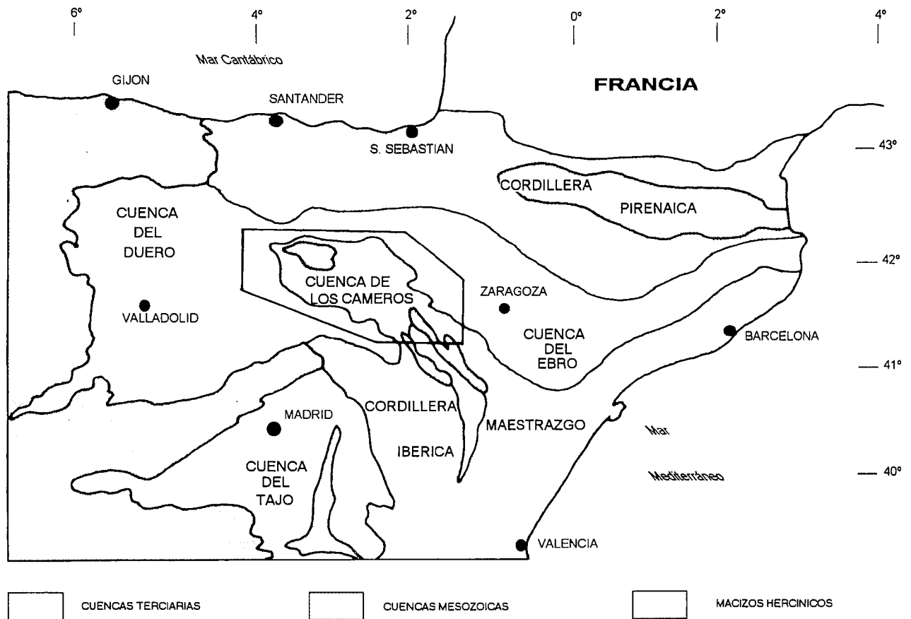
Figura 1.- Localización de la Cuenca de Los Cameros en el contexto de las Cuenchas Mesozoicas del NE de la Península Ibérica.
