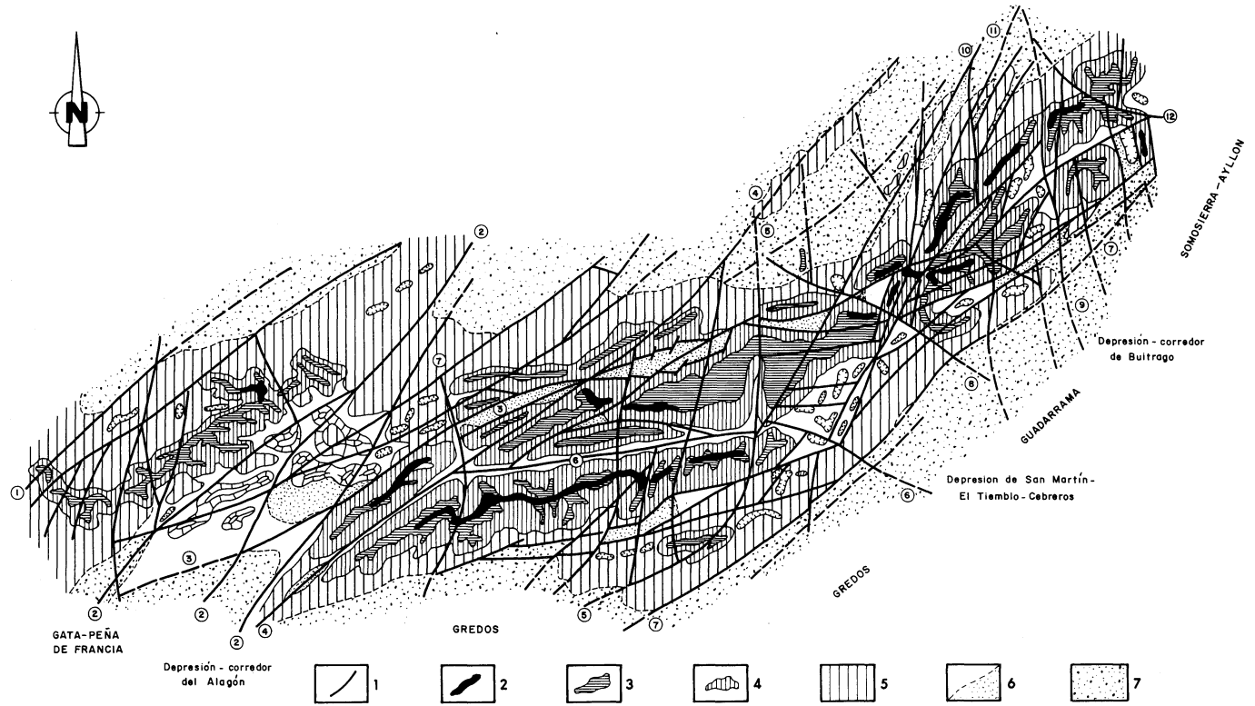
Fig. 1. Esquema de las principales alineaciones morfotectónicas del Sistema Central Español (según PEDRAZA, 1994).
