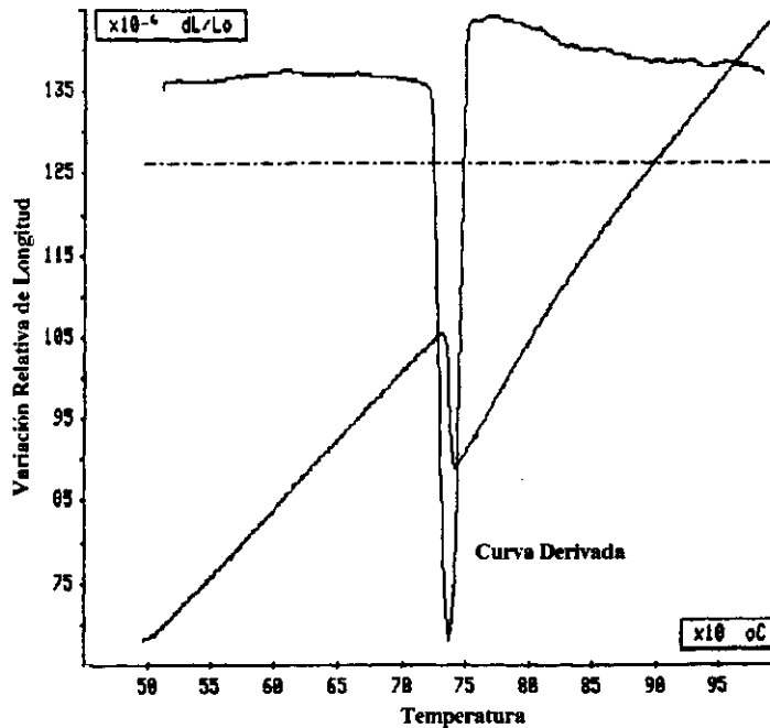
Figura 19.- Curva dilatométrica y curva derivada.
