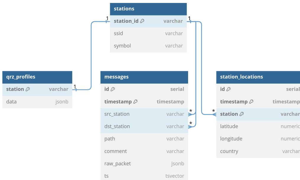
Figura 3.6: Estructura de la base de datos (elaboración propia).
