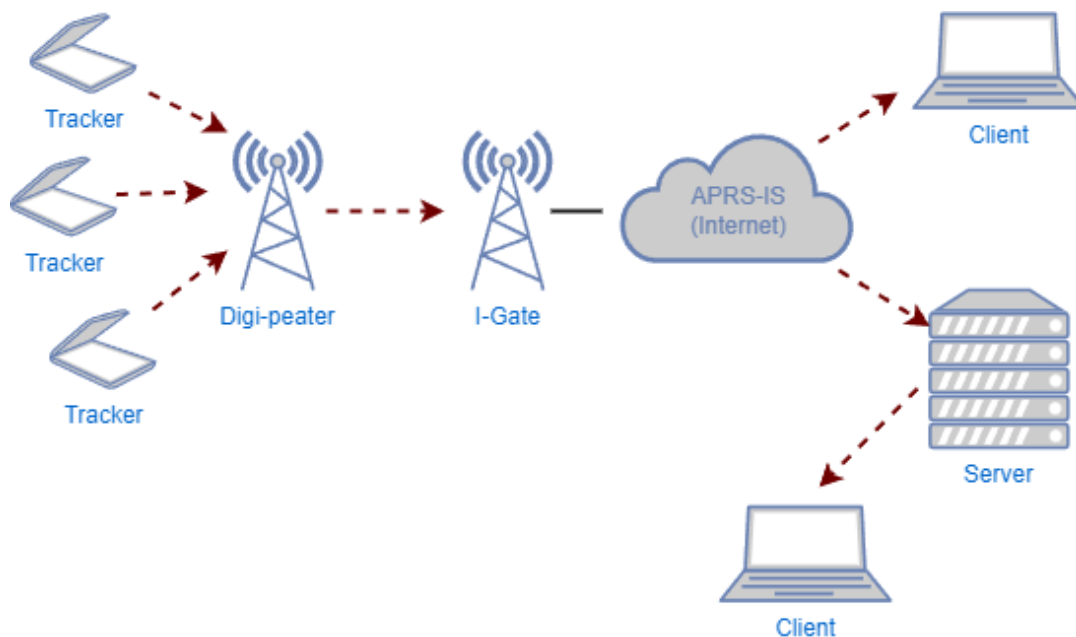
Figura 3.3: Infraestructura de la red APRS - APRS-IS (elaboración propia).
