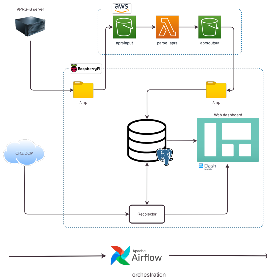
Figura 3.7: Flujo de datos en APRSINT (elaboración propia).
