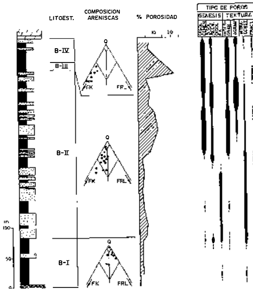
Fig. 2.—Porcentaje y tipo de porosidad (genético y textural) de las areniscas de facies Buntsandstein y Muschelkalk en la columna de Aranda del Moncayo. También se representa la composición de las mismas en relación a las unidades litoestratigráficas definidas.
