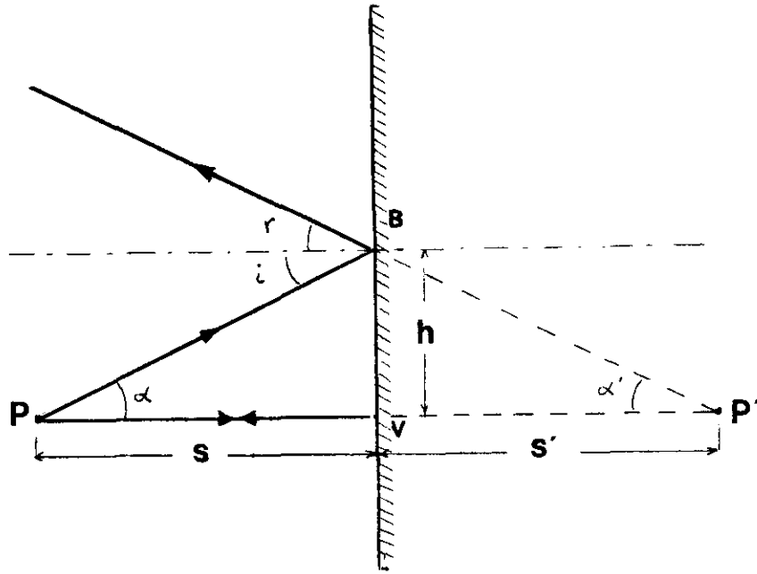
Fig.8.- Los rayos que divergen desde un punto P parecen divergir desde el punto P', después de la reflexión en una superficie plana
