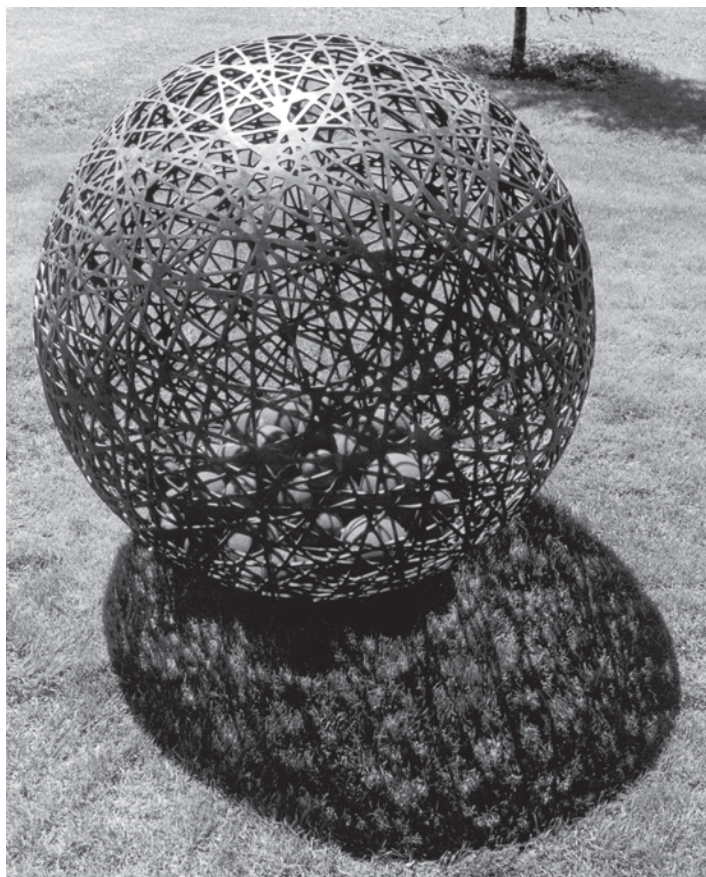
Imagen 12. Plutón.
