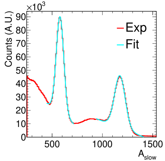
(b) ^{88}\text{Y}
