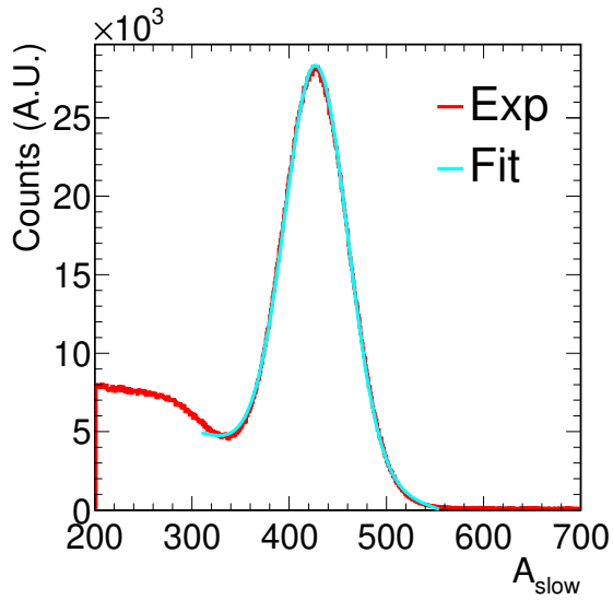
(a) ^{137}\text{Cs}
