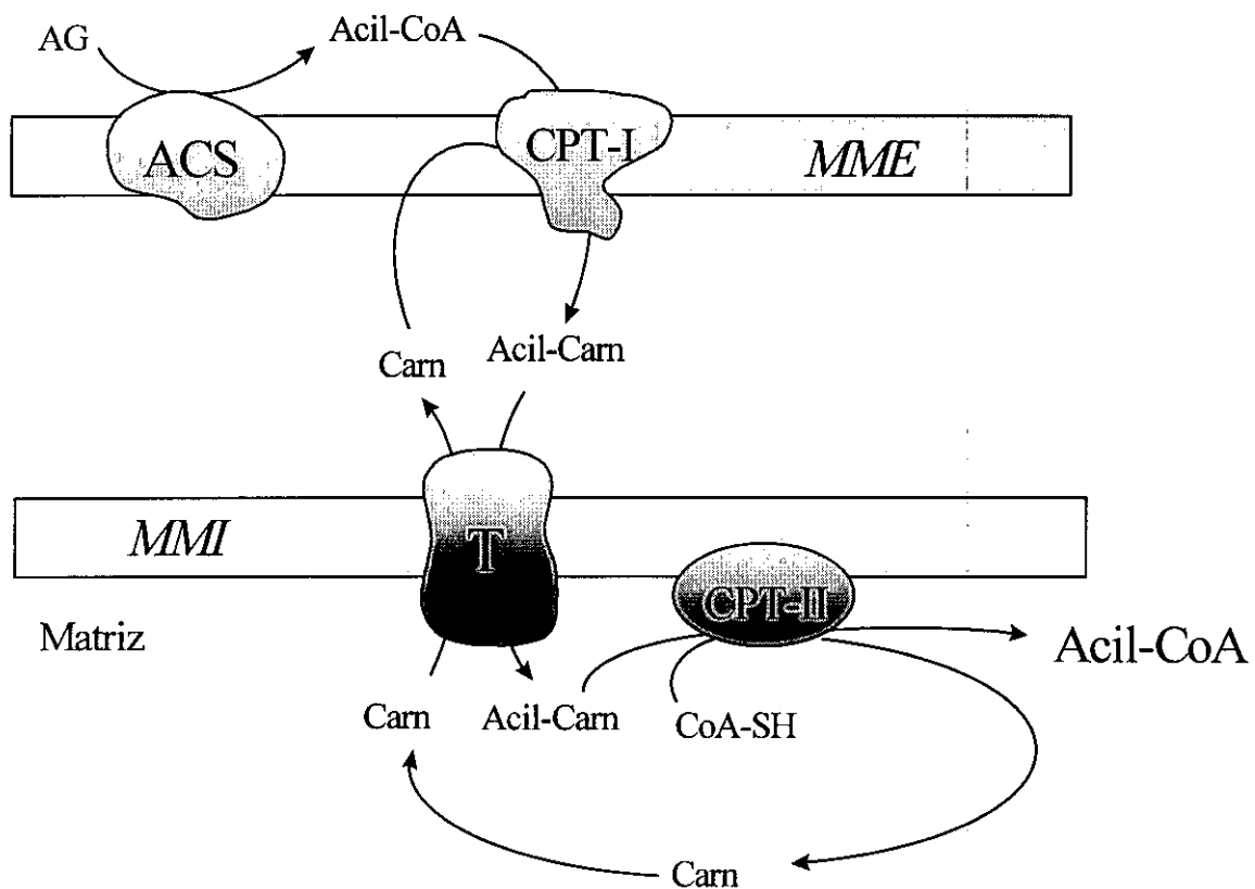
Figura 4. Traslocación de ácidos grasos a la matriz mitocondrial. Abreviaturas: ACS, acil-CoA sintetasa; AG, ácido graso; Carn, carnitina; MME, membrana mitocondrial externa; MMI, membrana mitocondrial interna; T, translocasa de carnitina:acilcarnitina
