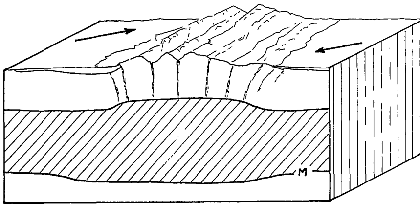
Fig. 2.—Modelo conceptual de la formación de los relieves del Sistema Central en el contexto de la deformación de la corteza en una zona de cizalla intraplaca. El rayado oblicuo representa la corteza inferior.
