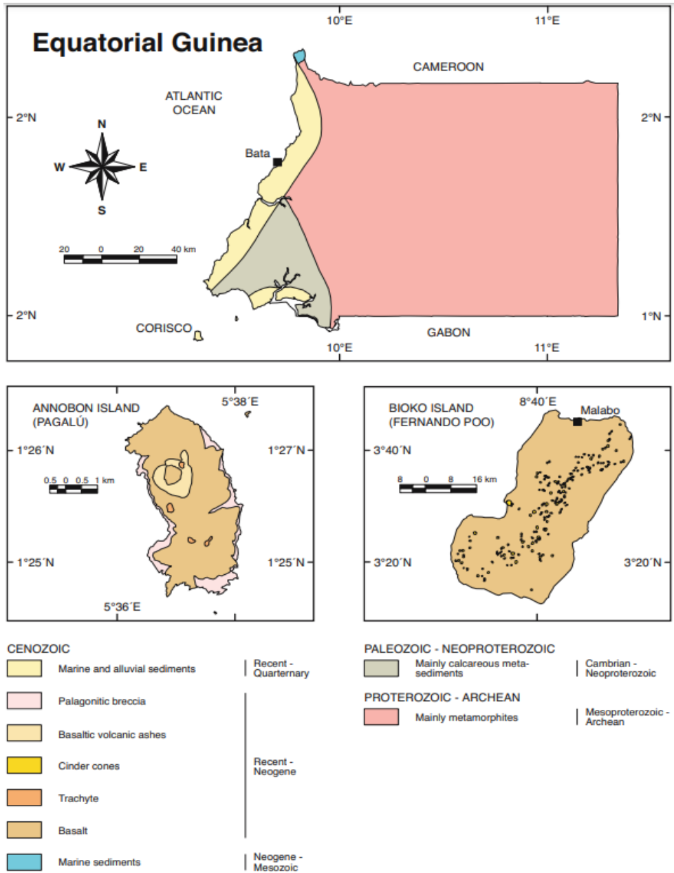
Figura 7: Vista general de la geología de Guinea Ecuatorial (Schlüter, 2006: 93)
