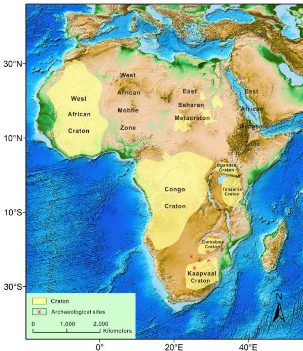
Figura 8: Mapa geológico de África con los Cratones Arcaicos (Sun et al. , 2016: 7)
