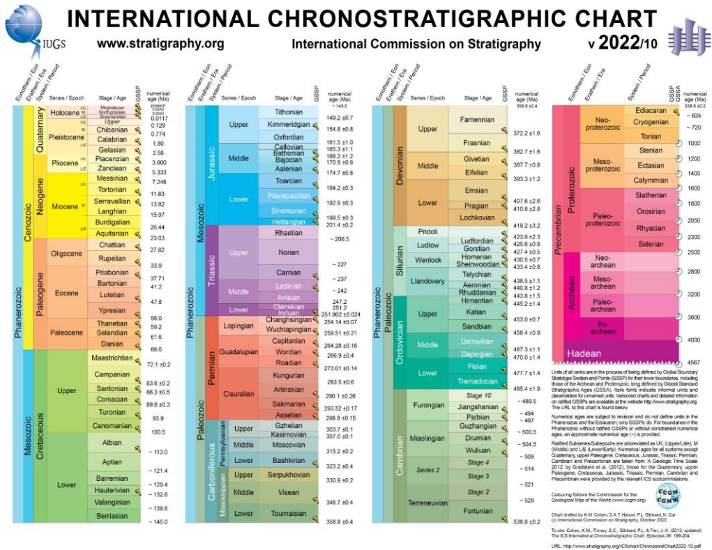
Figura 5: Tabla Cronoestratigráfica 2022 (fuente: https://stratigraphy.org/chart )
