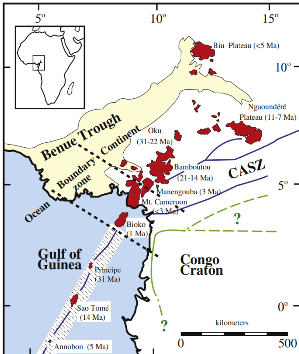
Figura 6: Línea Volcánica de Camerún (LCV) (Gannoun et al , 2015: 2)
