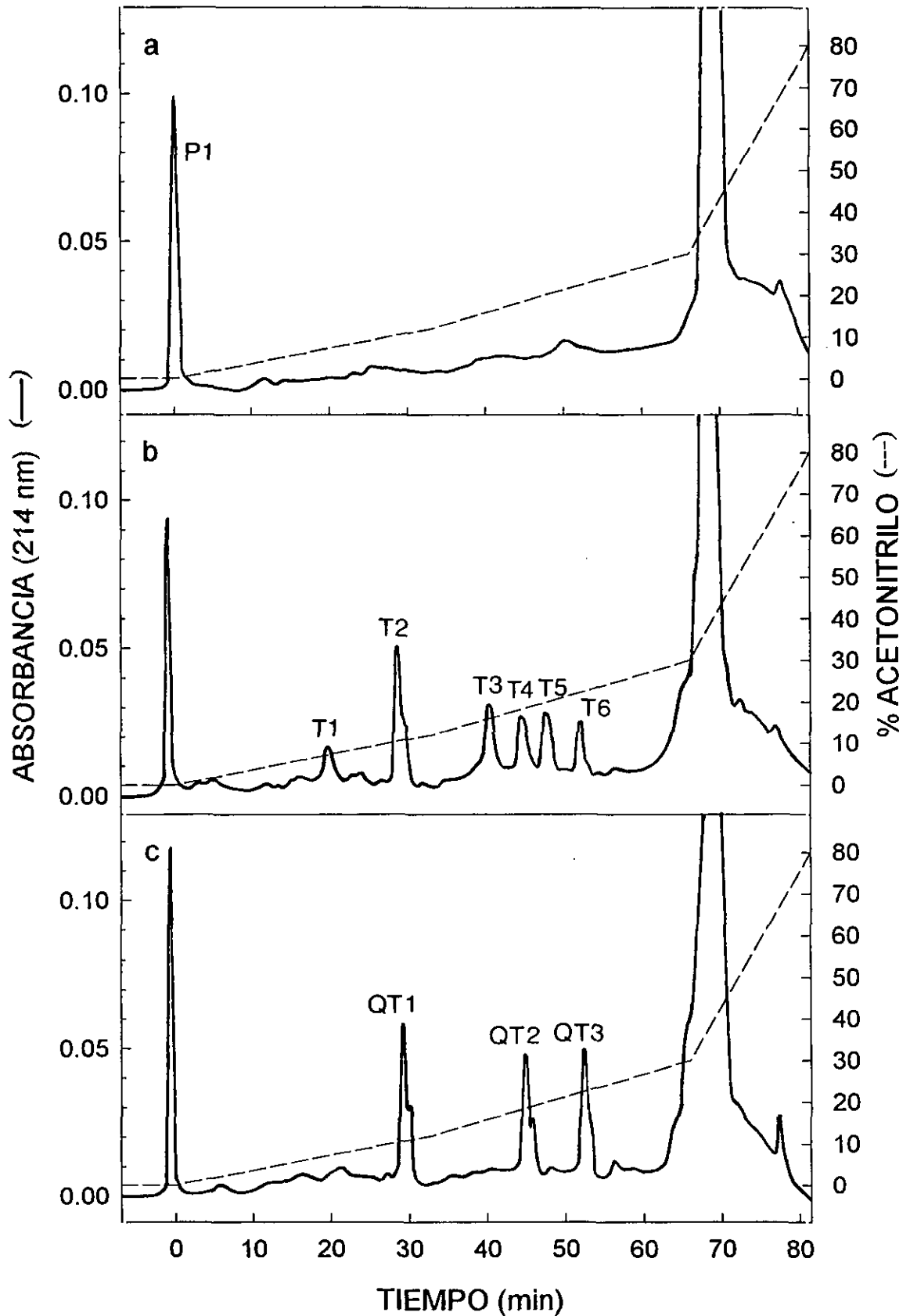
Figura 33. Perfiles de elución en RP-HPLC (columna Nucleosil C 18 ) de las digestiones de Sin a 1 con: (a) pepsina (pico P1); (b) tripsina (péptidos T1 a T6); (c) quimotripsina (péptidos QT1 a QT3).
