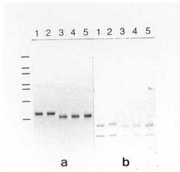
Figura 32. PAGE-SDS mostrando la resistencia a proteasas del alérgeno de la mostaza nativo. Líneas: 1, Sin a 1 sin digerir; 2, Sin a 1 tratado con pepsina; 3, Sin a 1 tratado con tripsina; 4, Sin a 1 tratado con quimotripsina; 5, Sin a 1 tratado simultáneamente con tripsina y quimotripsina. (a) Muestras sin reducir; (b) muestras reducidas con un 5% de \beta -mercaptoetanol.
