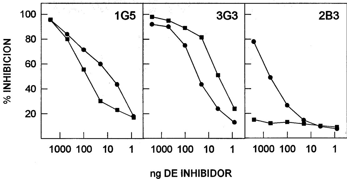
Figura 25. Curvas de inhibición de la unión de tres anticuerpos monoclonales a Sin a 1 adsorbido a poliestireno, utilizando como inhibidores (●) el alérgeno de mostaza nativo o (■) el recombinante. La desviación estándar en estos ensayos no supera en ningún caso el 5% del porcentaje de inhibición observado.
