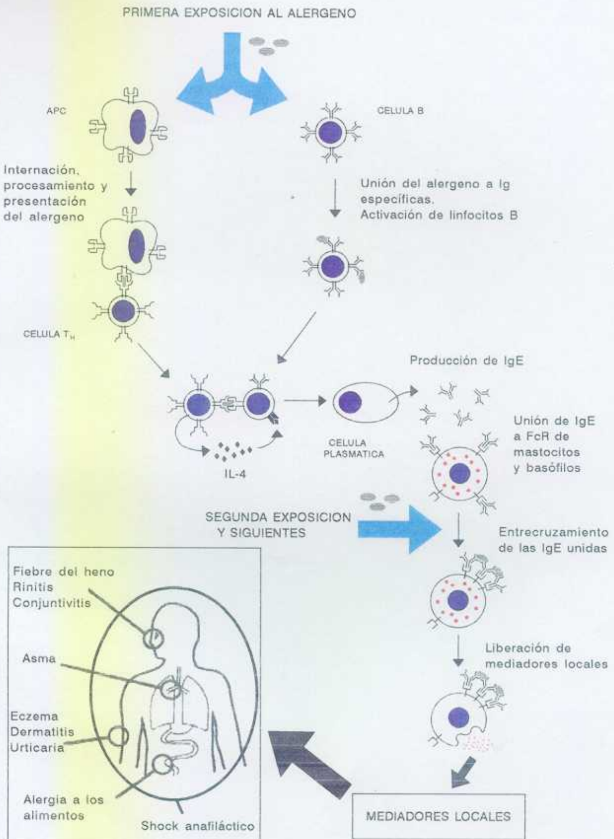
Figura 1. Secuencia de acontecimientos en la hipersensibilidad inmediata (ver texto). El contacto inicial con el alergeno conduce a la síntesis de grandes cantidades de IgE circulante. Estos anticuerpos se unen a la superficie de mastocitos o basófilos a través de los receptores de Fc de alta afinidad (FcR), lo que, en las siguientes exposiciones, desencadena la liberación de los mediadores químicos responsables de los síntomas clínicos de la alergia. APC, células presentadoras de antígeno; IL-4, interleucina-4.
