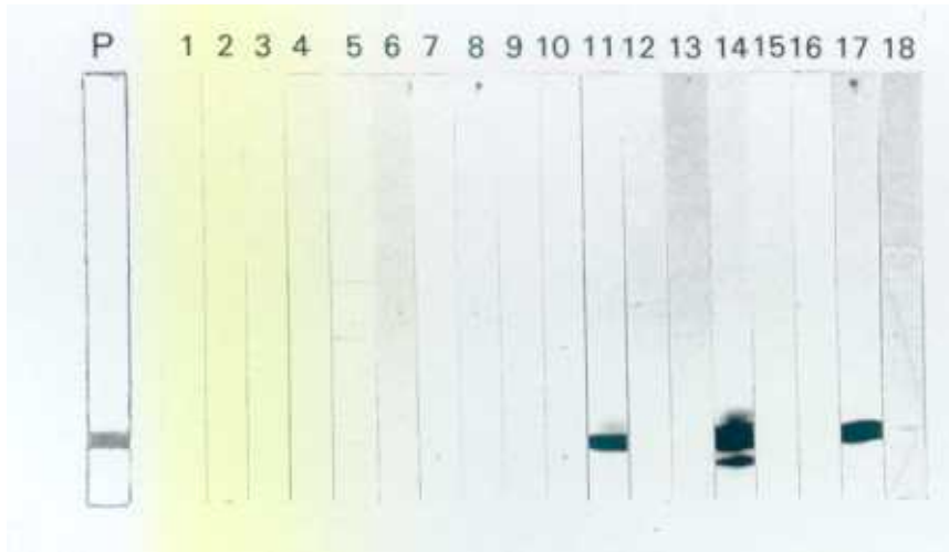
Figura 30. Inmunotransferencias del alérgeno de la mostaza tras PAGE-SDS en condiciones reductoras teñidas con 18 sueros de pacientes alérgicos a mostaza (tiras 1 a 18). La tira P corresponde a la misma muestra teñida con suero de conejo anti-Sin a 1.
