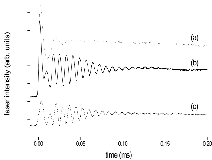
Figura 4.2: Medida experimental de: (a) intensidad total, (b) componente transmitida, (c) componente reflejada. Las curvas no están a escala debido a la distinta sensibilidad de los detectores.
