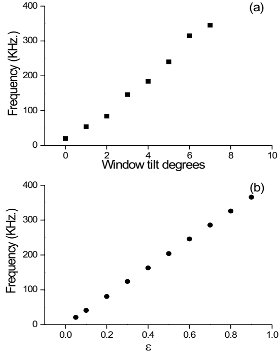
Figura 4.3: Comportamiento de la frecuencia de la oscilación de competición de polarización. (a) Experimental, en función de la inclinación de la ventana intracavidad ( V ), (b) Numérica, en función del parámetro de acoplo \epsilon .
