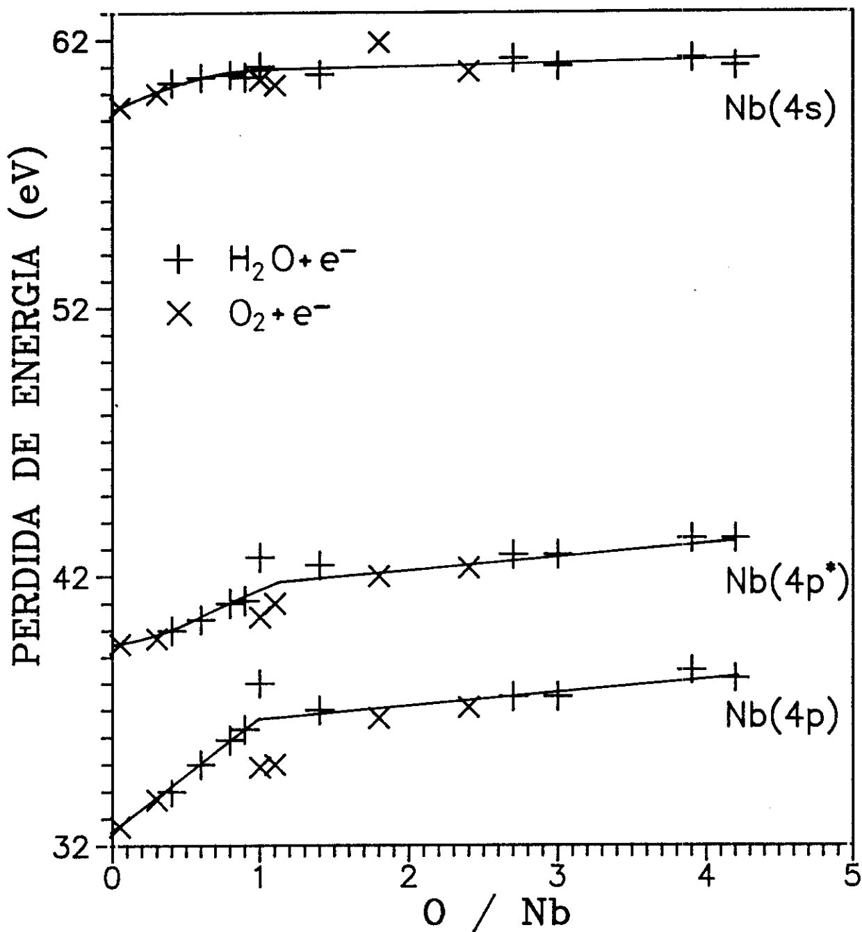
Fig. V.20.(b). Variación de las energías de las estructuras correspondientes a Nb(4p), Nb(4p*) y Nb(4s) en función de la relación O/Nb que presentaba la superficie con la exposición a H 2 O y O 2 y a distintas dosis de bombardeo electrónico.
