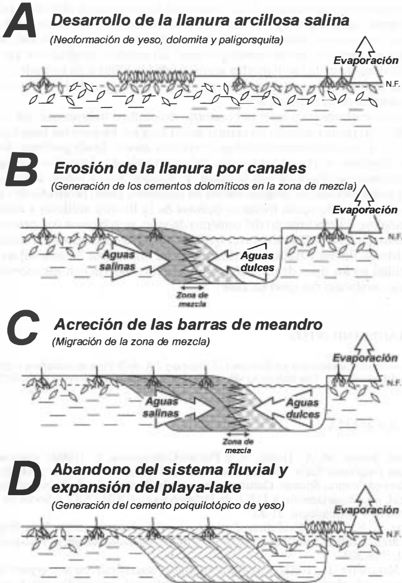
Fig. 11.—Etapas evolutivas de la sedimentación de los depósitos de ríos meandriformes asociados a ambientes de playa-lake y su relación con la generación de los cementos dolomítico y yesífero.
