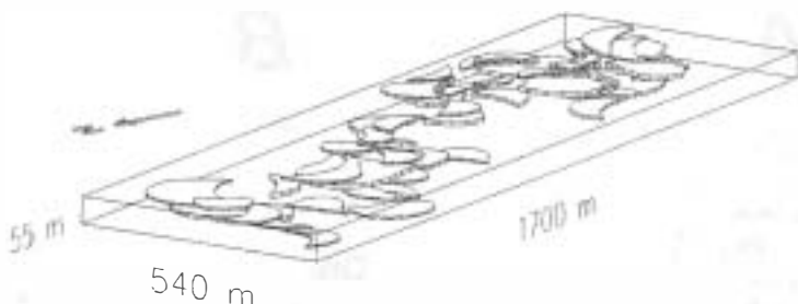
Fig. 6.—Reconstrucción tridimensional de los lóbulos de meandro del intervalo de «areniscas blancas». Cada lóbulo de meandro ha sido representado por un prisma recto con bases paralelas. La superficie de contacto vertical entre los prismas es sólo de un 20% de su superficie basal, predominando los cuerpos aislados.
