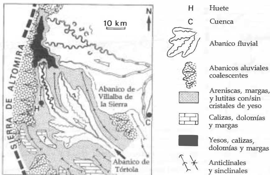
Fig. 3.—Reconstrucción paleogeográfica de la subunidad 2 (Ageniense) en la cuenca de Loranca. Fig. 3.—Paleogeographic reconstruction of the subunit 2 (Ageniense) in the Loranca Basin.
