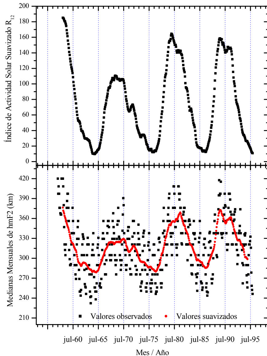
Fig. 3.3 Variaciones mensuales del índice R_{12} y Medianas mensuales de hmF2 observadas y suavizadas a las 12SLT para la Estación de Ekaterinburg (56.4°N ; 58.6°E).
