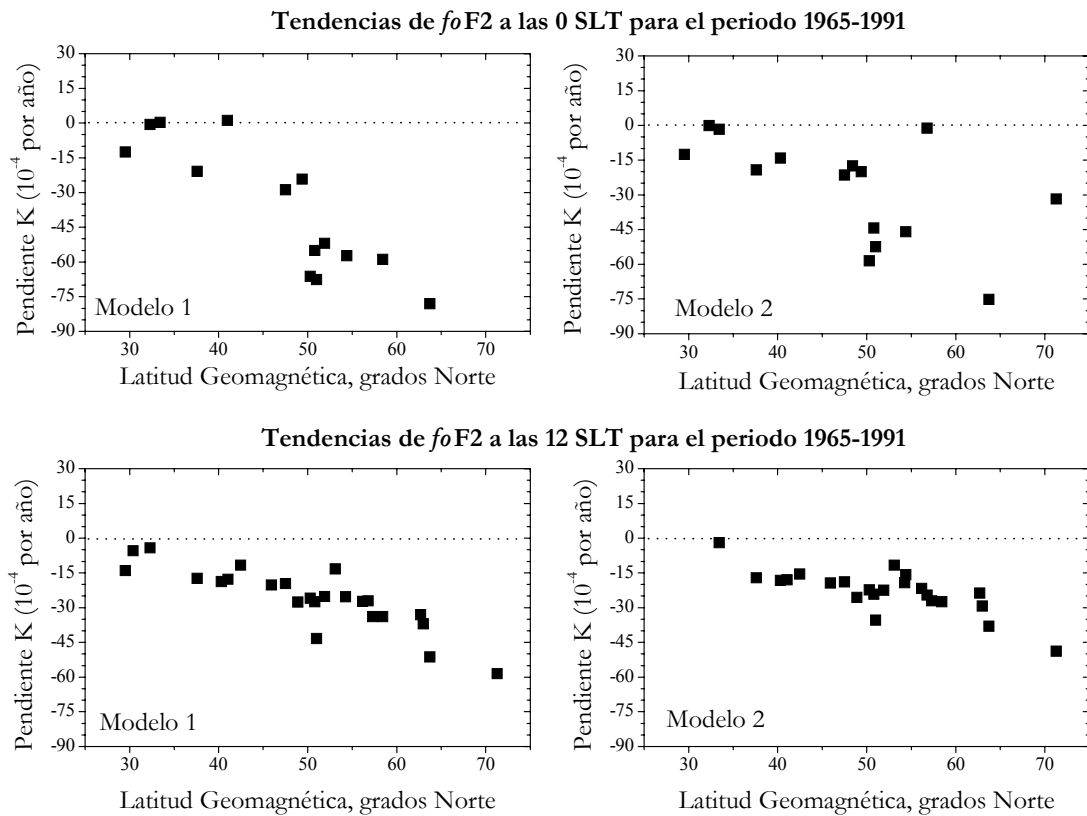
Fig. 3.14 Dependencia de las tendencias de f_oF2 con la latitud geomagnética a las 0 y 12 SLT cuando se consideran los años mínima actividad solar del periodo temporal 1965-1991. Los modelos 1 (regresión de f_oF2 con R_{12} ) y 2 (regresión de f_oF2 con R_{12} y Ap_{12} ) se han usado en la obtención de los resultados. Únicamente se muestran las Estaciones con tendencias significativas para un nivel de confianza del 90%.
