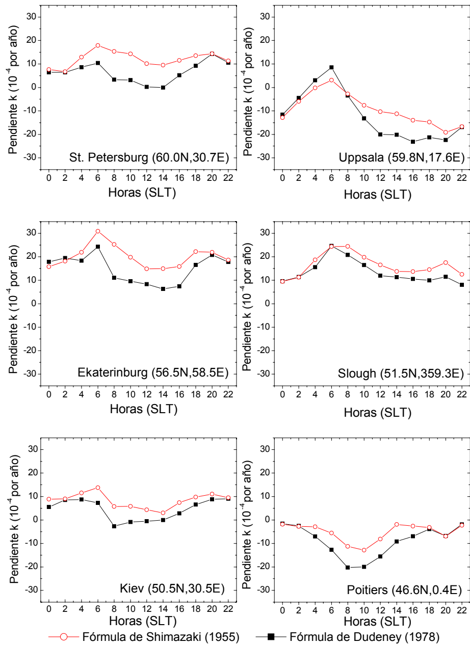
Fig. 3.12 Variaciones diurnas de las tendencias de hmF2 cuando se usan las fórmulas de Shimazaki (ecuación 3.1) y de Dudeney (ecuación 3.7) en la obtención de los valores de hmF2 .
