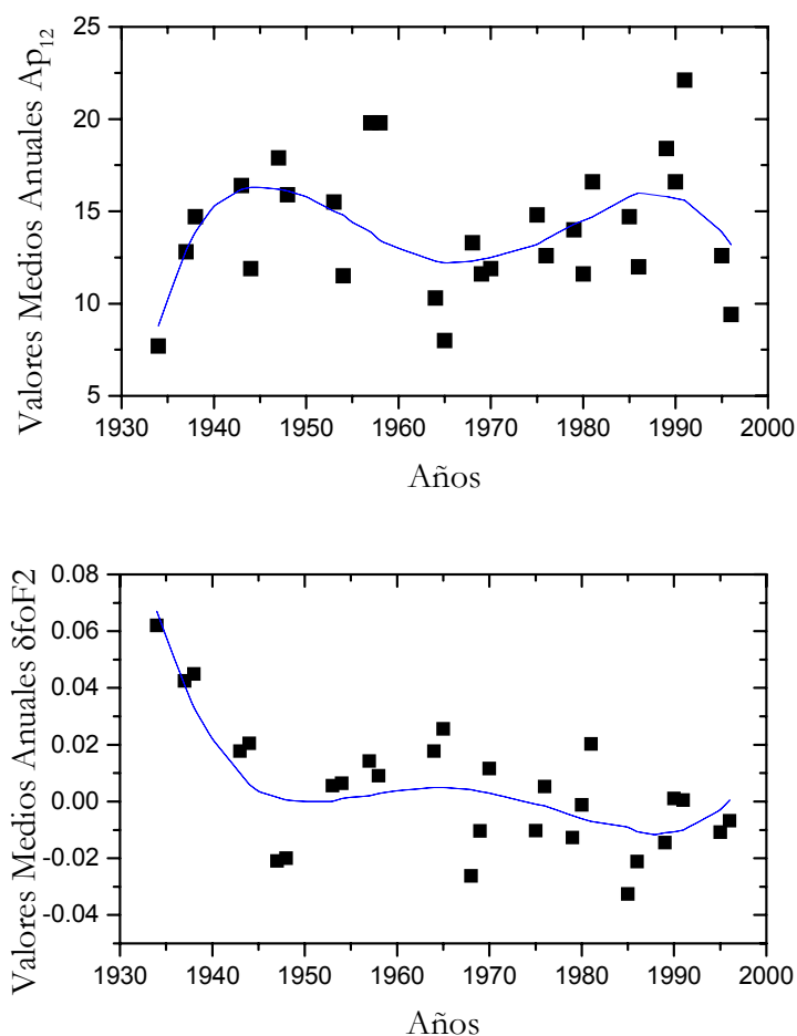
Fig. 3. Variaciones a largo-plazo de los valores medios anuales de Ap_{12} y \delta f_oF2 para la estación de Slough. La línea continua muestra un ajuste polinómico de cuarto grado. Únicamente se han considerado los años correspondientes a los máximos y mínimos de cada ciclo de actividad solar.
