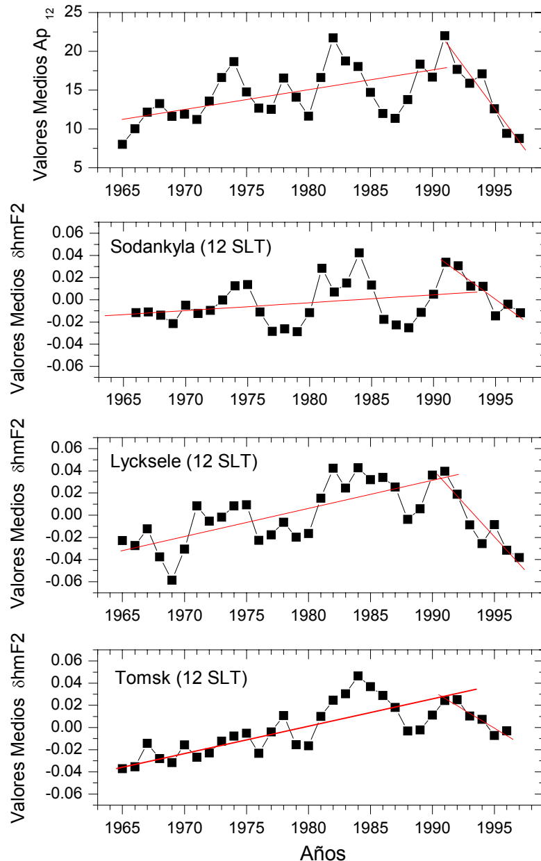
Fig. 3.23 Variaciones a largo-plazo de los valores medios anuales de A_p^{12} y \delta hmF2 para las Estaciones de Sodankyla, Lycksele y Tomsk. La líneas continuas representan ajustes lineales para los intervalos de tiempo anteriores y posteriores a 1991.
