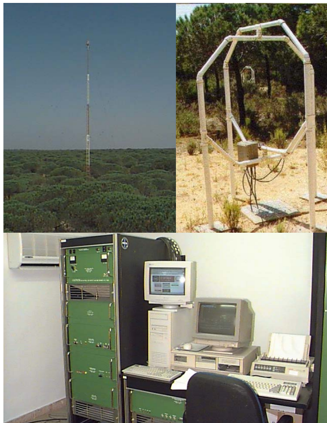
Fig. 2.6 Digisonda 256 de la Estación de Sondeos Atmosféricos “El Arenosillo” – INTA (37.1°N ; 6.7°W)
