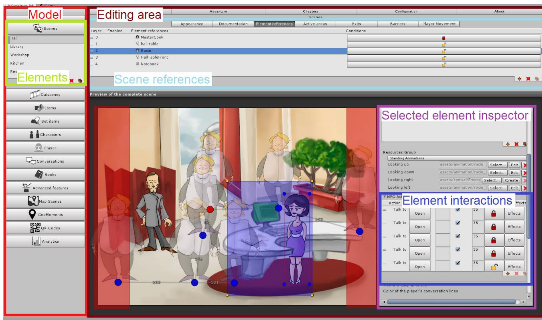
Figura 16. Nuevo editor de escenas de uAdventure con inspector.
