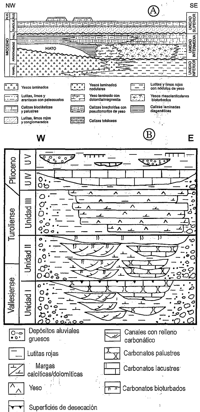
Figura 2.- A) Esquema litoestratigráfico del relleno sedimentario neógeno de la zona central de la Cuenca de Calatayud-Daroca (modificado de Sanz-Rubio, 1999). B) Esquema litoestratigráfico del relleno sedimentario neógeno de la zona norte de la Cuenca de Teruel (modificado de Alonso-Zarza y Calvo, 2000).
