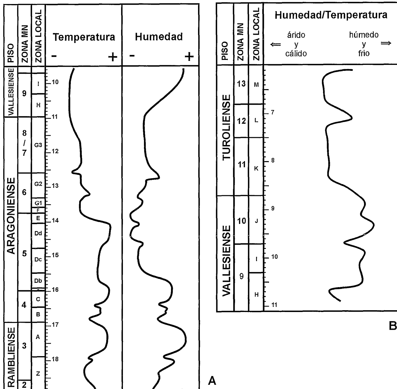
Figura 9.- Curvas de humedad y temperatura relativas basadas en asociaciones de faunas de micromamíferos. A) Resultados obtenidos a partir del registro Rambliesense-Vallesiense en el área de Villafeliche-Daroca (sector oriental de la Cuenca de Calatayud-Daroca) y Calamocha (modificado a partir de Meulen y Daams, 1992); B) Resultados obtenidos a partir del registro Vallesiense-Turoliense en el sector norte de la Cuenca de Teruel (Región de Teruel-Alfambra) y, en lo que se refiere al Vallesiense inferior, también en Daroca (modificado de Dam, 1997).
