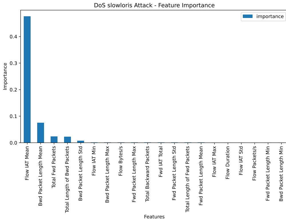
Figura B.7: Características de DoS slowloris
