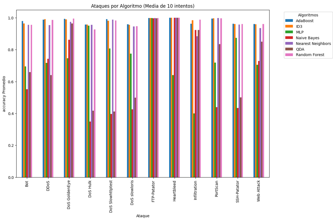
Figura C.1: Accuracy promedio por Ataque
