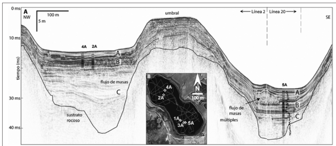
Figura 2. A. Perfil sísmico realizado en la laguna de Estanya con la división en las principales unidades sísmicas, localización de los sondeos y presencia de flujos de masas. B. Ortofoto de la cuenca lacustre con las líneas sísmicas medidas y la ubicación de los cinco puntos de sondeo (1A-5 A)
