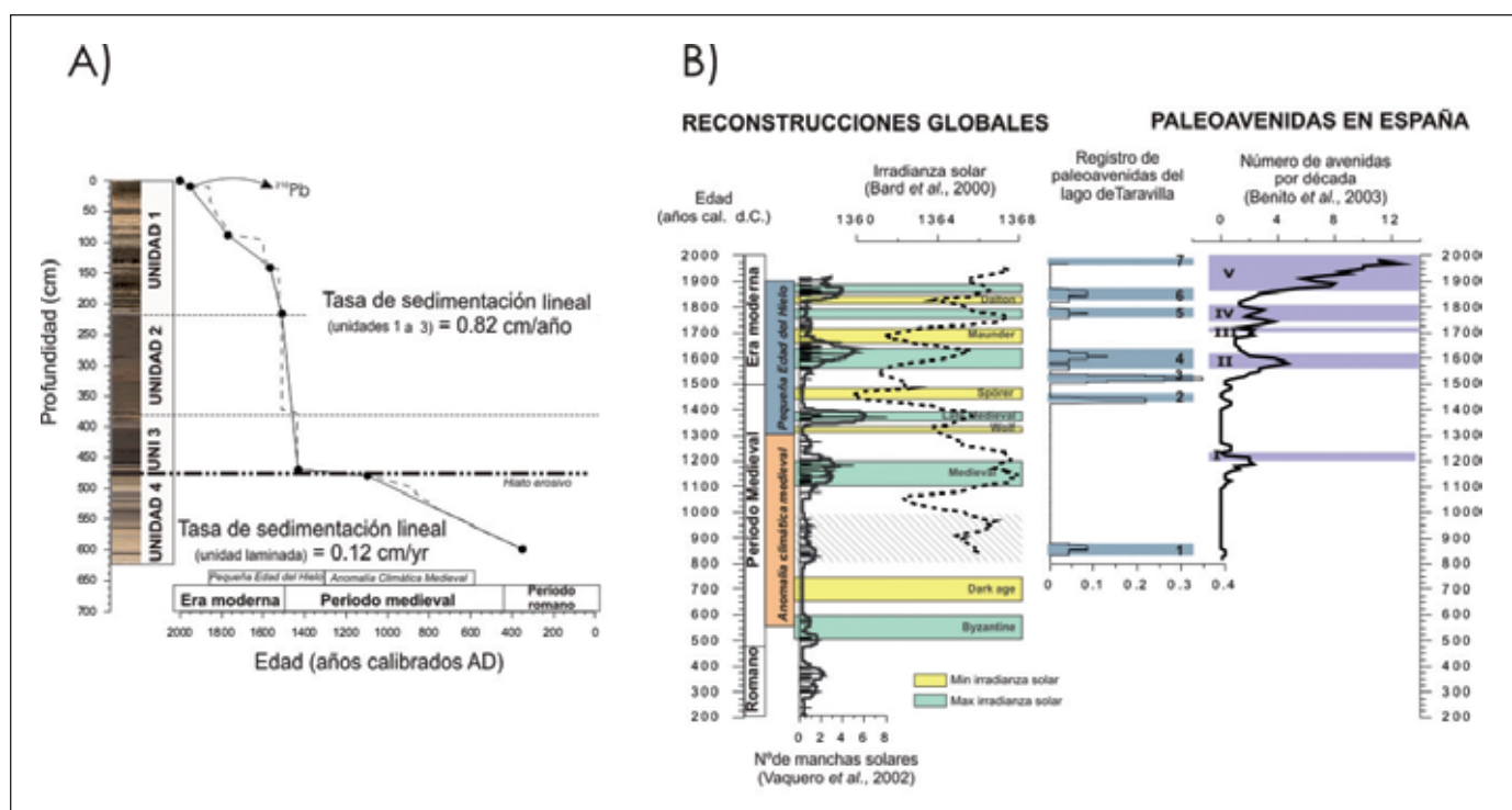
Figura 6. A. Modelo de edad de la secuencia sedimentaria recuperada en el Lago de Taravilla a partir de dataciones de ^{14}\text{C} y de ^{210}\text{Pb} . B. Comparación durante los últimos 2000 años de la radiación solar (representada aquí por el número de manchas solares de Vaquero et al. , 2002 y por la reconstrucción realizada por Bard et al. , 2000 a partir de isótopos de ^{14}\text{C} y de ^{10}\text{Be} con los resultados de la frecuencia de paleoavenidas obtenidos en el Lago de Taravilla y en el río Tago (Benito et al. , 2003) Figure 6. A. Age model based on ^{14}\text{C} and ^{210}\text{Pb} dates for the Taravilla sequence. B. Comparison of the last 2000 years of solar radiation (represented by the sun-spot numbers from Vaquero et al. , 2002 and by ^{14}\text{C} and ^{10}\text{Be} production from Bard et al. , 2000) and with flood frequency deduced from Taravilla Lake and Tago River records (Benito et al. , 2003)
