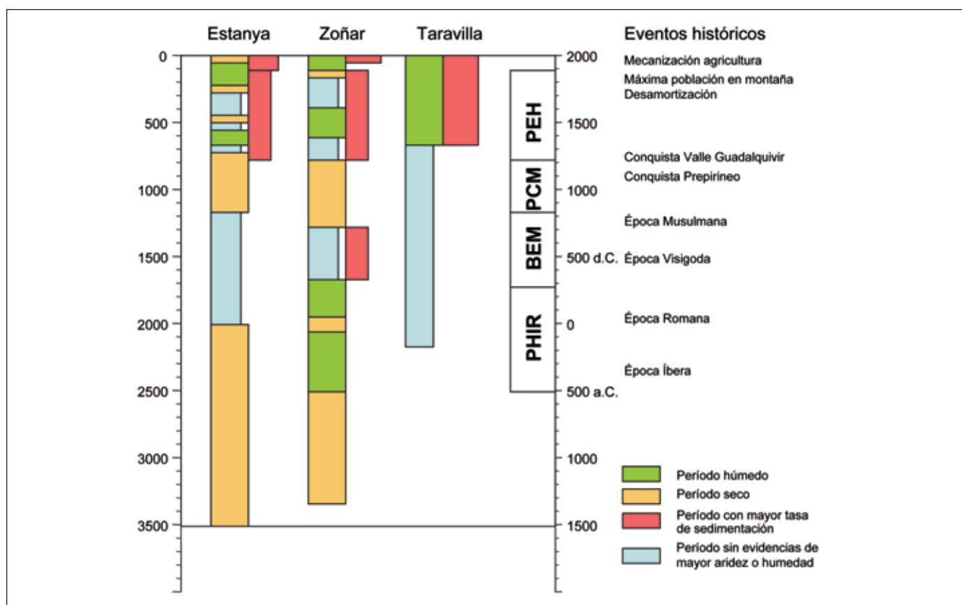
Figura 7. Principales fases húmedas y áridas reconstruidas en los tres lagos estudiados y periodos de mayor aporte de sedimentos clásicos durante los últimos 3000 años : PCM (Período Cálido Medieval), PEH (Pequeña Edad del Hielo), BEM (Baja Edad Media), PHIR (Periodo Húmedo Ibero Romano)
