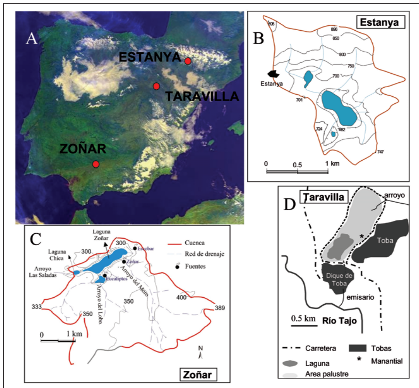
Figura 1. A. Localización de los lagos kársticos estudiados: Zoñar (Córdoba), Taravilla (Guadalajara) y Estanya (Huesca). Mapas de las cuencas vertientes a los lagos: B. La laguna de Estanya. C. La laguna de Zoñar. D. La laguna de Taravilla
