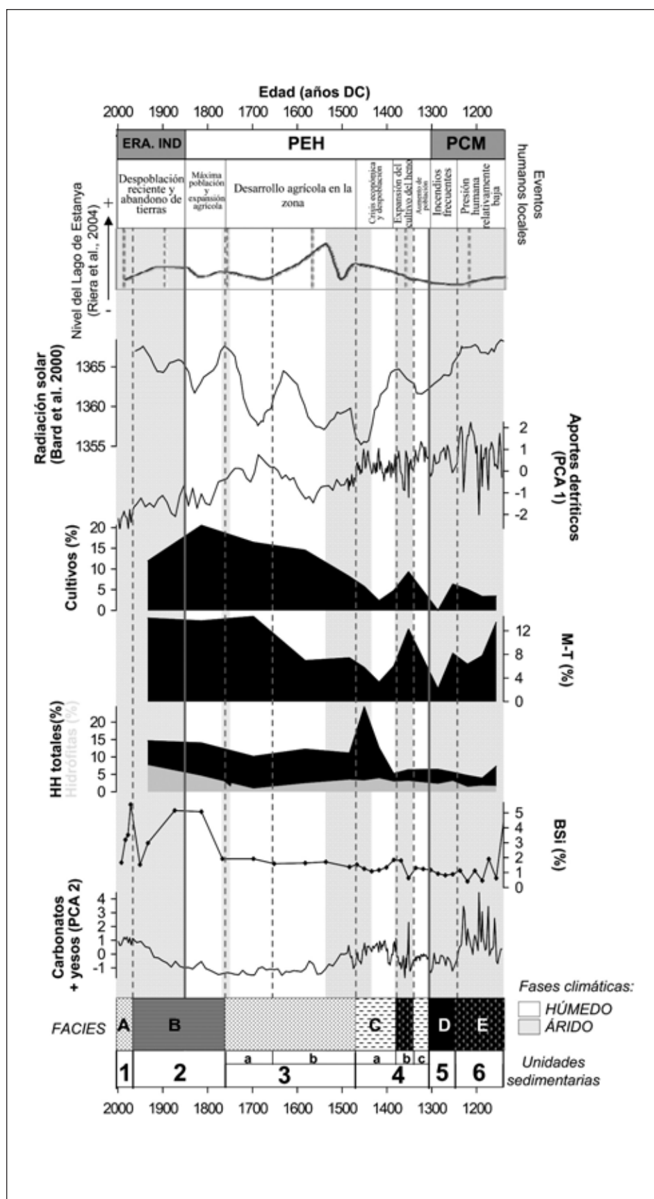
Figura 5. Resumen del registro paleoambiental de Estanya de los últimos 800 años. Incluye (de abajo a arriba): división en unidades sedimentarias, facies sedimentarias, contenido en carbonatos y yesos (deducido a partir del Análisis de Componentes Principales de los datos de geoquímica elemental de alta resolución), isótopos de materia orgánica \delta^{13}C_{org} silíce biogénica (BSi), contenido en polen de hidrofitas totales (HH, negro) y acuáticas (gris), MesoTermófitos (M-T) y cultivos, Aportes detríticos (deducido a partir del ACP de los datos de geoquímica elemental de alta resolución); comparados con la radiación solar en el hemisferio norte (Bard et al. , 2000), las variaciones en el nivel de Estanya deducidas por (Riera et al. , 2004), escala de eventos humanos locales en la región y principales fases climáticas de este período: PCM (Período Cálido Medieval), PEH (Pequeña Edad del Hielo). Leyenda de facies: A. Alternancia de limos grises y negros, masivos con materia orgánica; B. Limos versicolores finamente laminados, alternando: arcillas grises masivas, láminas marrones oscuras, masivas, ricas en materia orgánica y limos grises-marrones masivos; C. Limos grises oscuros y marrones laminados con materia orgánica; D. Arcillas limosas negras, masivas a débilmente laminadas; E. Alternancia de sapropel marrón, masivo a débilmente laminado con yeso nodular y en láminas blancas a amarillas con limos grises-oscuros, masivos con bioturbación y restos vegetales Figure 5. Synthesis of the paleoenvironmental record of Estanya for the last 800 years. From bottom to top: sedimentary units, sedimentary facies, carbonate and gypsum content (inferred from PCA analyses of high resolution geochemistry data set), organic matter isotopes \delta^{13}C_{org} biogenic silica (BSi), pollen content in total hydrophytophytes (HH, black) and aquatics (grey), mesothermophilous (M-T) and cultivars, clastic input (inferred from PCA analyses of high resolution geochemistry data set). Reconstructions are compared with solar radiation in the Northern Hemisphere (Bard et al. , 2000), Estanya lake level changes interpreted by Riera et al. , (2004), local and regional human events and main climate phases: PCM (Medieval Warm Period), PEH (Little Ice Age). Facies legend: A. Grey and black silts, massive with organic matter; B. Variegated finely laminated silts with massive grey clays, dark brown, massive, organic-matter- rich and massive grey-brown silts; C. Dark grey and brown, laminated, organic matter –rich silts; D. Black, massive to faintly laminated silty clays; E. Brown, massive to faintly laminated sapropels and nodular and laminated gypsum, with some dark grey silts with plant remains and bioturbation textures
