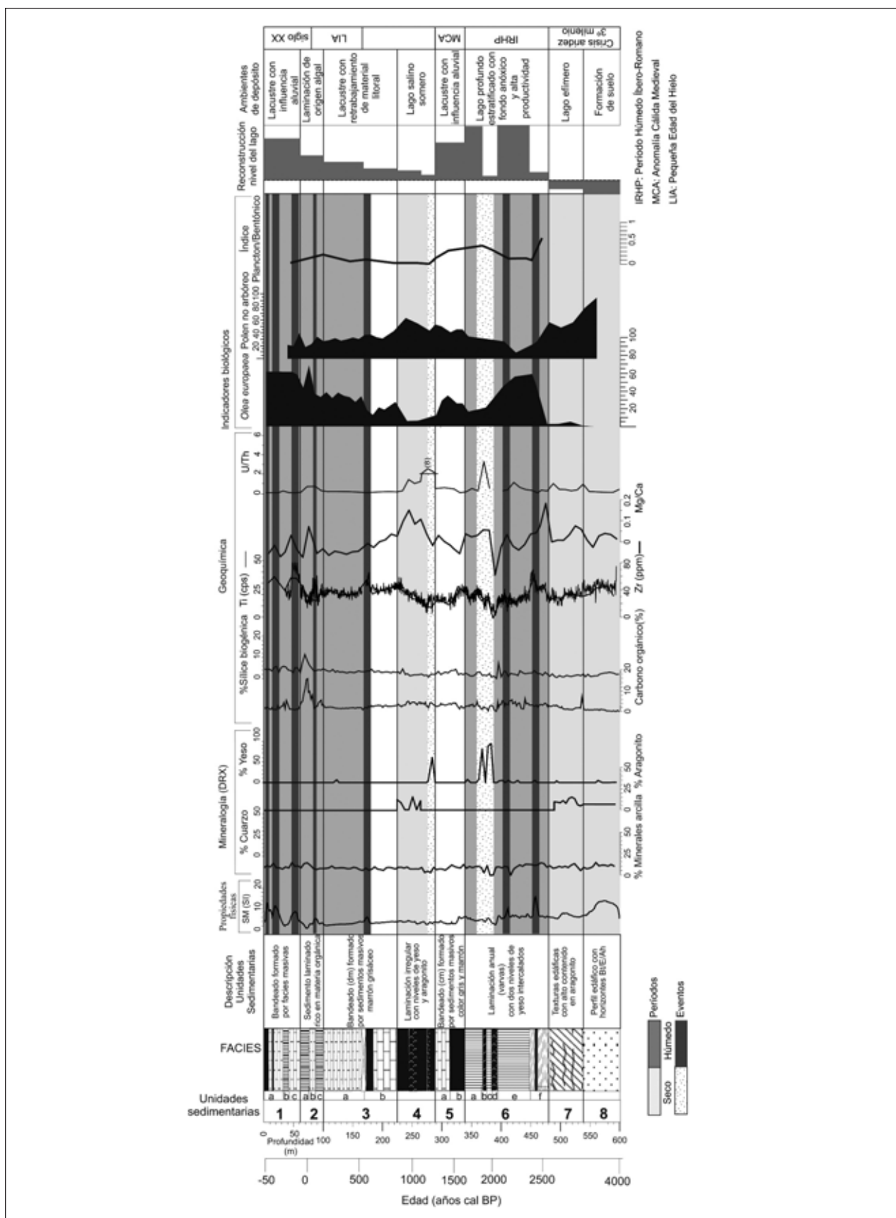
Figura 4. Resumen del registro de Zoñar. Descripción de facies sedimentarias, propiedades físicas, mineralogía, geoquímica, polen, reconstrucción de los ambientes de depósito y cronología Figure 4. Synthesis of the Zoñar record. Facies description, physical properties, mineralogy, geochemistry, pollen, reconstruction of depositional environments and chronology
