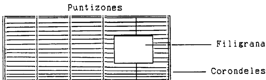
Gráfico 5. Formadora de papel.
