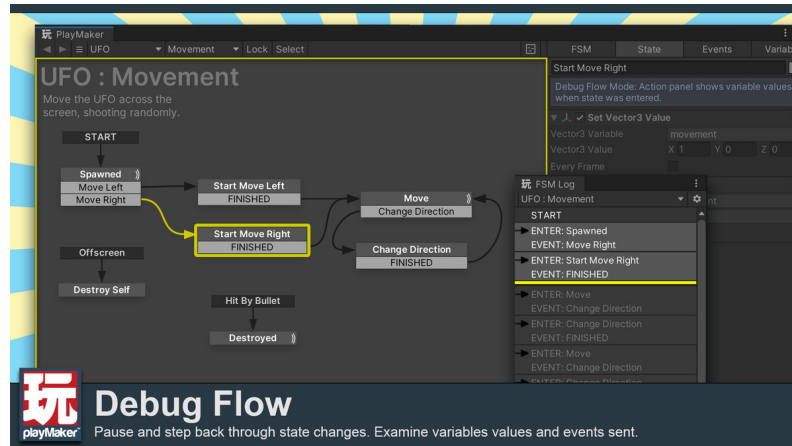
Figura 2.6: Ejemplo de uso de Play Maker
