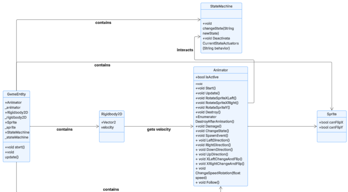
Figura 4.8: Diagrama UML del módulo de animación.
