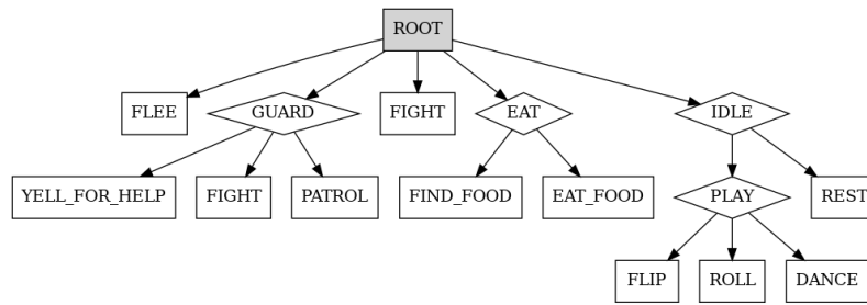
Figura 2.3: Ilustración de un árbol de comportamiento tomado del diseño del videojuego Spore , utilizado para modelar decisiones complejas en NPC's. 4
