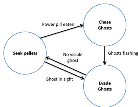
Figura 2.1: Comportamiento del jugador en Pac-Man , basado en una máquina de estados finita, extraído de Yannakakis y Togelius (2018).
