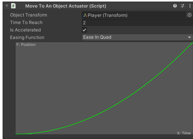
Figura 3.1: Easing Function que describe la variación de la posición de un objeto con el movimiento Move To An Object
