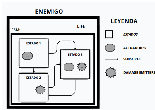
Figura 3.3: Ejemplo de estructura general de un enemigo basado en FSM.
