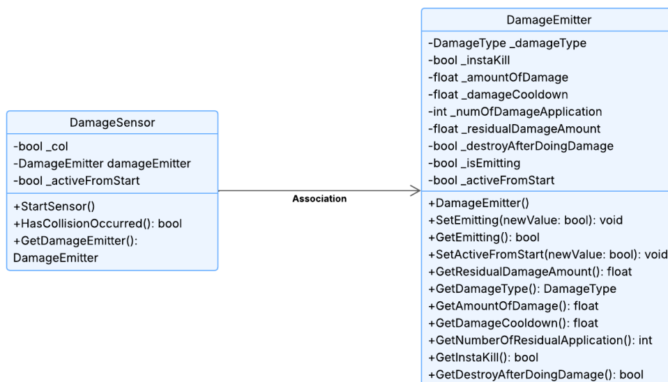
Figura 4.7: UML del apartado de daño de la herramienta
