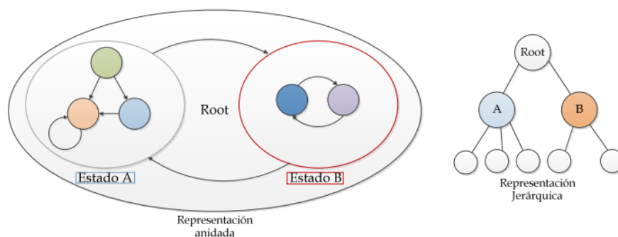
Figura 2.2: Ejemplo de maquinas de estado jerárquicas extraído de Borbor (2012).
