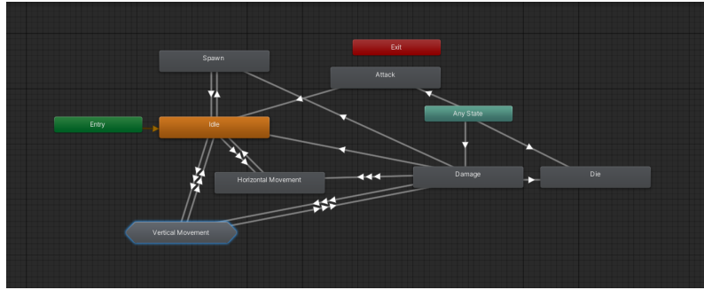
Figura 4.9: Animator Controller con sus estados y transiciones.
