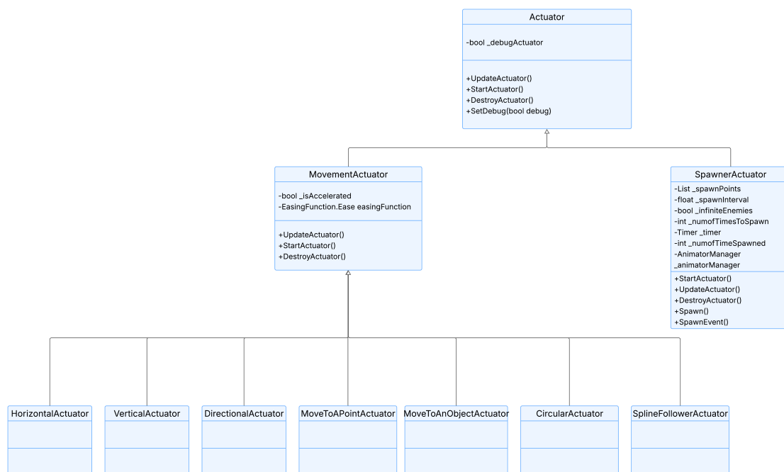
Figura 4.2: Diagrama UML del módulo Actuator.
