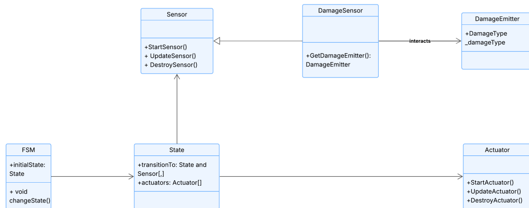
Figura 4.1: Diagrama UML de la composición.
