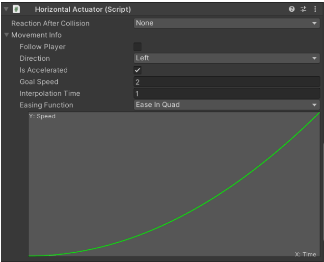
Figura 3.2: Easing Function que describe la variación de la velocidad de un objeto con el movimiento Horizontal
