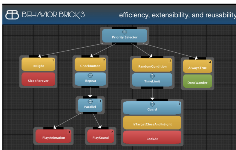
Figura 2.5: Ejemplo de uso de Behavior Bricks
