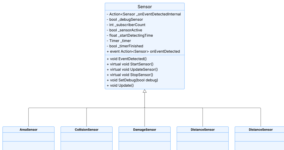
Figura 4.3: Diagrama UML del módulo de sensores.
