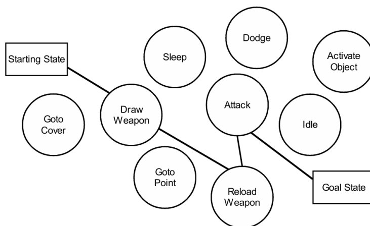
Figura 2.4: Ejemplo ilustrativo de GOAP donde el estado final es la eliminación de un enemigo.
