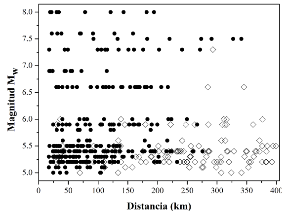
Fig. 2. Distribución de los datos con la magnitud M_w y la distancia más próxima al plano de ruptura. Los símbolos indican el tipo de dato disponible. Círculos: acelerogramas; rombos: registros de velocidad de banda ancha.
