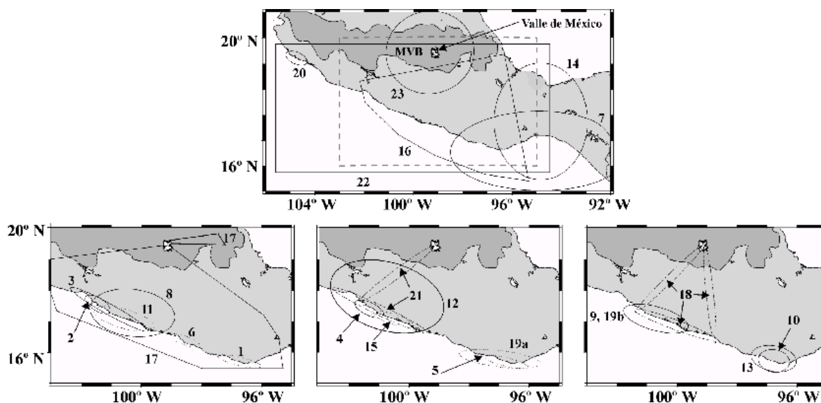
Figura 8: Región aproximada que abarcan los estudios de la Tabla 2 (los números se corresponden con los de la tabla). Mapa superior: trabajos regionales o que analizan áreas fuera del recuadro señalado en trazo discontinuo. Mapas inferiores: representación a menor escala de la zona contenida en dicho recuadro. En trazo discontinuo se muestran las áreas de aquellos estudios cuya extensión no se conoce con exactitud, y con rayas y puntos las líneas de atenuación de perfiles sísmicos.
