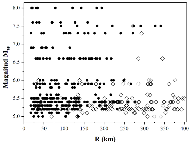
Fig. 2. Distribución de los datos con la magnitud M_w y la distancia más próxima al plano de ruptura. Los símbolos indican el tipo de datos disponible. Círculos: acelerogramas ( SM o BB ); rombos: registros de velocidad de BB .
