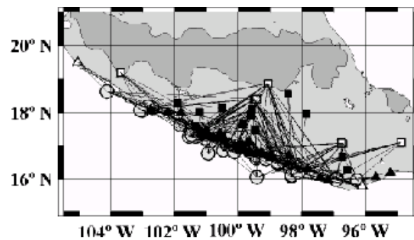
Fig. 3. Epicentros de los terremotos interplaca (círculos), estaciones (triángulos y cuadrados) y trayectorias utilizados en este Capítulo. Los símbolos coinciden con los de la Figura 1.
