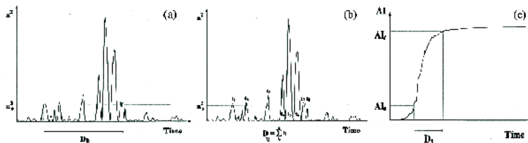
Figura 2: Ilustración de la definición genérica de la: (a) duración acotada, D_b ; (b) duración uniforme, D_u ; (c) duración significativa, D_s . En (a) y (b) se representa la historia temporal de la aceleración cuadrática; en (c) se representa el diagrama de Husid ( I_A frente al tiempo). (Modificado de Bommer y Martínez-Pereira, 1999)
