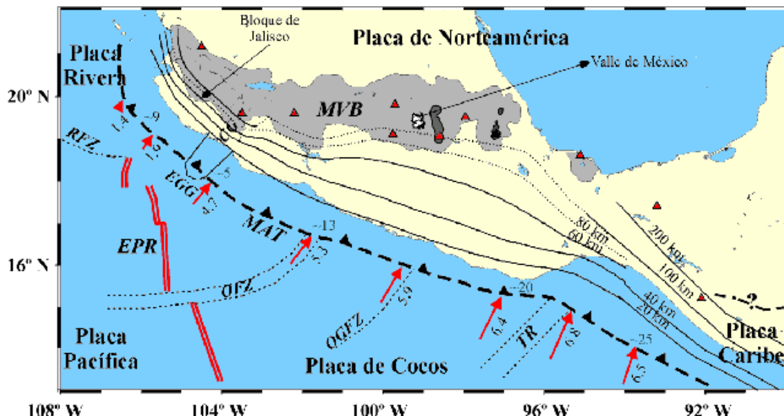
Figura 3: Sismotectónica del centro de México. Se marca la ubicación de la EPR (trazo rojo) y la MAT (trazo discontinuo grueso). Las flechas y números a lo largo de la MAT indican el sentido y velocidad de convergencia relativa (en cm/año), supuesta NOAM estática (DeMets et al. , 1994). También se señala la edad (en m.a.) de la litosfera oceánica en la MAT (Singh y Mortera, 1991). En trazo fino se delimitan otros rasgos tectónicos referidos en el texto. Las isobatas del slab se muestran en línea continua si están bien definidas por la sismicidad, y punteadas cuando se han inferido (Singh y Mortera, 1991; Pardo y Suárez, 1995). Triángulos rojos: volcanes activos. (Modificado de Kostoglodov y Pacheco, 1999)
