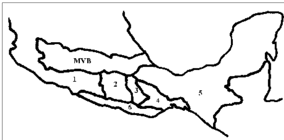
Figura 2: Terrenos tectonoestratigráficos de la zona centro-sur de México según Campa y Coney (1983). 1: Terreno Guerrero; 2: Terreno Mixteco; 3: Terreno Oaxaca; 4: Terreno Juárez; 5: Terreno Maya; 6: Complejo Xolapa. ( MVB : Cinturón Volcánico Mexicano)
