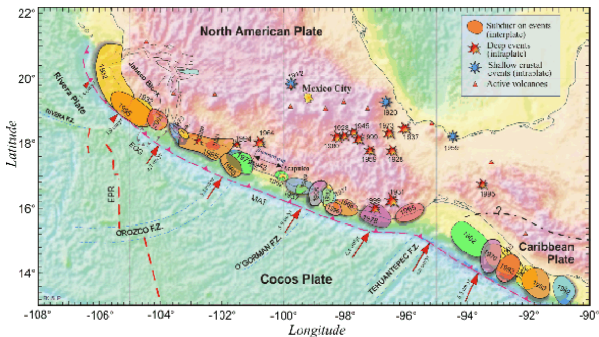
Figura 5: Grandes terremotos interplaca e intraslab del siglo XX en el centro de México. Se muestran las áreas de ruptura de los mayores eventos interplaca, inferidas a partir del área de réplicas, así como la localización de los eventos intraslab más notables (estrellas rojas). Las estrellas azules representan los grandes sismos corticales intraplaca. (Kostoglodov y Pacheco, 1999).
