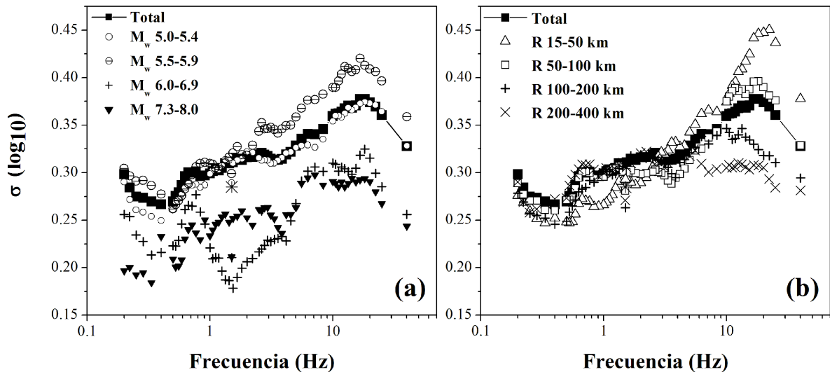
Fig. 6. (a) Variabilidad aleatoria (desviación estándar de los residuos en \log_{10} ) de la componente horizontal de la estimación del movimiento para la PSA y la PGA (representada a 40 Hz). La curva continua y los cuadrados negros simbolizan los resultados para todo el conjunto de datos. El resto de símbolos muestra la variabilidad para diferentes intervalos de magnitud. (b) Igual que en (a), pero ahora los distintos símbolos representan la variabilidad para diferentes intervalos de distancia. En ambos casos la variabilidad de la PGV se ha dibujado arbitrariamente a 1.5 Hz, y para el conjunto completo de los datos se denota por una estrella.
