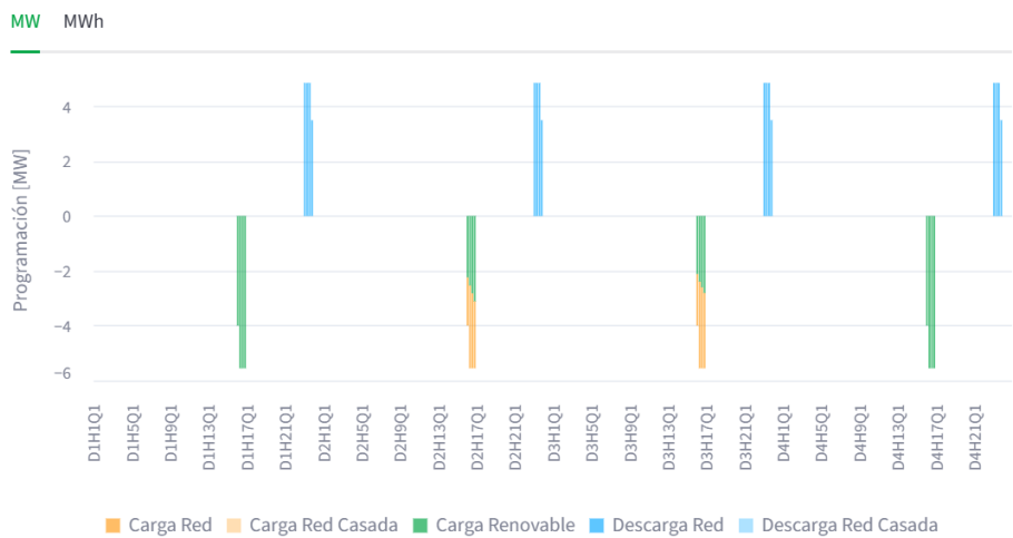
Figura 7.9: Programa de la topología híbrida con prioridad de carga de generación, en donde la batería no puede cargar hasta agotar el recurso de generación. Se observa como, aunque la batería quiera cargar de la red por la existencia de precios negativos beneficiosos, no es capaz de hacerlo.
