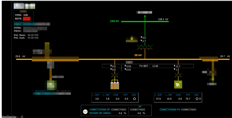
Figura 3.11: Visualización industrial de las señales de una instalación.
