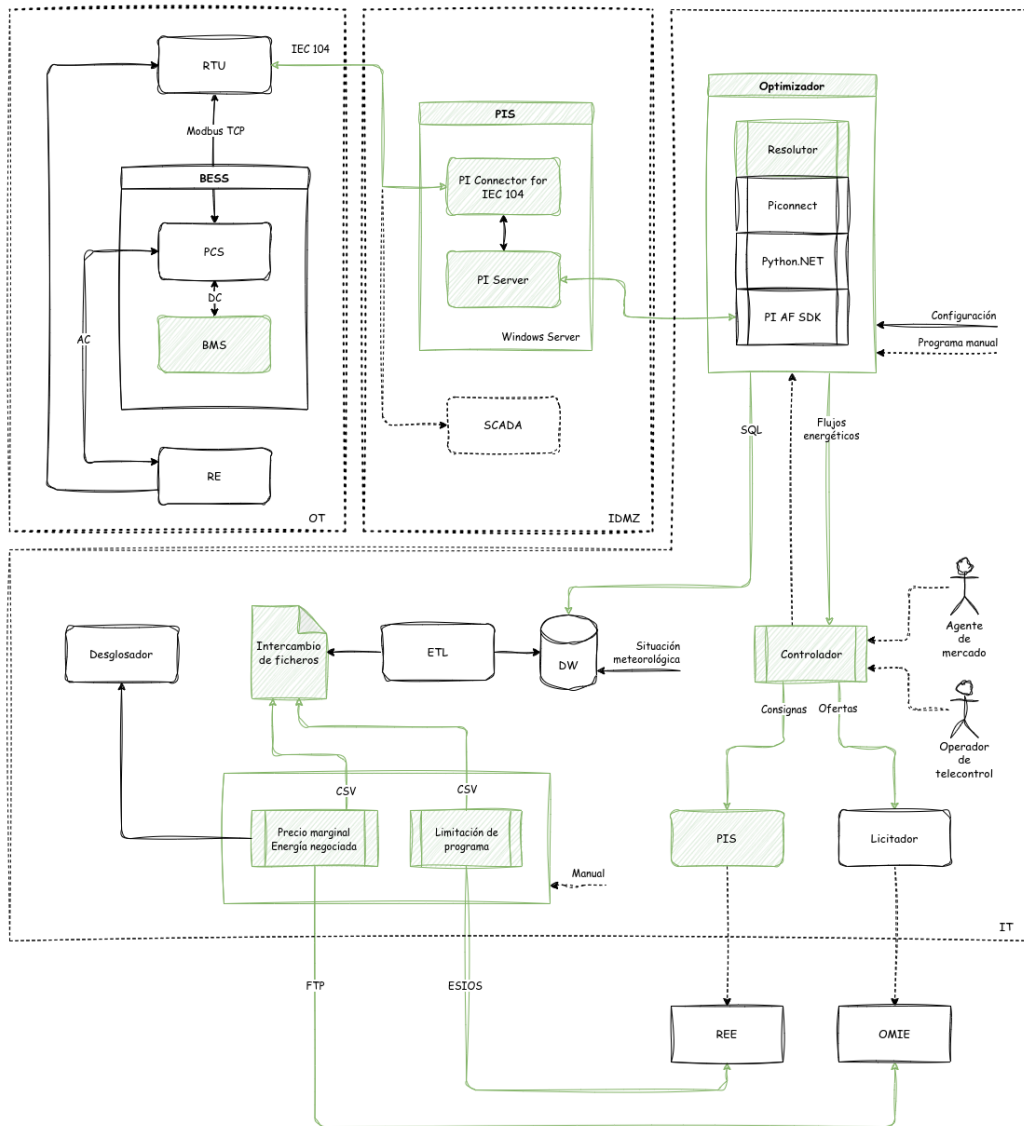
Figura 8.1: Arquitectura del flujo de información del sistema, diferenciando los elementos pertinentes al proyecto. En términos generales, los datos de las señales de los activos son obtenidos a través de la comunicación del PIS con la red operativa, mientras que la información de mercado es extraída de las instituciones regulatorias por tareas temporizadas y depositada en ficheros a insertar en el DW . El optimizador consulta las dos fuentes según la sesión de mercado y calcula los flujos de energía óptimos a realizar por los activos energéticos. Con ellos, el controlador los transforma en consignas mandadas de vuelta al PIS y ofertas a licitar. A su vez, los agentes de mercado y operadores de telecontrol son capaces de interactuar con el sistema a través del cuadro de mandos, informando al optimizador de las operaciones a realizar.
