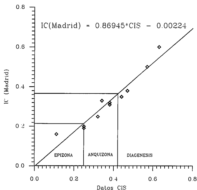
Figura 3.- Recta de calibración utilizando los datos de cristalinidad de los patrones CIS (Warr y Rice, 1994) y los medios en el difractómetro del Departamento de Cristalografía y Mineralogía de la U.C.M.
