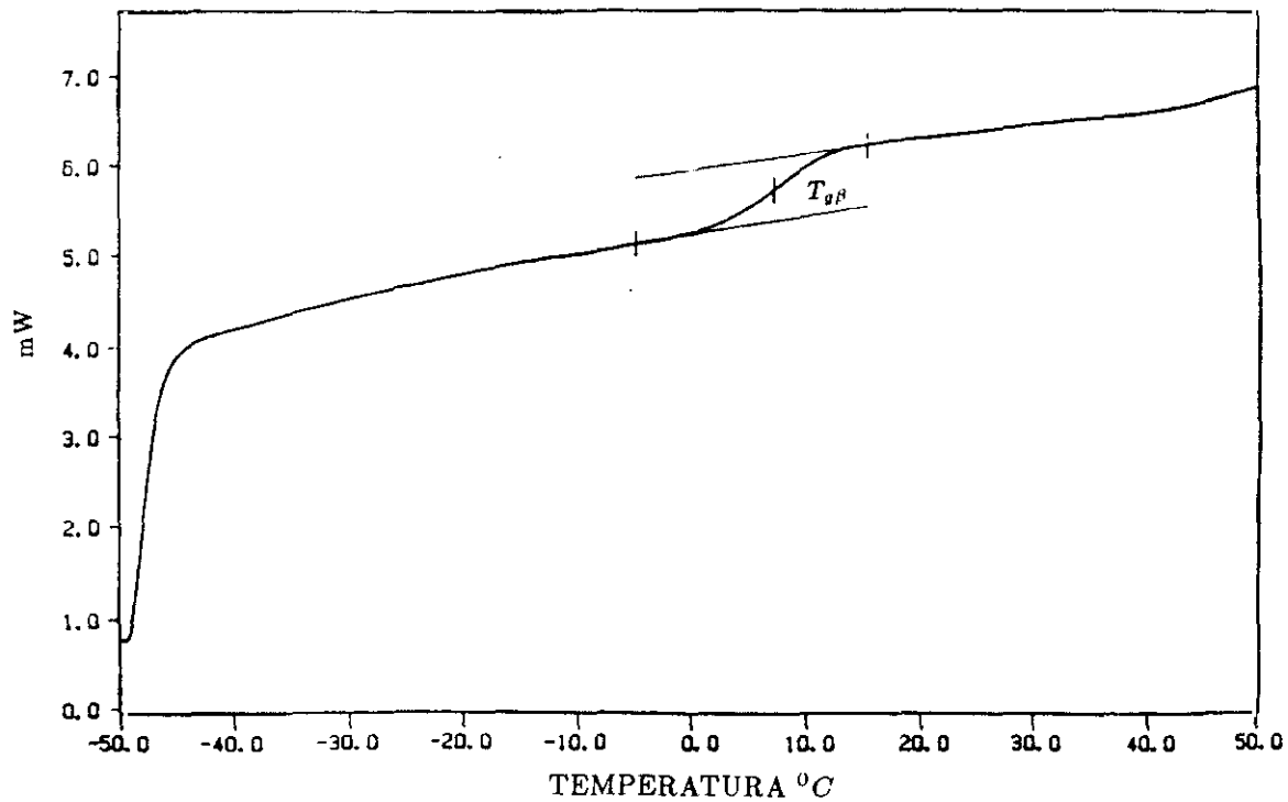
Figura 23: Temperatura de transición vítrea ( \beta ) del preimpregnado para el MATERIAL 1 obtenida por D.S.C. a una velocidad de calentamiento de 20^{\circ}\text{C}/\text{min}
