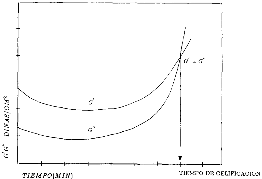
Figura 6: Curva típica obtenida para la determinación del tiempo de gelificación
