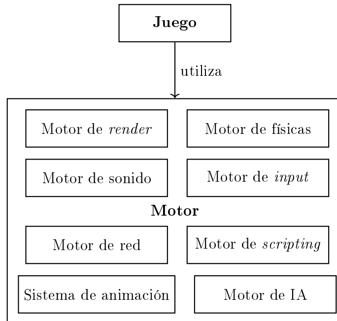
Figura 3.4: Representación esquemática de la estructura de un juego y su motor con algunos de los componentes principales
