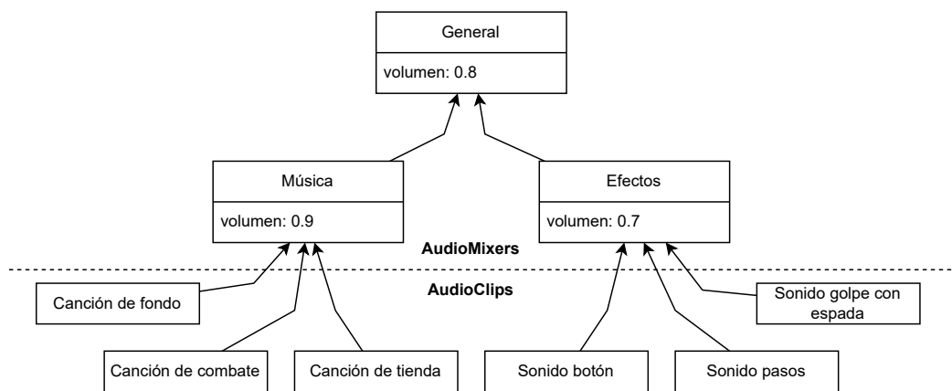
Figura 5.3: Representación de un ejemplo de las conexiones de los elementos del sistema de audio del motor.
