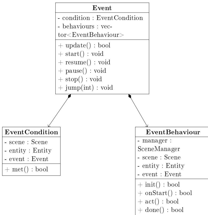
Figura 5.4: Esquema de la estructura de un evento del motor.
