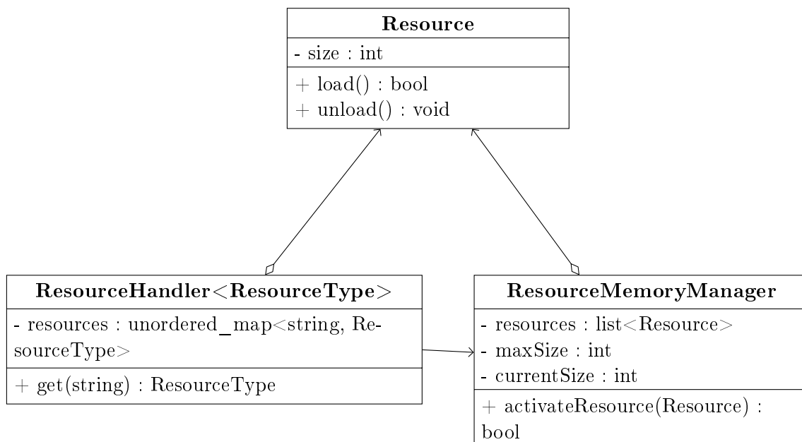
Figura 5.2: Esquema de la estructura del sistema de gestión de recursos del motor.
