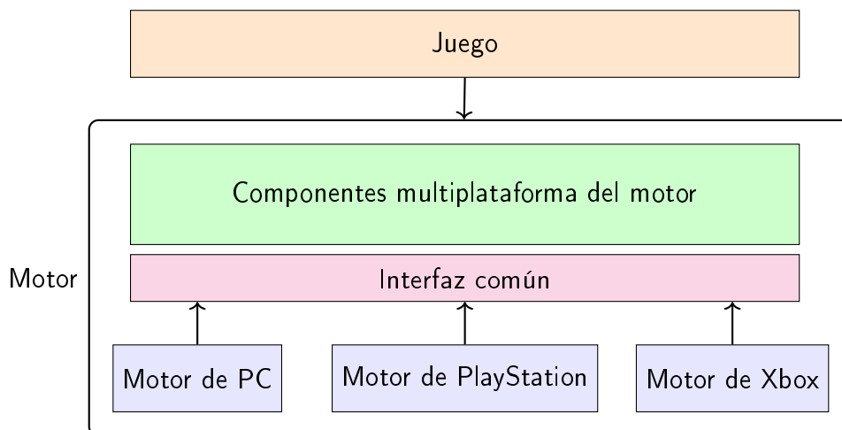
Figura 3.6: Representación esquemática de la arquitectura de un motor multiplataforma
