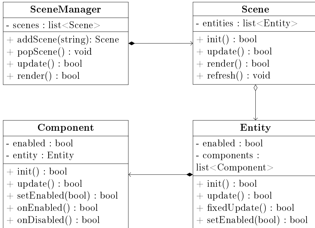
Figura 5.1: Esquema de la estructura del sistema de entidad componente del motor.
