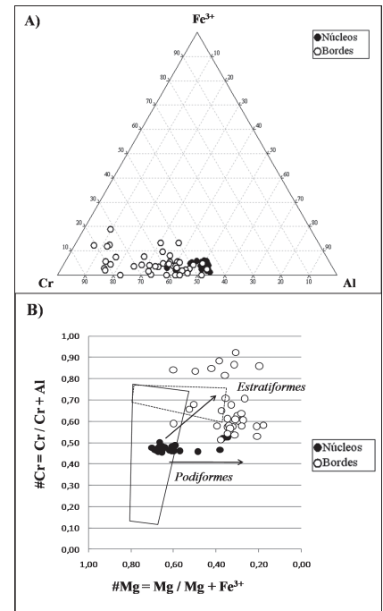
Fig. 2.- A) Composición química de los núcleos y bordes de grano de cromitas de cromititas en un diagrama Cr- \text{Fe}^{3+} -Al; B) Representación de la composición de núcleos y bordes de cromita de cromititas en diagrama \# \text{Mg} - \# \text{Cr} .
