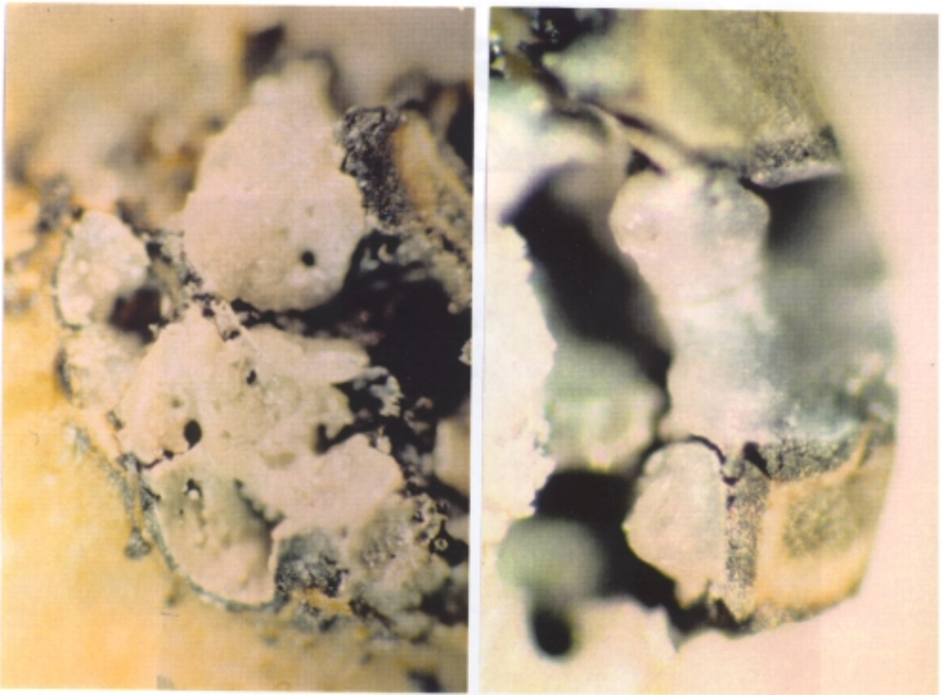
Figura n° 44: Areas de cristalización fusionadas. (x 20). Bisel apical tras interacción láser a 10 W de potencia.
