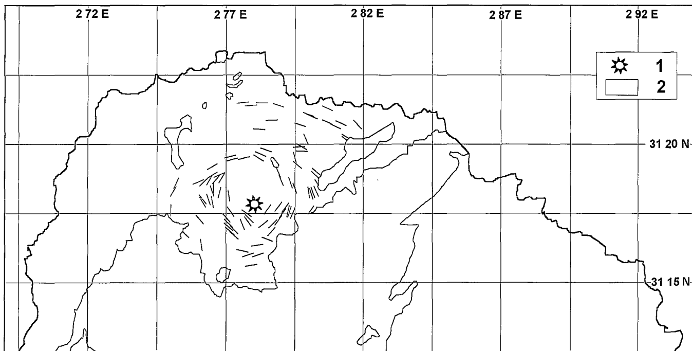
Figura 1: a) Distribución de los diques del enjambre cónico (sólo se han señalado los utilizados en los cálculos): 1: Posición del centro de convergencia calculado. 2: Series volcánicas posteriores al enjambre. b) Rosa de distribución de los sentidos de buzamiento.
