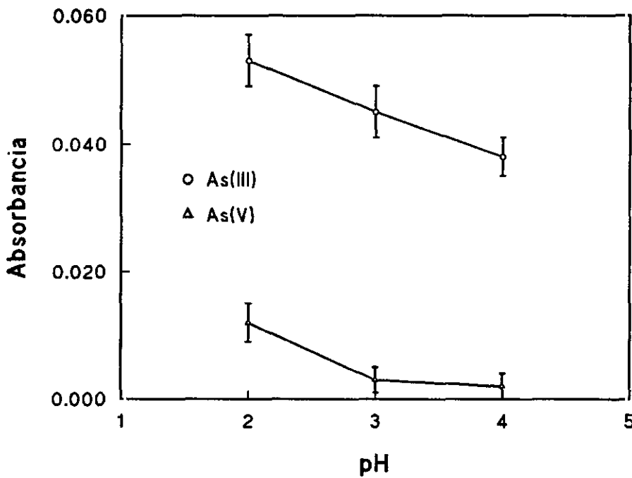
Figura V. 31.- Variación de la absorbancia obtenida para el hidruro de arsénico a partir de As(III) y As(V), en medio cítrico/citrato de distintos pH, mediante un sistema de inyección en flujo. (60 \mu\text{g l}^{-1} ).
