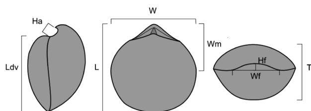
Figure 3. Main biometric parameters measured on Liospiriferina specimens from Almonacid de la Cuba and Ariño localities: L: total length; W: width; T: thickness; Ldv: length of the dorsal valve; Wm: length from the apex to the maximum width; Ha: Height of the cardinal area; Hf: height of the dorsal anterior fold; Wf: width of the dorsal anterior fold. 3. ábra. Az Almonacid de la Cuba és az Ariño lelőhelyekről származó Liospiriferina -példányokon mért fontosabb méretek. L: teljes hosszúság; W: szélesség; T: vastagság; Ldv: a dorsális teknő hossza; Wm: a csücsktől a legnagyobb szélességig mért távolság; Ha: a cardinális terület magassága; Hf: a dorsális anterior kiemelkedés magassága; Wf: a dorsális anterior kiemelkedés szélessége
