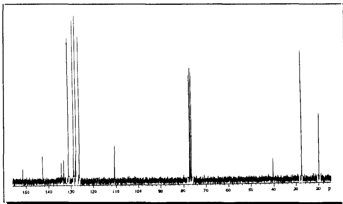
Figura 14. Espectro de ^{13}\text{C} -RMN del compuesto 11d.
