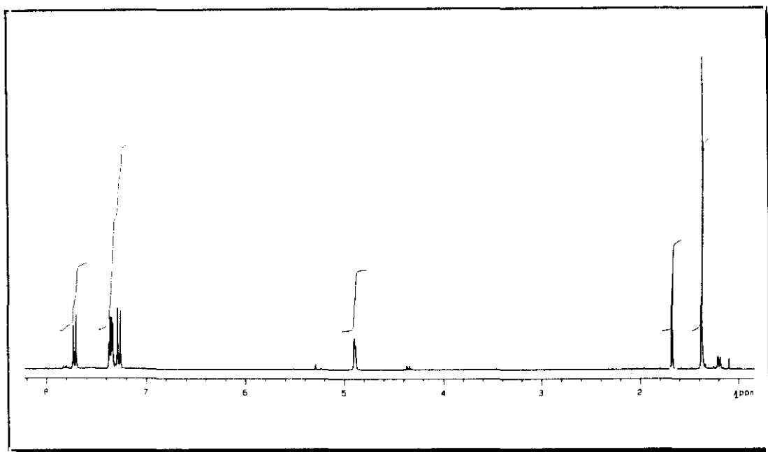
Figura 13. Espectro de ^1\text{H} -RMN del compuesto 11d.
