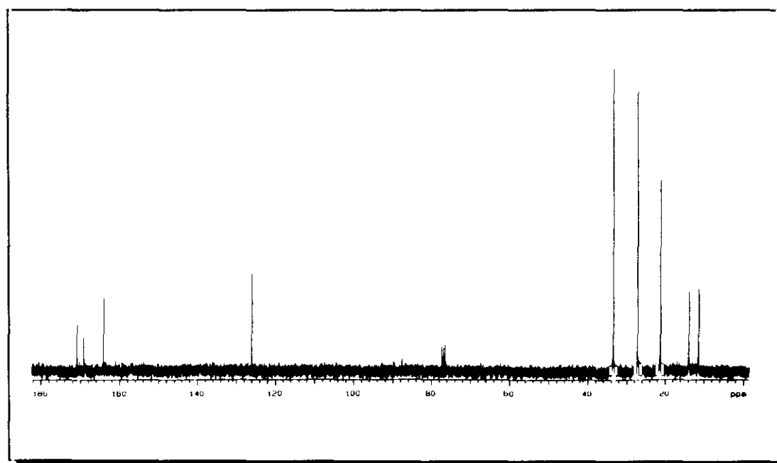
Figura 37. Espectro de ^{13}\text{C} -RMN del compuesto 6d.
