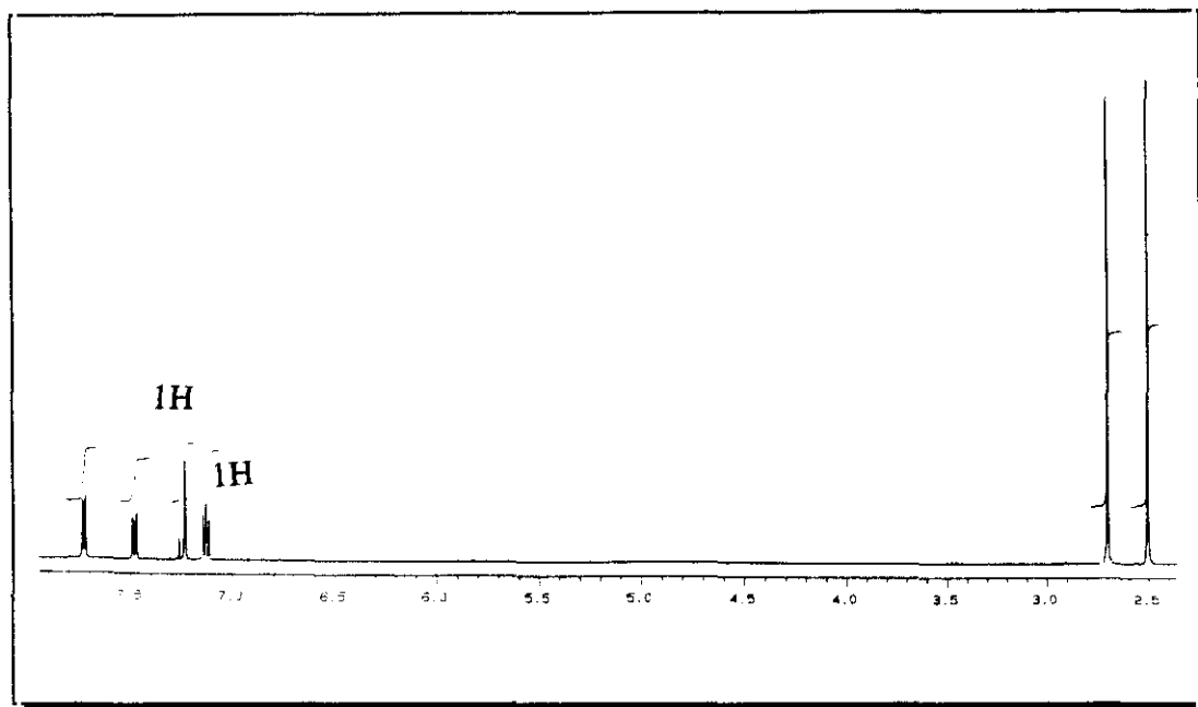
Figura 30. Espectro de ^1\text{H} -RMN del compuesto 4b.
