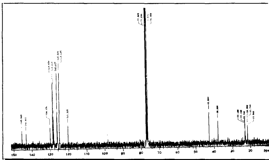
Figura 6. Espectro de ^{13}\text{C} -RMN del compuesto 11a en \text{CDCl}_3 .
