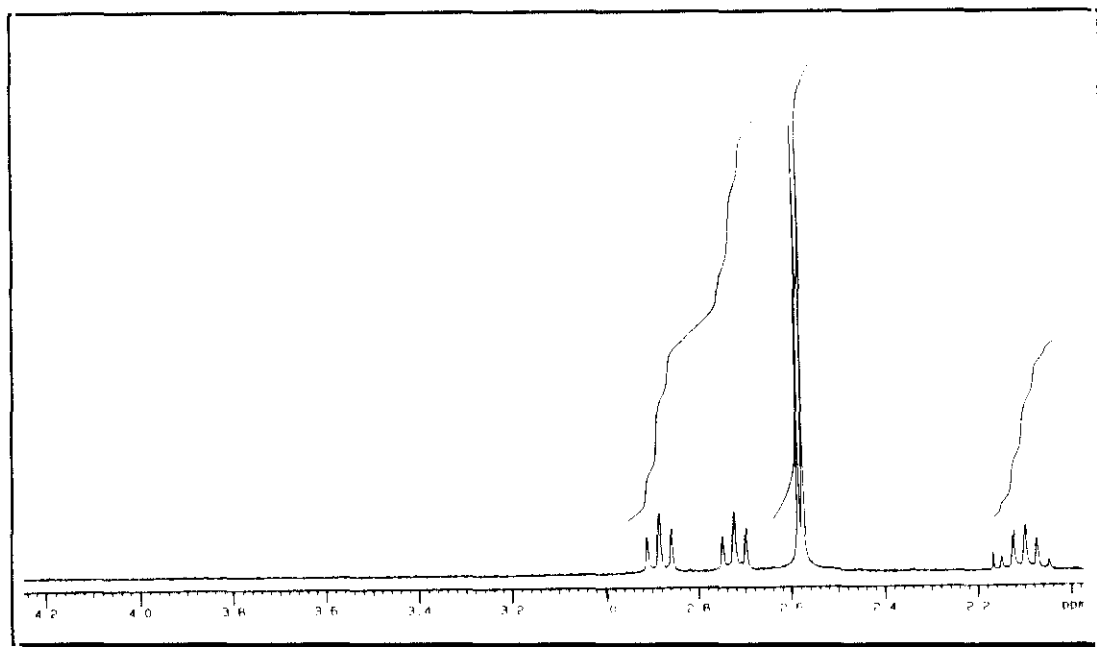
Figura 36. Espectro de ^1\text{H} -RMN del compuesto 6d.
