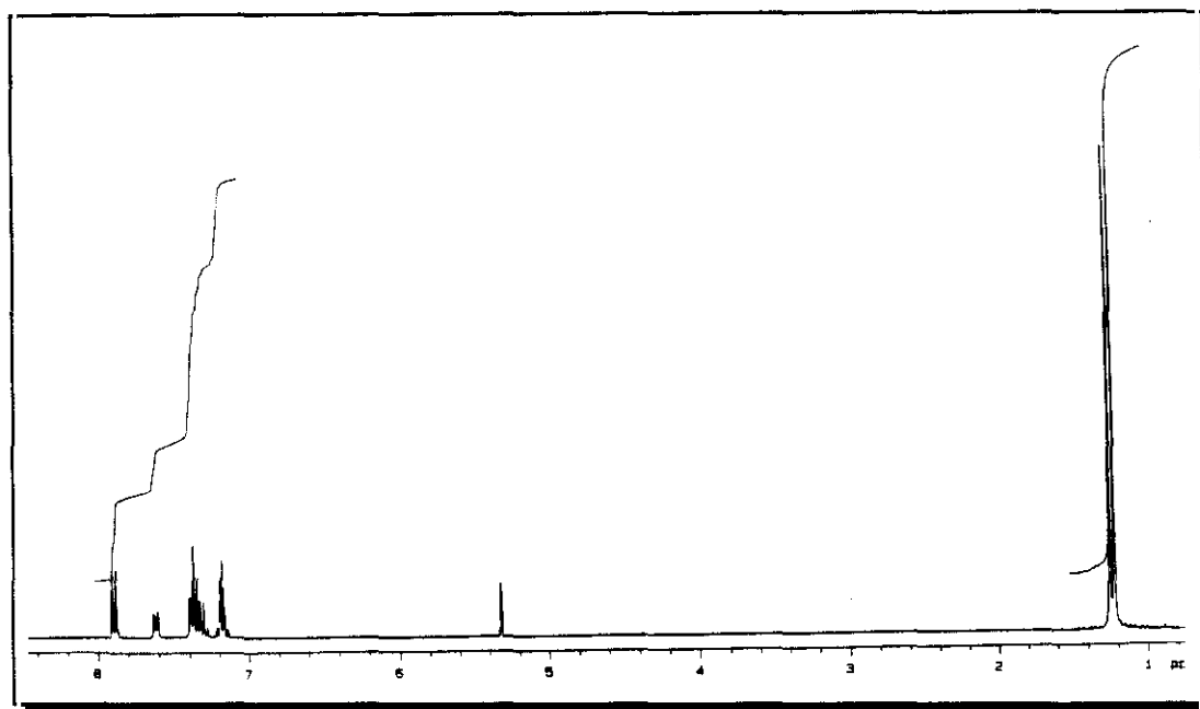
Figura 5. Espectro de ^1\text{H} -RMN del compuesto 11a en \text{CD}_2\text{Cl}_2 .
