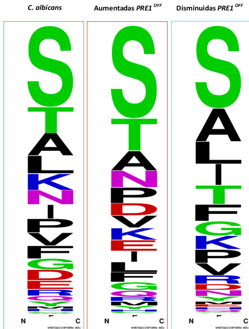
Figura 51. Representación gráfica de la frecuencia de aa en 2 a posición del N-terminoma en C. albicans .
