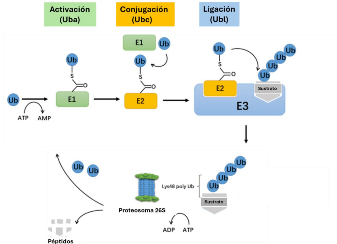
Figura 6. Ruta de ubiquitinación.
