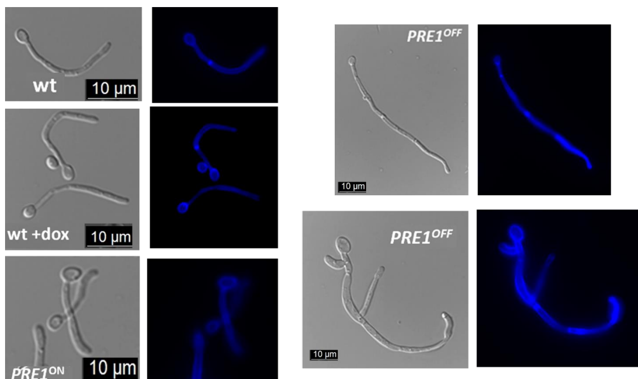
Figura 39. Microscopía de fluorescencia de las células teñidas con blanco de calcoflúor.
