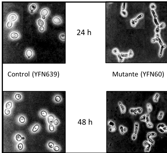
Figura 42. Morfología celular de la cepa candidizada .
