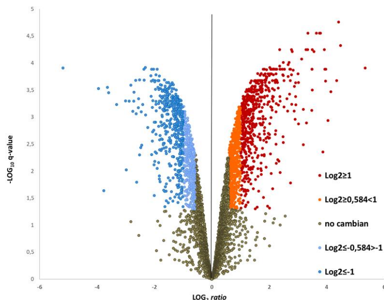
Figura 34. Ratios de la abundancia de proteínas PRE1^{OFF}/PRE1^{ON} .
