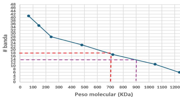
Figura 31. Localización de los complejos del proteosoma 20S y 19S en el gel nativo.
