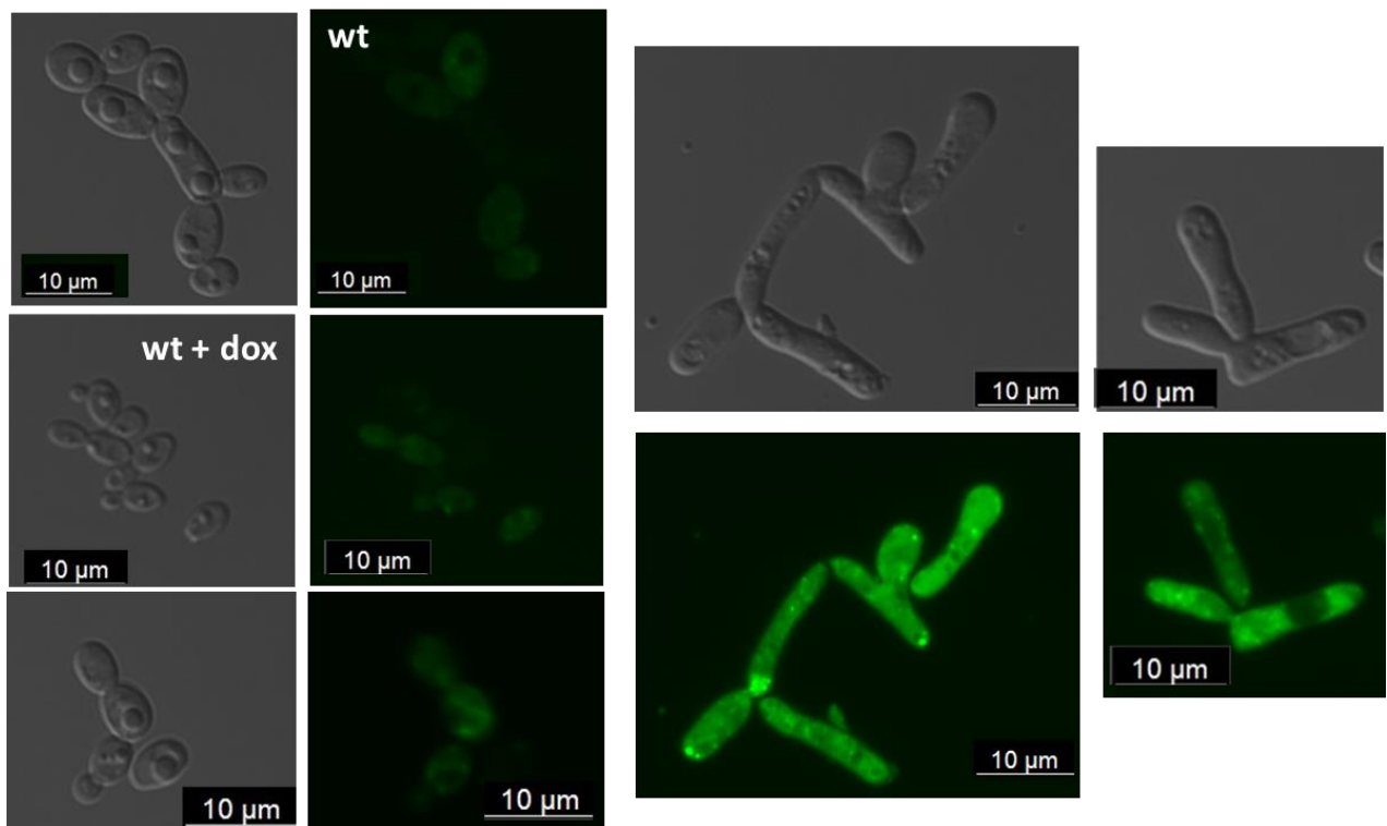
Figura 40. Microscopía de fluorescencia de las células teñidas con DHR123.
