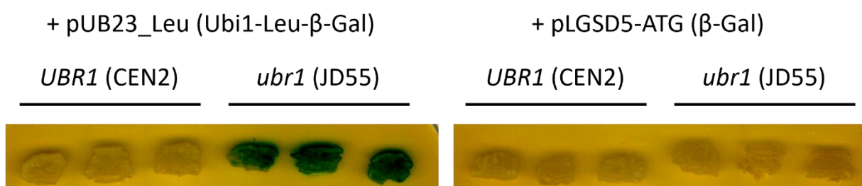
Figura 46. Estudio del fenotipo de la cepa ubr1 \Delta de S. cerevisiae en medio sólido.
