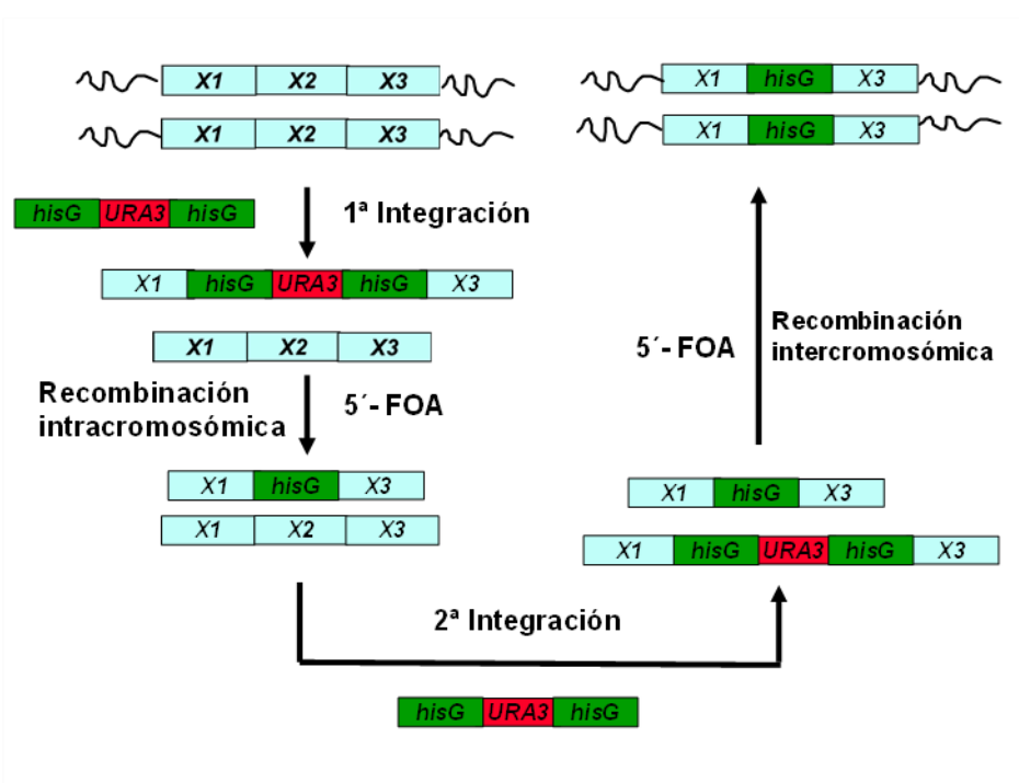
Figura 10. Estrategia de interrupción o delección de genes en C. albicans .
