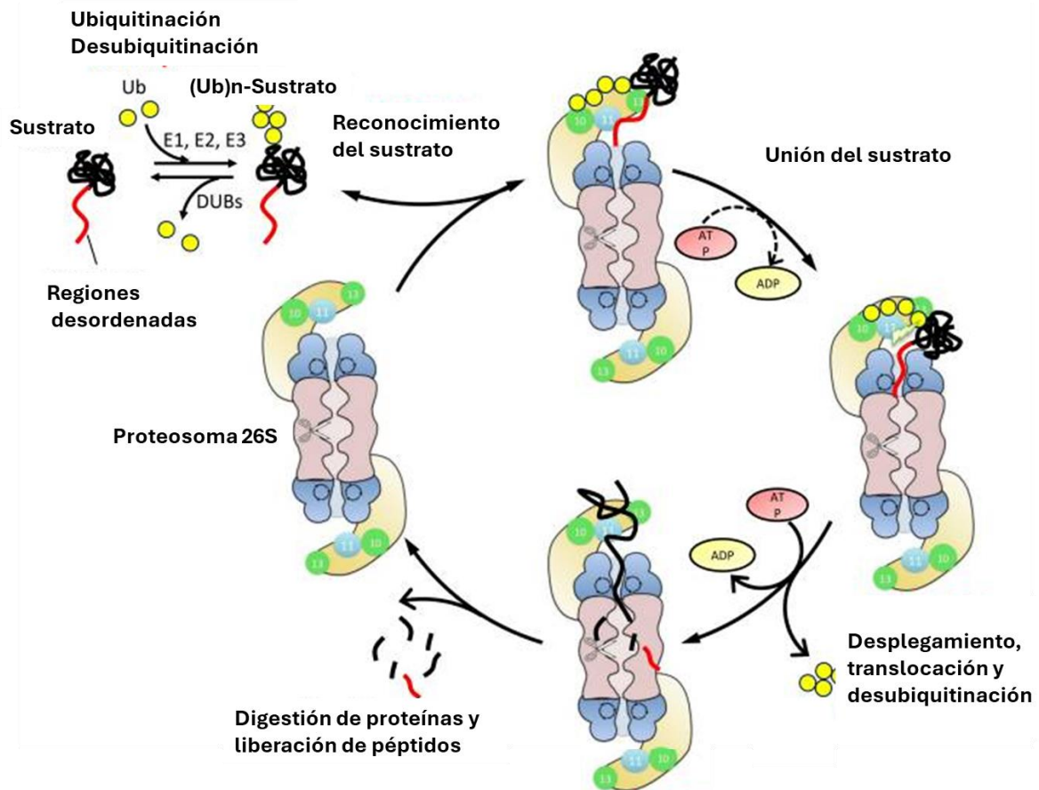
Figura 5. Mecanismo de acción del proteosoma 26S.
