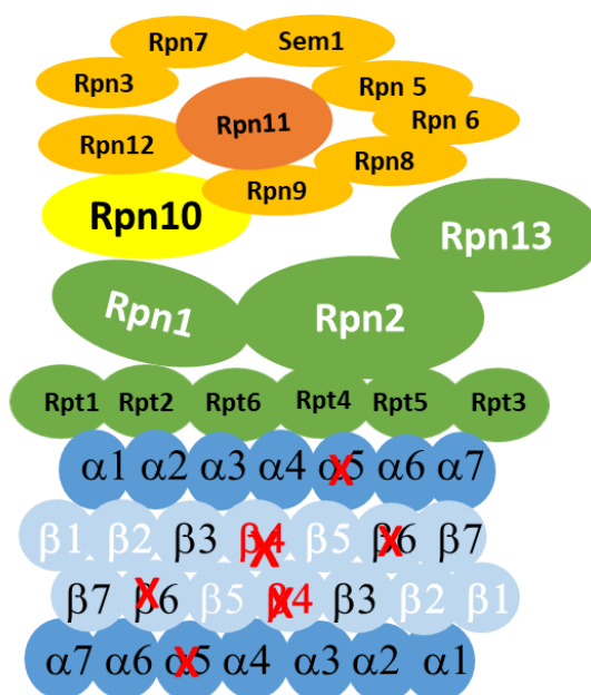
Figura 54. Cambios observados en el ensamblaje de las subunidades del proteosoma 19 S y 20S.
