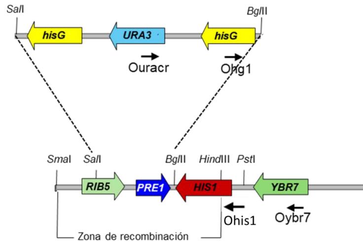
Figura 11. Construcción de delección del gen PRE1 en C. albicans .
