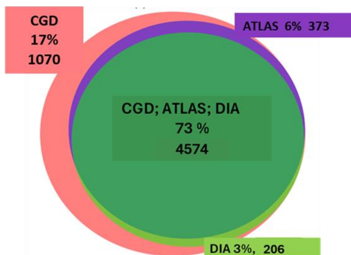
Figura 55. Diagrama de Venn comparativo de proteínas identificadas
