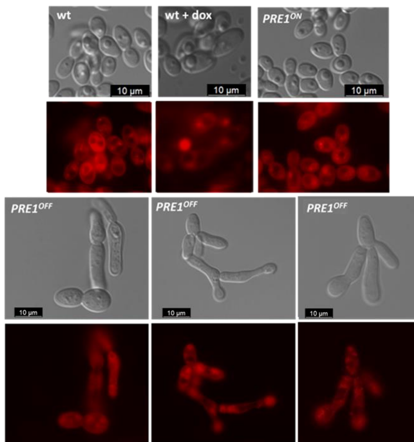
Figura 41. Microscopía de fluorescencia de las células teñidas con el fluorocromo FM4-64.
