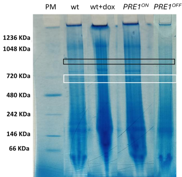
Figura 30. Separación de complejos proteicos mediante electrofóresis nativa (BN-PAGE).
