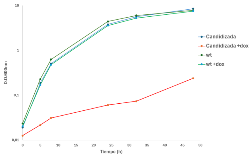
Figura 43. Curva de crecimiento de la cepa candidizada en condiciones de inducción/represión.
