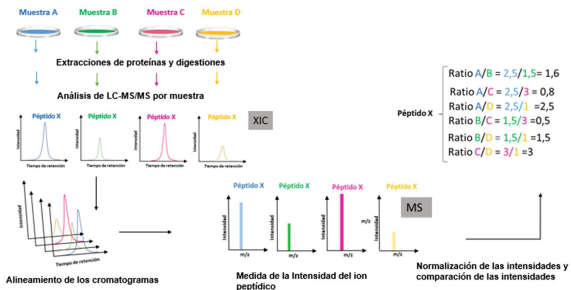
Figura 8. Estrategia de cuantificación proteómica sin marcaje ( label-free ).
