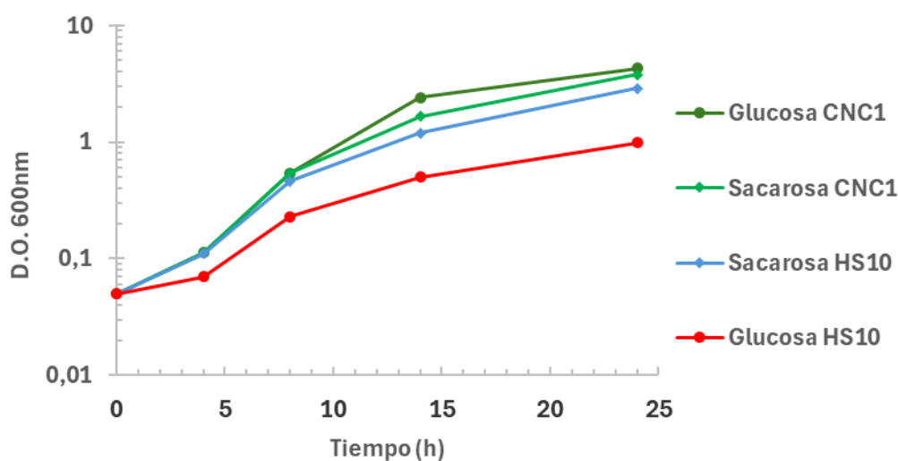
Figura 22. Capacidad de crecimiento del mutante condicional HS10.
