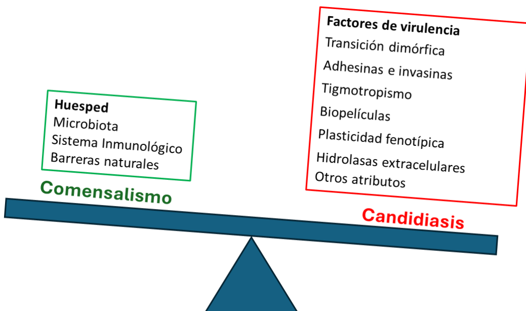
Figura 1. Factores causantes del paso de C. albicans de comensal a patógeno.
