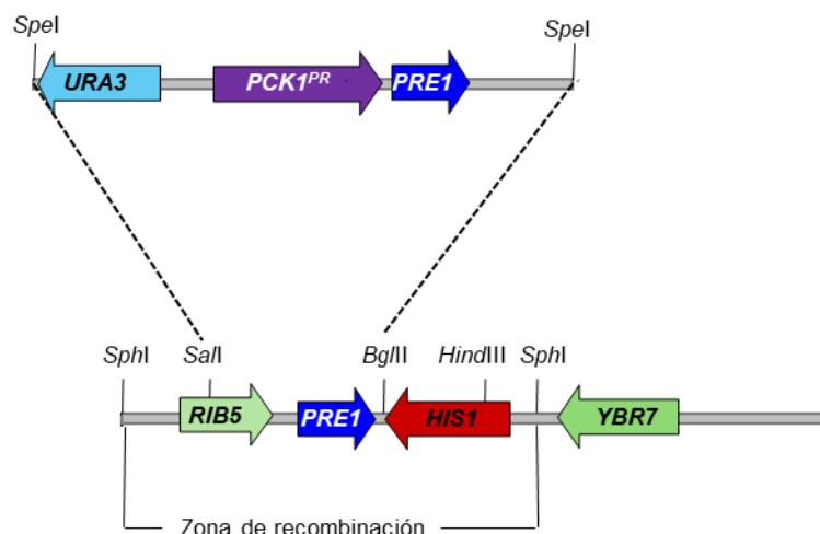
Figura 14. Estrategia de obtención del mutante condicional en CaPRE1 de C. albicans .
