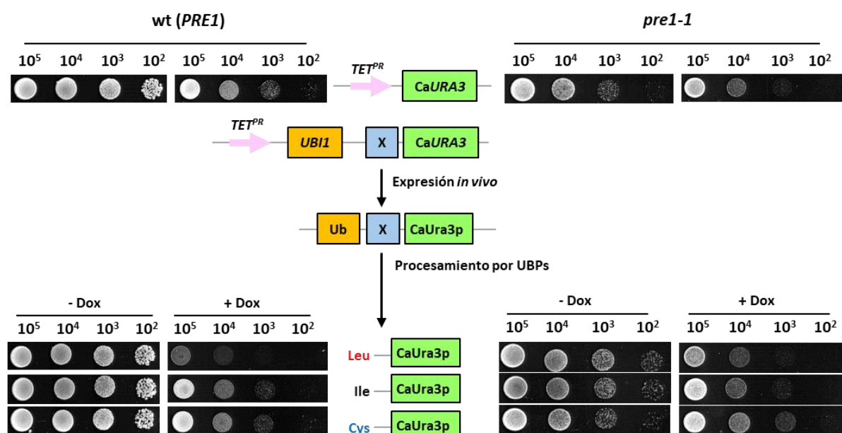
Figura 50. Crecimiento en medio sólido de variantes de CaUra3p en mutantes en proteosoma.
