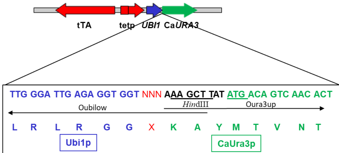
Figura 15. Detalle de la construcción de las fusiones UBI1-X-CaURA3 .
