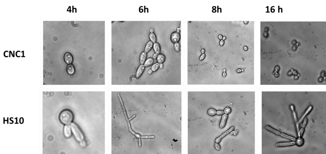
Figura 23. Morfología celular del mutante condicional PRE1 en condiciones de represión.
