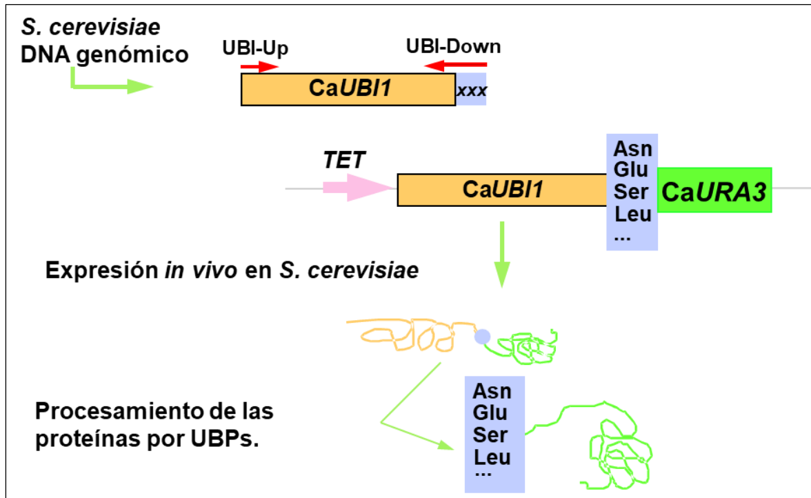
Figura 45 Generación de sustratos de la proteólisis según la regla del extremo amino-terminal.
