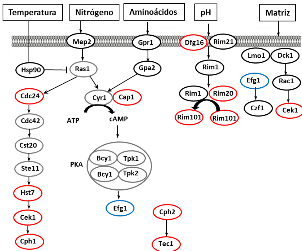
Figura 58. Esquema de diferentes vías de regulación de la filamentación.
