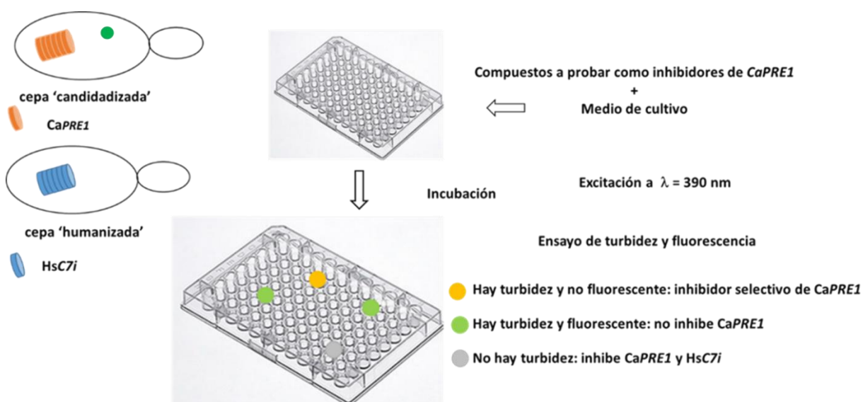
Figura 44. Bioensayo basado en el marcaje diferencial de las cepas humanizada y candidizada .
