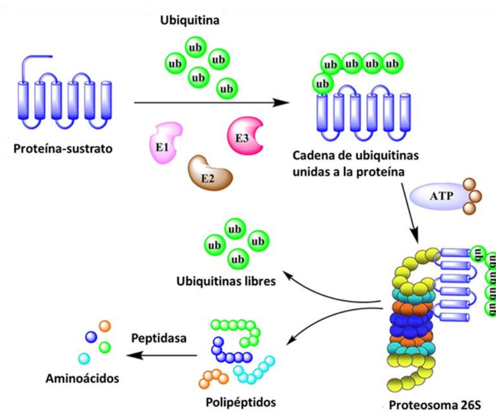
Figura 57. Esquema de la actividad proteolítica del proteosoma.
