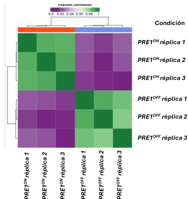
Figura 33. Matriz de correlación de Pearson.
