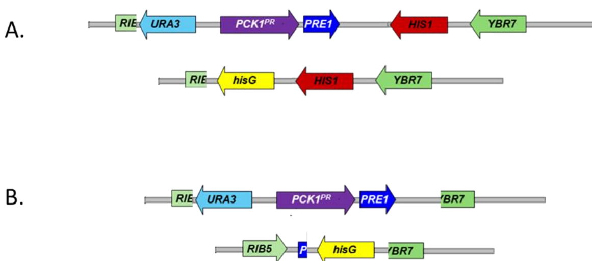
Figura 20 Esquema del genotipo de mutantes condicionales pre1 de C. albicans .
