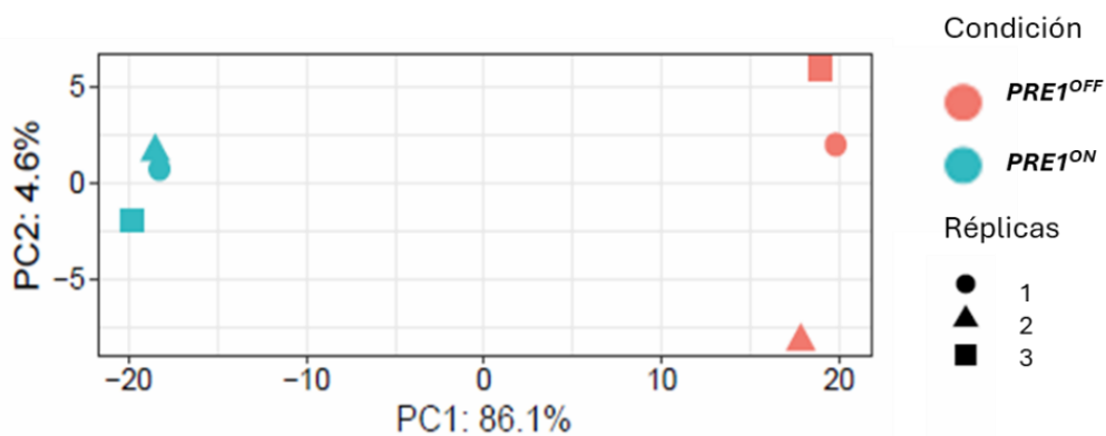
Figura 32. Análisis de componentes principales (PCA).
