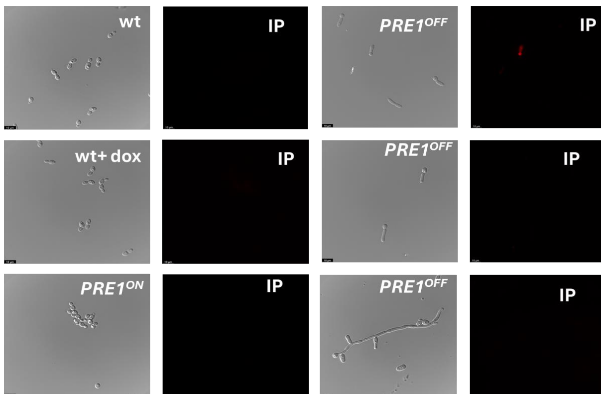
Figura 29. Estudio de viabilidad celular de PRE1 OFF .
