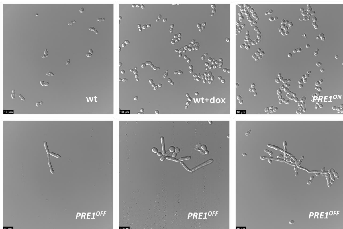
Figura 28. Caracterización morfológica del mutante condicional en condiciones de inducción y represión de CaPRE1.
