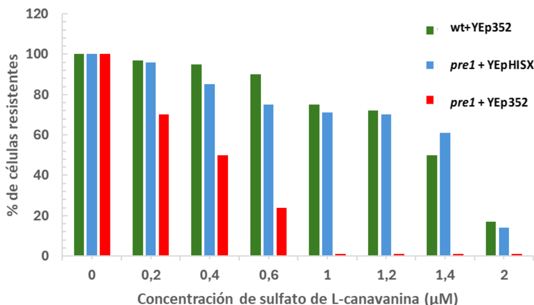
Figura 19. Complementación del fenotipo de sensibilidad a sulfato de L-canavanina del mutante pre1 de S. cerevisiae por el gen CaPRE1 .
