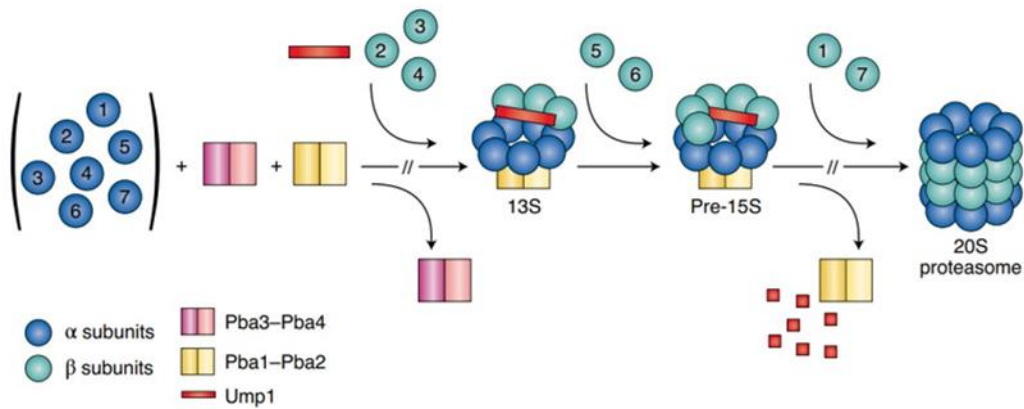
Figura 56. Ensamblaje de la partícula catalítica 20S del proteosoma.
