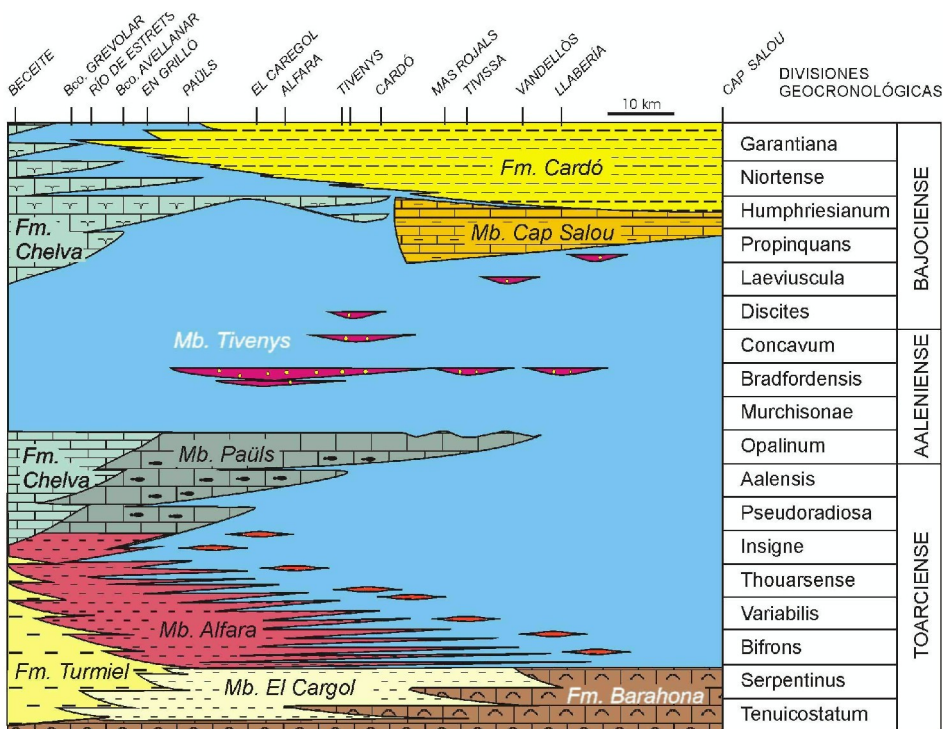
FIG. 4.—Distribución geocronológica de los distintos miembros de la Fm. Sant Blai (según Fernández-López et al., 1998).
