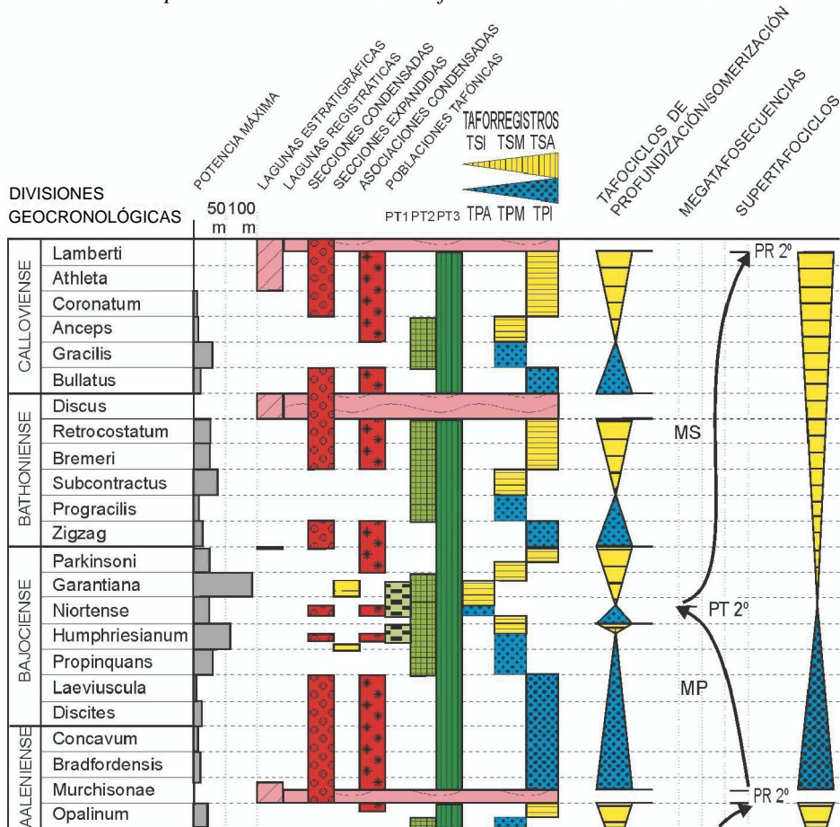
FIG. 8.—Variaciones a escala zonal de la potencia máxima, distribución de lagunas, secciones condensadas o expandidas, asociaciones condensadas, tipos de poblaciones tafónicas y tavorregistros de ammonites, tafociclos de profundización/somerización, megatafosecuencias y supertafociclos identificados en el Jurásico Medio de las plataformas Castellana, Aragonesa y de Tortosa. MS= megatafosecuencia de somerización. PT1= poblaciones tafónicas de tipo 1. PT2= poblaciones tafónicas de tipo 2. PT3= poblaciones tafónicas de tipo 3. TPI= tavorregistro de profundización incipiente. TPM= tavorregistro de profundización media. TPA= tavorregistro de profundización avanzada. TSI= tavorregistro de somerización incipiente. TSM= tavorregistro de somerización media. TSA= tavorregistro de somerización avanzada. PT2° = pico transgresivo de segundo orden. PR2° = pico regresivo de segundo orden (según Fernández-López, 1997b).
