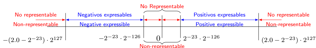
Figura 5.3: Números representables y desbordamientos en el estándar IEEE 754 de precisión simple. Figure 5.3: Representable numbers and over/under-flows in the IEEE 754 simple precision standard.
