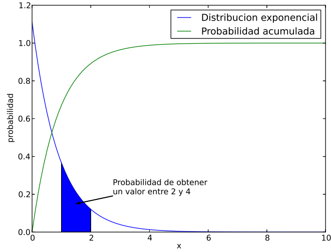
Figura 10.6: Distribución de probabilidad exponencial Figure 10.6: Exponential probability distribution
