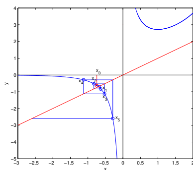
(f) iteracion 5: Raíz de la función
