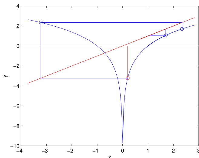
Figura 6.18: primeras iteraciones de la obtención de la raíz de la función f(x) = e^x - x^2 aplicando el método del punto fijo sobre la función g(x) = \ln(x^2) .
