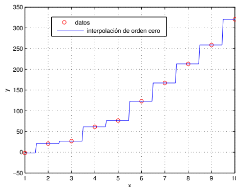
(a) Interpolación de orden cero (a) Zero-order interpolation
