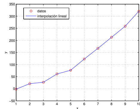
(b) Interpolación lineal (b) Linear interpolation
