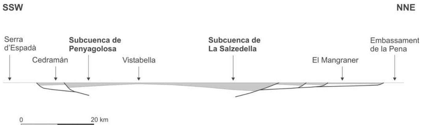
Fig. 2.- Corte estructural sintético de la cuenca del Maestrat restituído a la base de la sucesión postrift albiense superior-senoniense. Ver situación en la Fig. 1.
