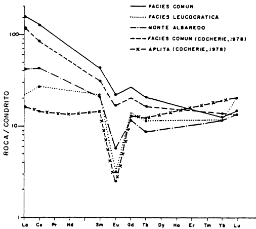
Fig. 4. Diagrama de REE (normalizados a valor condritico) de los granitoides del Macizo de Neira.
