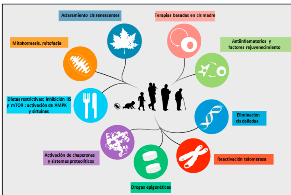
Figura 12. Marcadores moleculares asociados al envejecimiento se agrupan en tres categorías:
