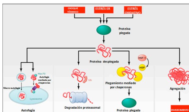
Figura 4. Pérdida de proteostasis. El estrés (endógeno o exógeno) causa el desdoblamiento de proteínas, las cuales pueden ser redobladas por las proteínas de choque térmico (HSP) o
