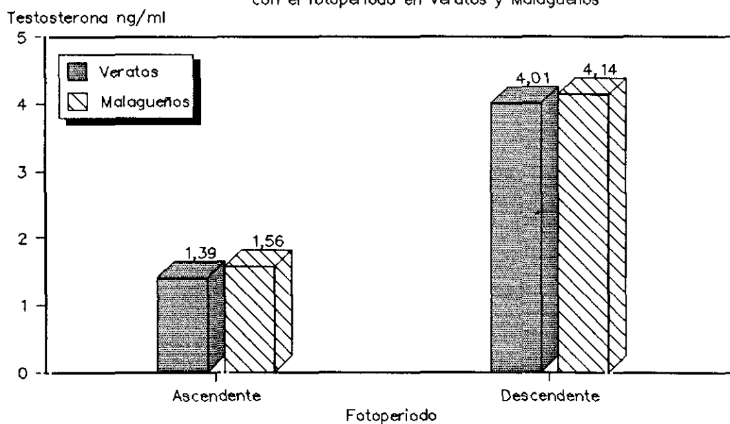
Gráfica 2.4.—Variaciones de la testosterona plasmática con el fotoperíodo en Veratos y Malagueños
