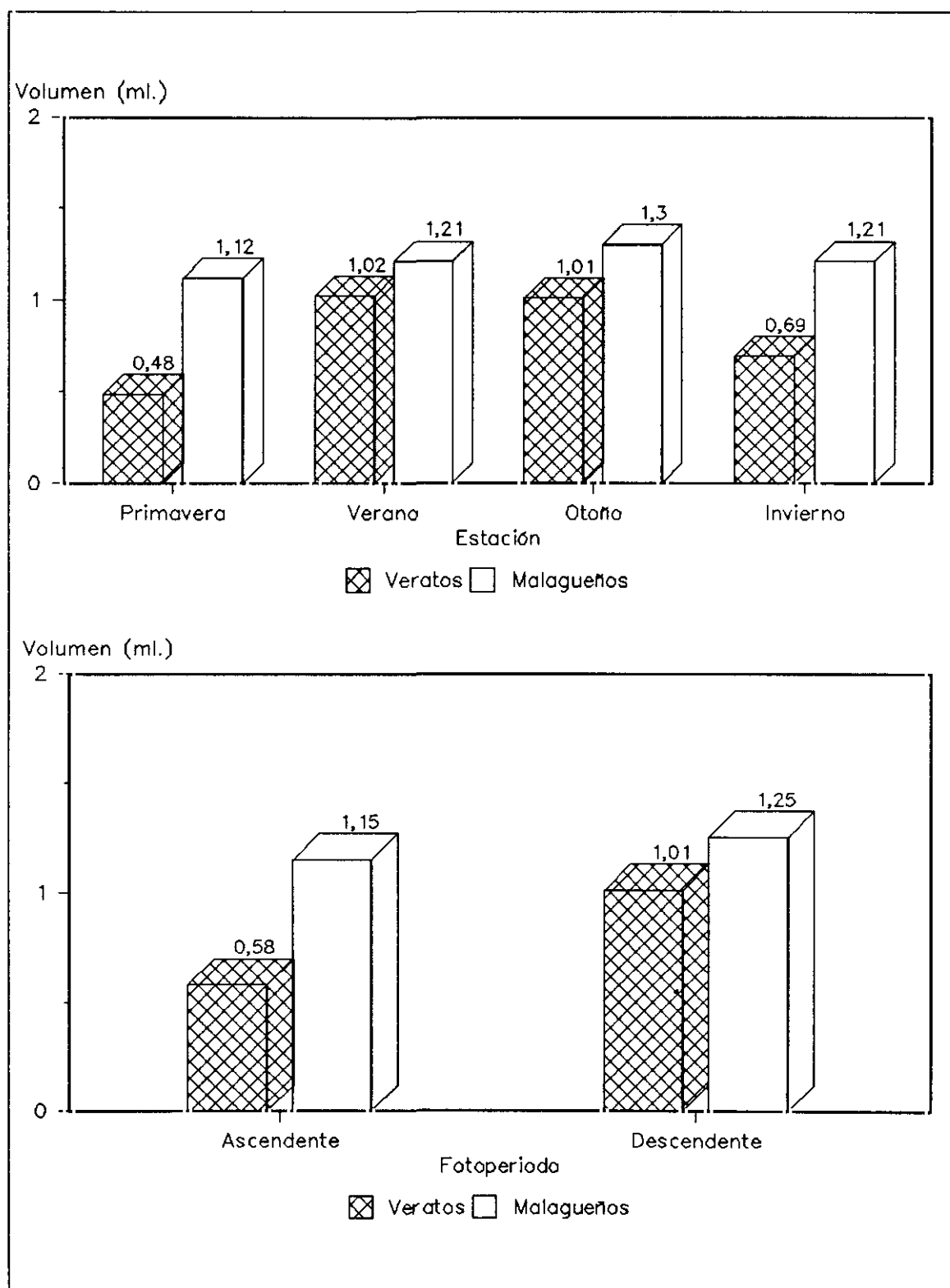
Gráfica 3.4.- Variaciones estacionales y efecto del fotoperíodo sobre el volumen del eyaculado en machos Veratos y Malagueños
