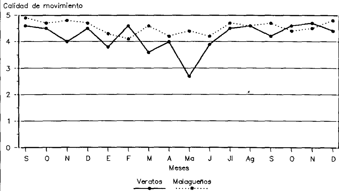
Gráfica 3.8.—Evolución de la calidad de movimiento en machos Veratos y Malagueños desde los 8 a los 23 meses de edad
