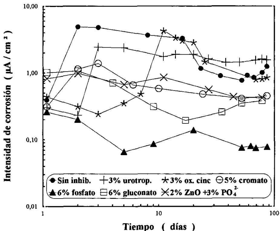
Fig. 54.- Comparación de las respuestas de diferentes inhibidores de corrosión, ensayados en un mortero de relaciones c/a/a=1/3/0,5 , expuesto a atmósferas muy húmedas.
