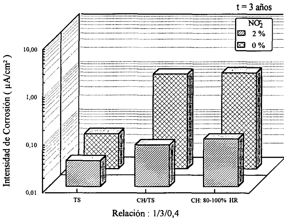
Fig. 44.- En el caso de las probetas fabricadas con agua de mar y arena de playa, las i_{corr} son mayores en ausencia de inhibidor que cuando se utiliza agua de mar y arena normalizada. El nitrito compensa también el efecto desfavorable adicional de los cloruros introducidos con la arena.
