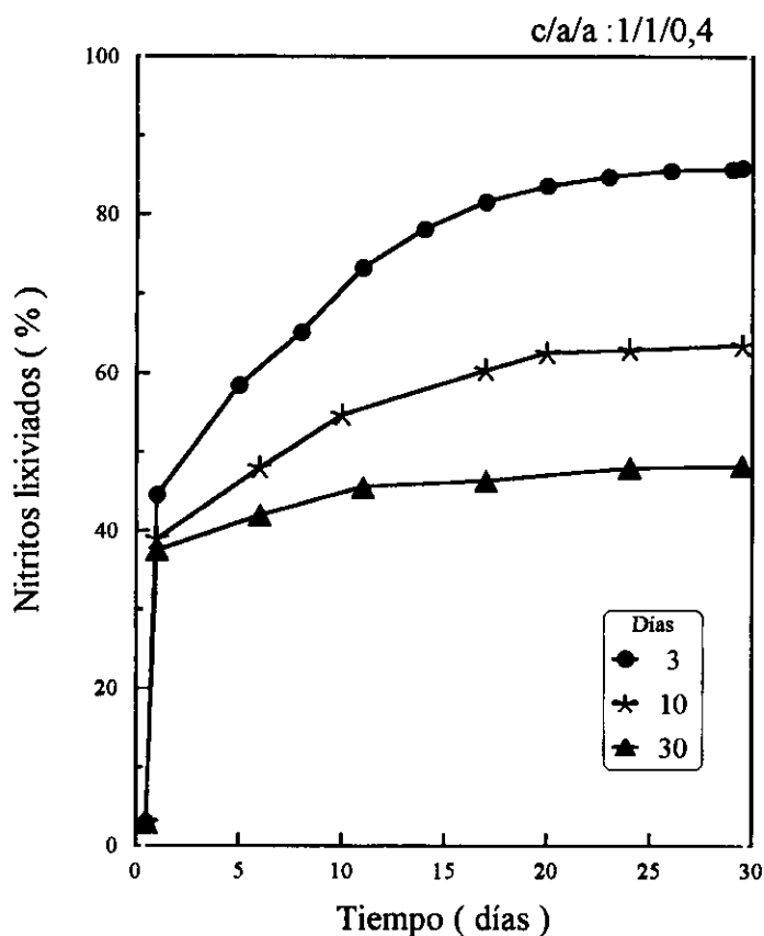
Fig. 29.- Extracción de nitratos por lixiviación en agua de Madrid, con renovación de agua cada 3 y cada 10 días y sin renovación, en el caso de un mortero de relación c/a/a = 1/1/0,4, con un 2% inicial de \text{NO}_2^- . Duración del ensayo 30 días.
