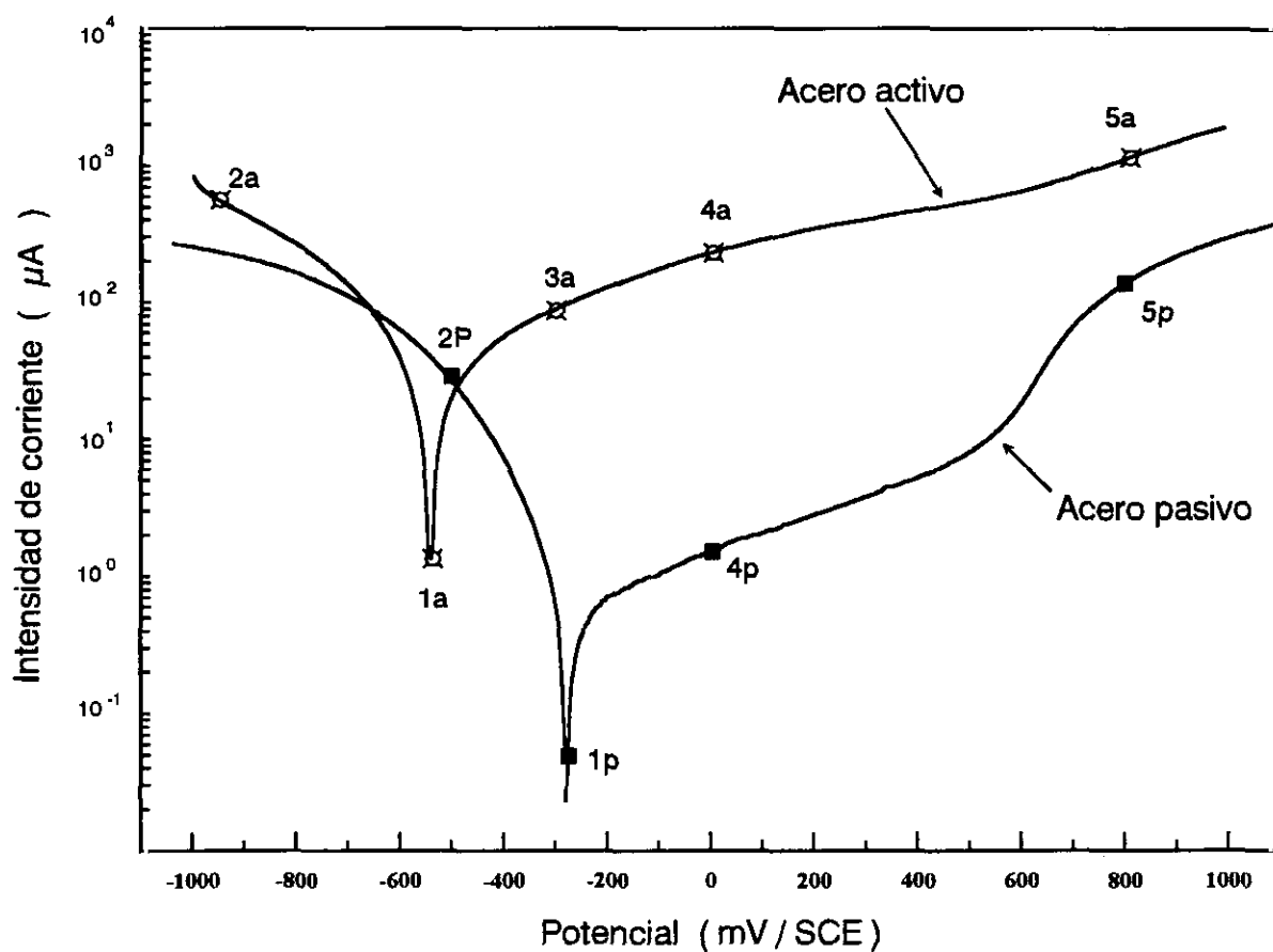
Fig. 68.- Curvas de polarización de acero activo y pasivo, embebidos en morteros con \text{Cl}^- y \text{Cl}^- + \text{NO}_2^- respectivamente. La superficie activa del electrodo de trabajo era de 6\text{cm}^2 .
