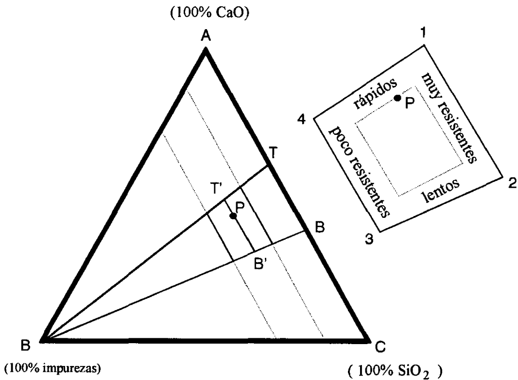
Fig. 2.- Diagrama ternario de composición de los cementos
