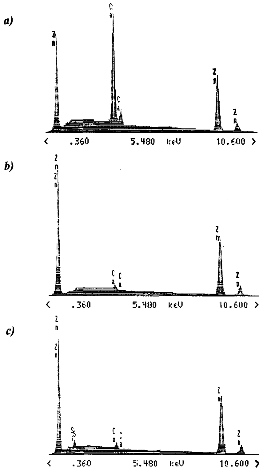
Fig. 96.- Análisis por EDX de los productos de corrosión desarrollados sobre el galvanizado: a) en el centro de una de las placas poligonales de la figura 93b; b) en el producto de corrosión situado entre las placas poligonales de la figura 93c, y c) en los conglomerados aciculares de la figura 94c.
