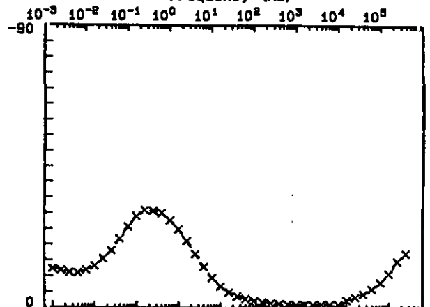
Fig. 114.- Respuestas de un electrodo de acero para armar aislado embebido en hormigón. Puede comprobarse que se obtienen R_t del orden de 10^4 Ohm \cdot cm ^2 , que corresponden a i_{corr} de 2-3 \mu\text{A}/\text{cm}^2 .
