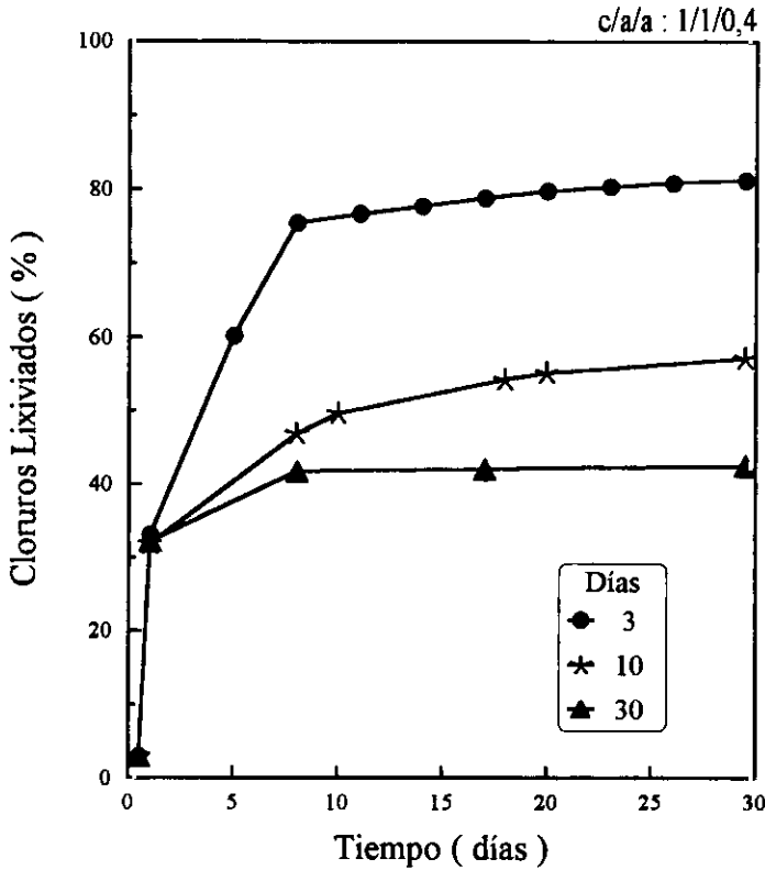
Fig. 32.- Extracción de cloruros por lixiviación en agua de Madrid, con renovación de agua cada 3 y cada 10 días y sin renovación, en el caso de un mortero de relación c/a/a = 1/1/0,4, con un 2% inicial de Ct. Duración del ensayo 30 días.
