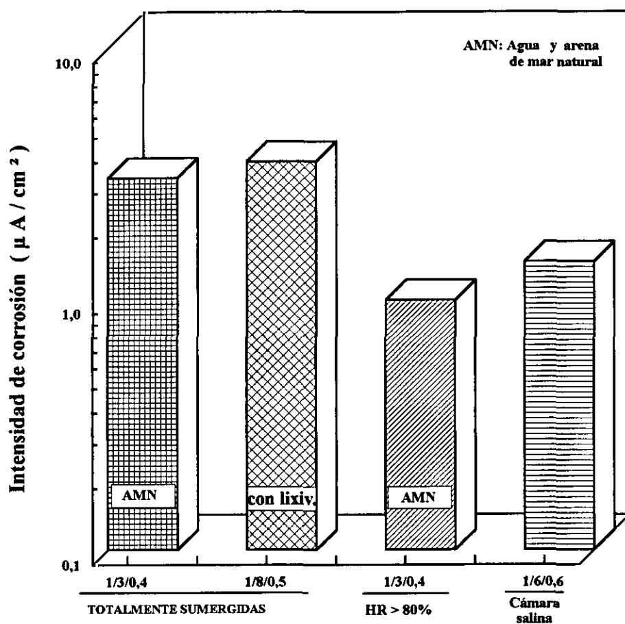
Fig. 53.- Comparación de las i_{corr} a las que se llega, una vez producida la activación, en distintos medios y en morteros con diferentes características
