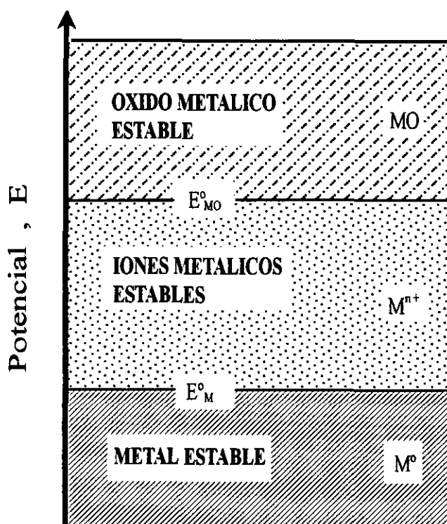
Fig. 102.- Existen potenciales de equilibrio que separan los campos de estabilidad de la forma iónica y del óxido o compuesto pasivante, más elevados que los potenciales que separan los campos de estabilidad de las formas iónica y metálica.
