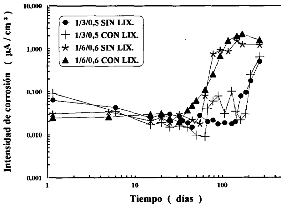
Fig. 52.- La lixiviación previa de los nitritos y la disminución de la relación c/a reducen muy significativamente el periodo de activación durante la exposición en cámara de niebla salina.
