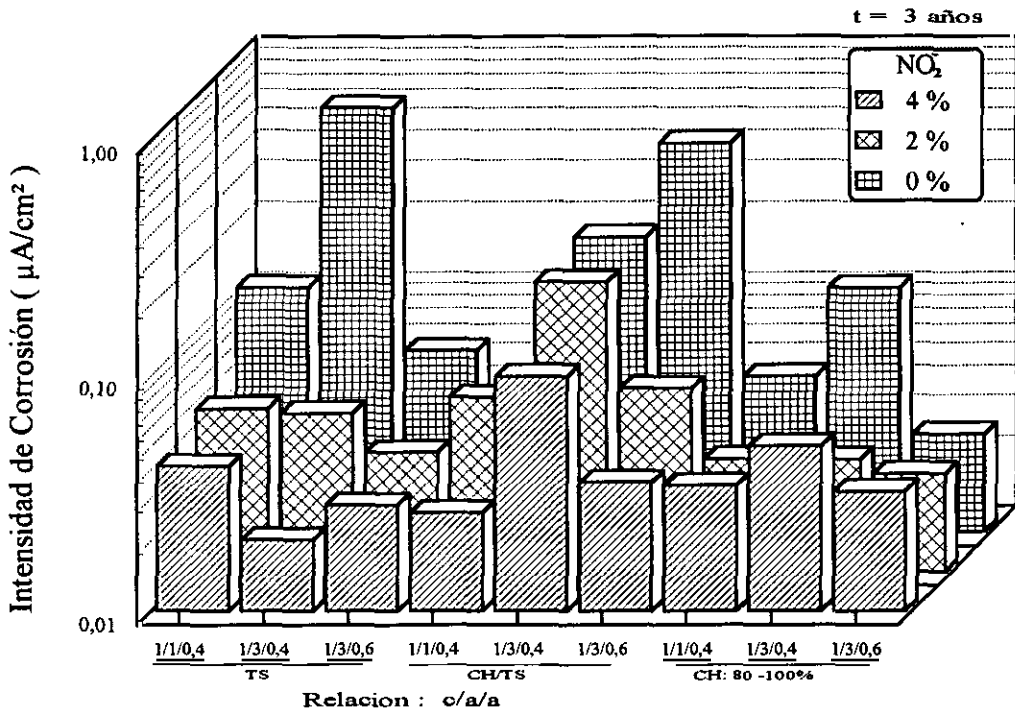
Fig. 43.- Valores de la i_{corr} al término de uno y tres años de exposición, en el caso de morteros amasados con agua de mar y expuestas a una atmósfera del 80 % de HR, en función del contenido en nitrito, y de las relaciones cemento/arena y agua/cemento.
