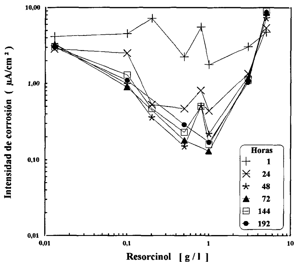
Fig. 36.- Evolución de la i_{corr} con el tiempo para el acero en soluciones saturadas de Ca(OH)_2 , con adiciones de resorcinol.
