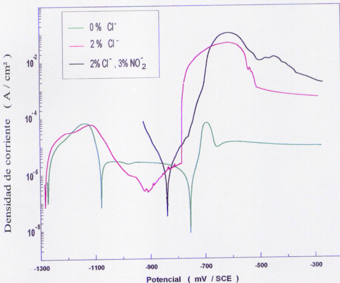
Fig. 87.- Curvas de polarización del acero galvanizado en soluciones saturadas de \text{Ca}(\text{OH})_2 sin aditivos, con un 2% \text{Cl}^- y con 2% \text{Cl}^- + 3% \text{NO}_2^- .
