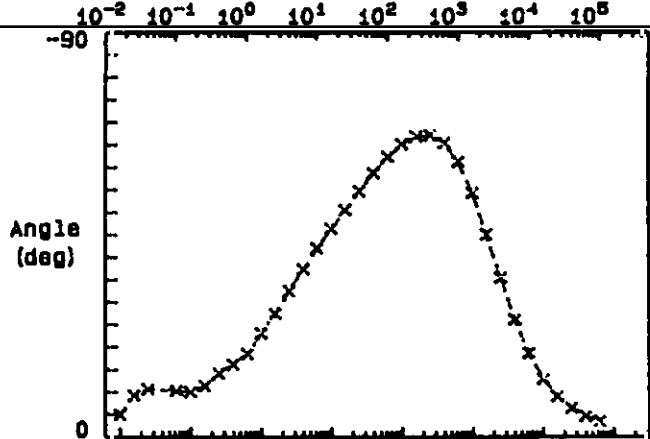
Fig. 81.- Diagramas de impedancia de acero galvanizado sumergido en una solución saturada de \text{Ca(OH)}_2 poco después de la inmersión.
