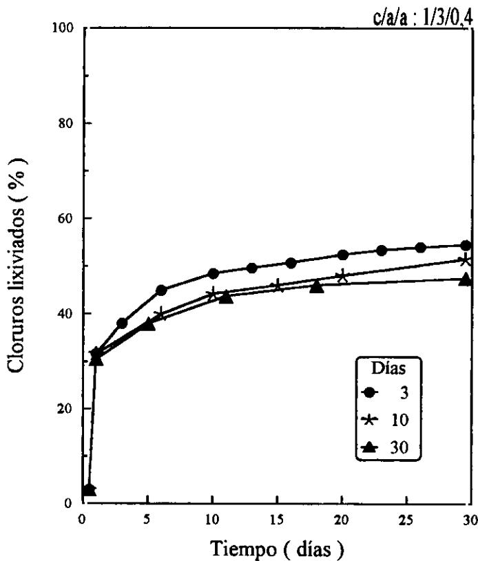
Fig. 33.- Extracción de cloruros por lixiviación en agua de Madrid, con renovación de agua cada 3 y cada 10 días y sin renovación, en el caso de un mortero de relación c/a/a = 1/3/0,4, con un 2% inicial de Ct y 2% de estearato sódico. Duración del ensayo 30 días.
