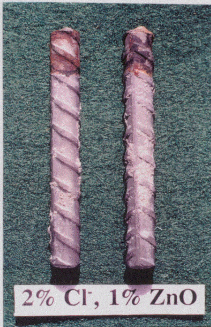
Fig. 62.- Aspecto de los redondos embebidos en un mortero con 2%Cl - + 1% ZnO al término del ensayo. El ZnO ha eliminado la corrosión en las superficies libres, pero no en las ocluidas bajo la resina epoxi, que pretendía enmascarar la soldadura con el alambre de cobre.
