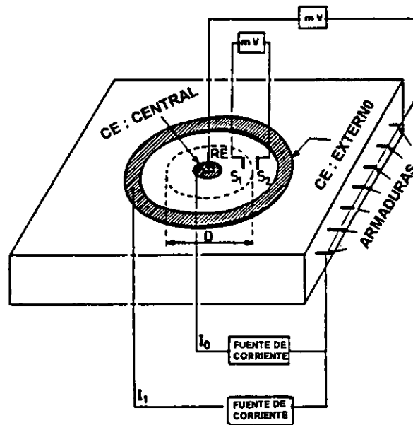
Fig. 124.- Esquema del confinamiento de las líneas de corriente en un área determinada con un anillo de guarda.
