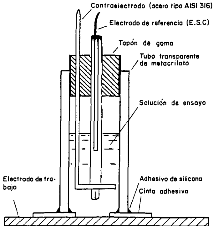
Fig. 20.- Corte transversal de la célula electroquímica utilizada en los ensayos de impedancia.
