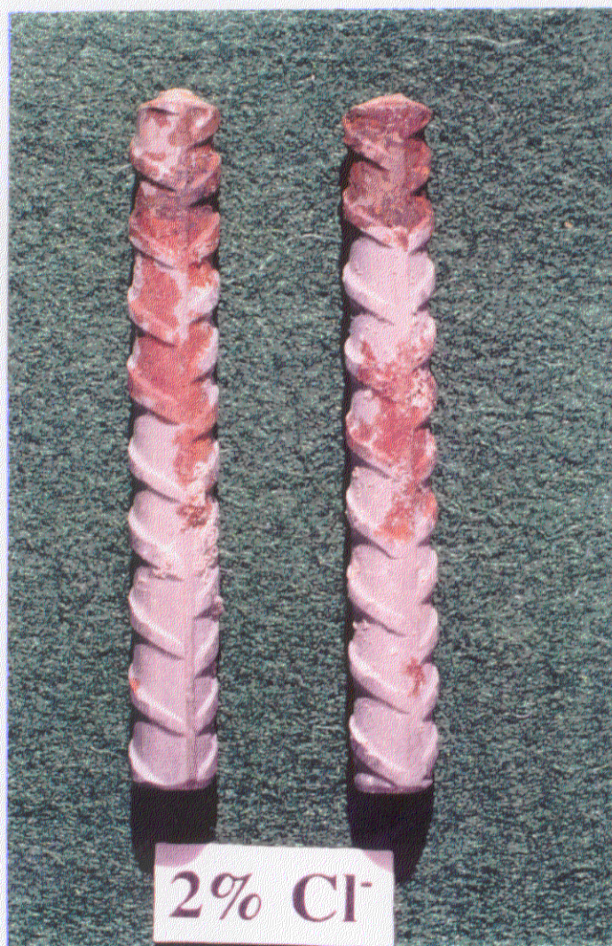
Fig. 58.- Aspecto de los redondos embebidos en un mortero con un 2% de \text{Cl}^- al término del ensayo.
